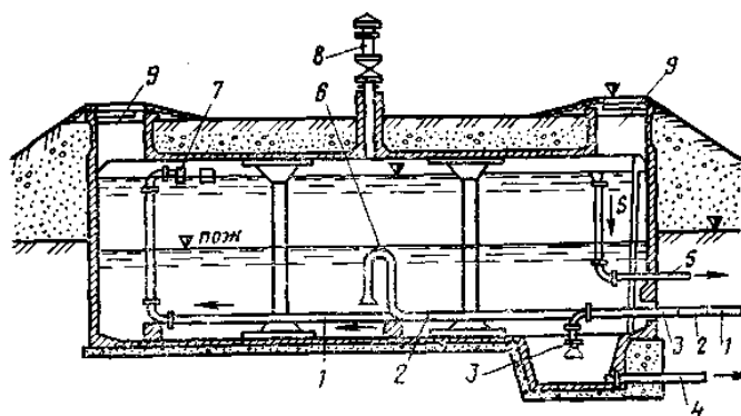
Рис. 4.18. Железобетонный резервуар:
