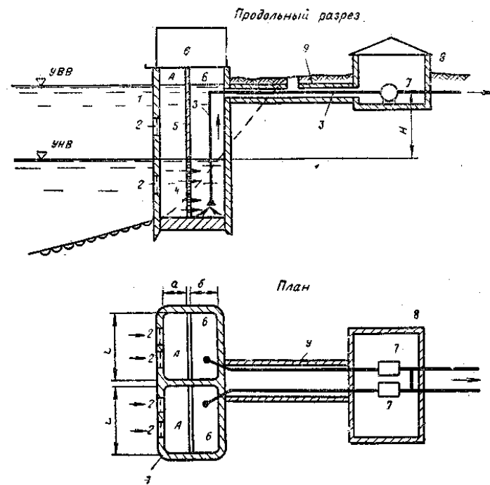
Рис. 3.6. Раздельный водоприемник берегового типа
