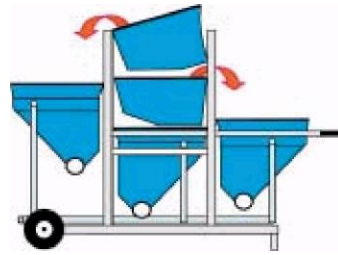
Рис. 8.4. Полуавтоматическое сортировочное устройство SK-I
