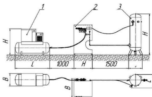
Ри 6.3. Кислородная установка «Провита»: 1 – воздушный компрессор; 2 – генерато кислорода; 3 – ресивер
