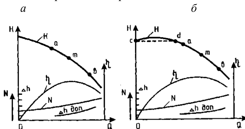
Рис. 4.7. Частные характеристики центробежного насоса: а – стабильная; б – нестабильная
