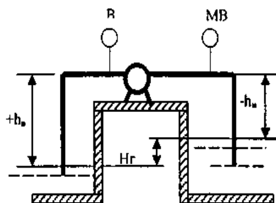
Рис. 4.5. Схема насосной установки с отрицательной высотой нагнетания
