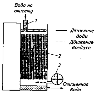
Рис. 5.14. Орошаемый биофильтр: 1 – реактивный ороситель; 2 – загрузка; 3 – воздушный насос
