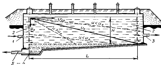
Рис. 5.1. Схема горизонтального отстойника:
