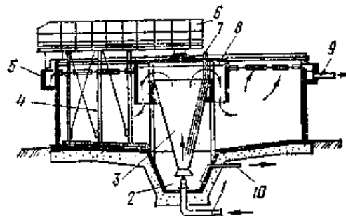
Рис. 5.3. Радиальный отстойник: 1 и 9 – подача исходной и отвод осветленной воды; 2 – приямок для сбора осадка; 3 – диффузор; 4 – вращающаяся ферма для удаления осадка; 5 – сборный кольцевой периферийный лоток; 6 – ходовой мостик; 7 – подача реагентов; 8 – водораспределительный стакан; 10 – сброс осадка
