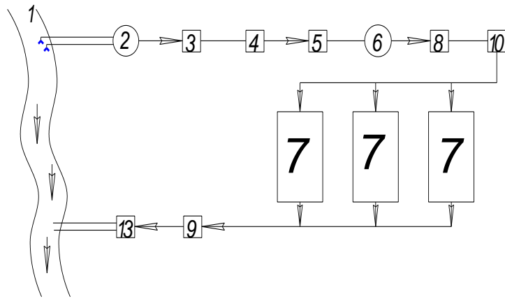
Рис. 3.2. Самотечная прямоточная схема водоснабжения:
