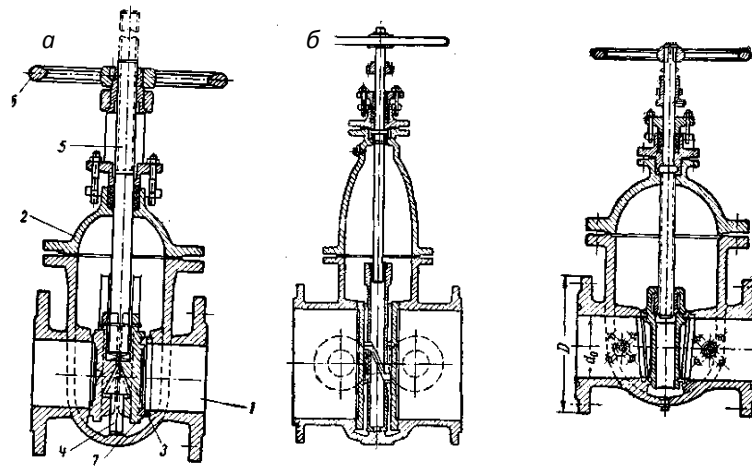
Рис. 4.13. Параллельная задвижка: a – с выдвижным шпинделем; б – с невыдвижным шпинделем
