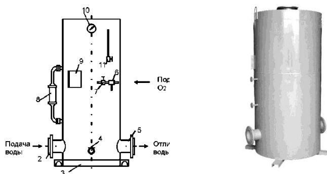
Рис. 6.2. Оксигенатор:
