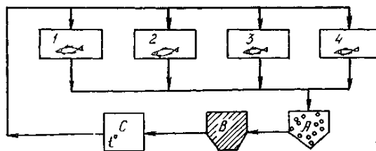
Рис. 5.9. Схема очистки воды с использованием аэротенка:
