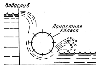
Рис. 6.5. Водослив с лопастным колесом
