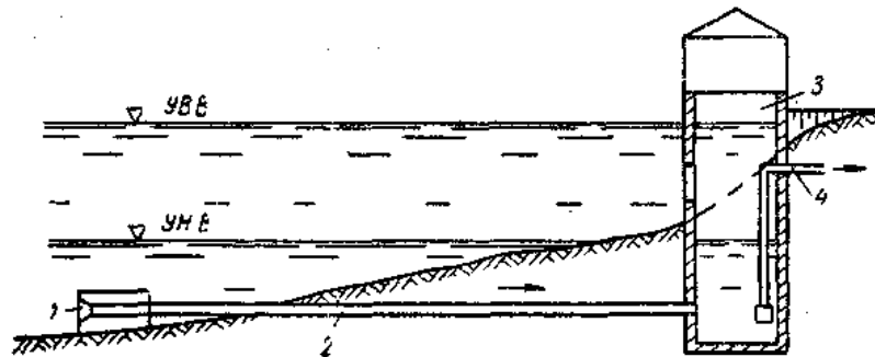
Рис. 3.7. Водоприемник руслового типа:
