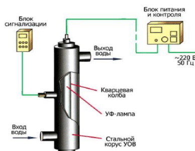
Рис. 5.7. Принципиальная схема ультрафиолетовой установки для обеззараживания воды
