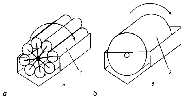
Рис. 5.16. Вращающиеся биофильтры: a – «Штеллерматик»; б – «Евроматик»; 1 – перфорированные трубы, заполненные гофрированными пластиковыми дисками; 2 – сетчатый барабан, заполненный пластиковой загрузкой
