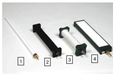
Рис. 6.12. Диффузоры:
