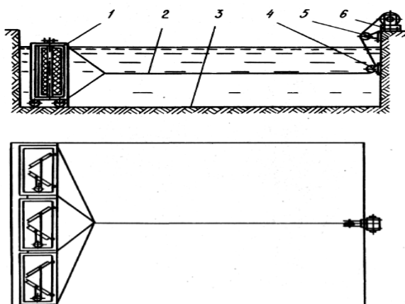
Рис. 8.11. Устройство для разделения форели в выростной емкости: 1 – модуль; 2 – фал; 3 – выростная емкость; 4, 5 – блоки; 6 – грузовая лебедка
