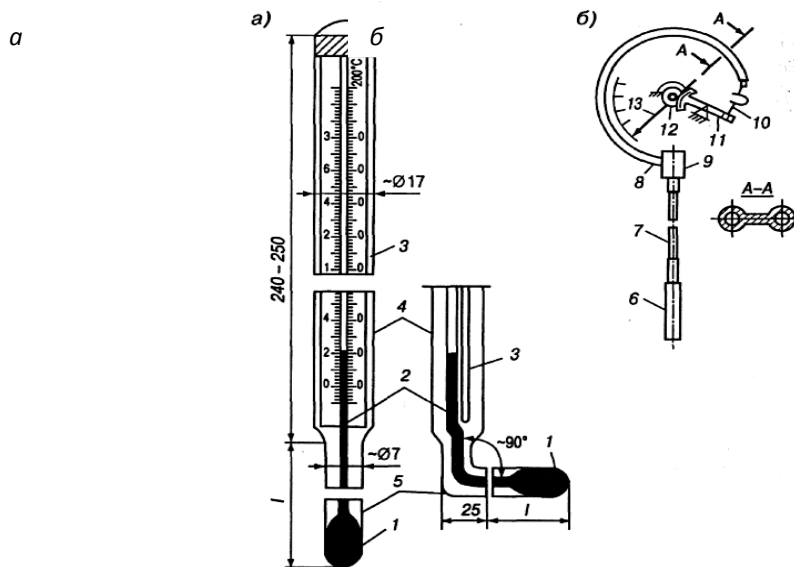
Рис. 5.17. Термометры расширения: а – технический жидкостный стеклянный; б – показывающий манометрический
