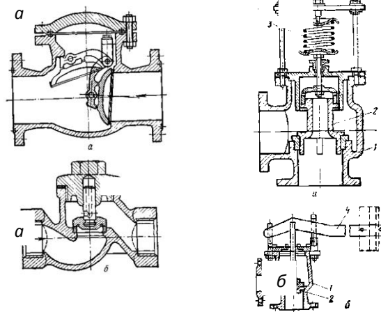
Рис. 4.16. Обратные клапаны: а – поворотный; б – подъемный Рис. 4.17. Предохранительные клапаны: а – пружинный; б – рычажно-грузовой; 1 – корпус; 2 – клапан; 3 – пружина; 4 – рычаг
