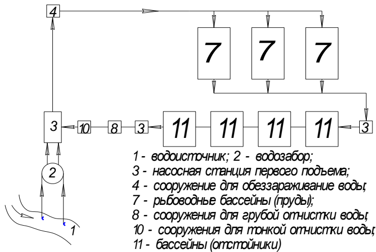
Рис. 3.3. Замкнутая напорная схема водоснабжения:
