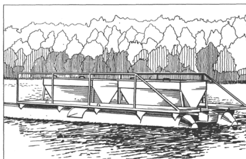
Рис. 7.15. Многомаятниковая автокормушка «Рефлекс Т-1500»
