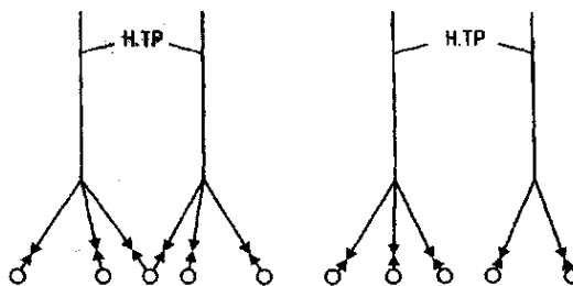
Рис. 4.12. Схемы объединения напорных трубопроводов
