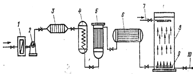
Рис. 5.8. Схема озонаторной установки:
