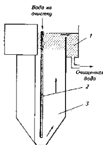
Рис. 5.13. Биофильтр с песчаной загрузкой: 1 – водосборное кольцо; 2 – водоподающая труба; 3 – загрузка (песок, удерживаемый во взвешенном состоянии током воды)
