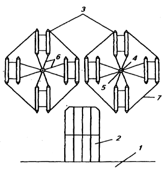
Рис. 7.16. Схема централизованного кормового места: 1 – дамба; 2 – эстакада; 3 – автокормушки; 4 – ось-штанга; 5 – ротор; 6 – жесткие лучи крепления; 7 – фалы
