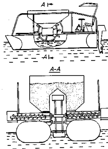
Рис. 7.2. Кормораздатчик КРБ-2
