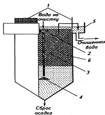
Рис. 5.15. Биофильтр с регенируемой загрузкой из полиэтиленовых гранул: 1 – сетка; 2 – приемная воронка; 3 – гидроэлеватор; 4 – отбойная тарелка; 5 – водосборное кольцо; 6 – загрузка (полиэтиленовые гранулы диаметром 2,5 мм)
