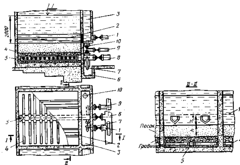
Рис. 5.4. Скорый фильтр:
