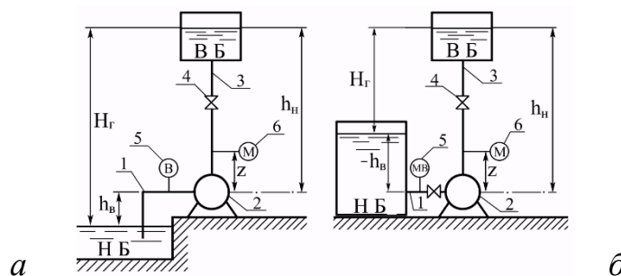
Рис. 4.4. Схемы насосной установки:
