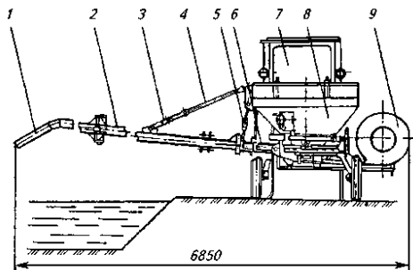
Рис. 7.3. Кормораздатчик ПД-0,6:
