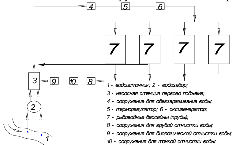
Рис. 3.1. Замкнутая самотечная схема водообеспечения
