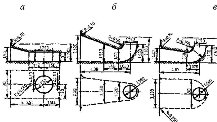
Рис. 4.11. Формы подводящих трубопроводов: а – с камерным подводом; б и в – с коленчатым подводом
