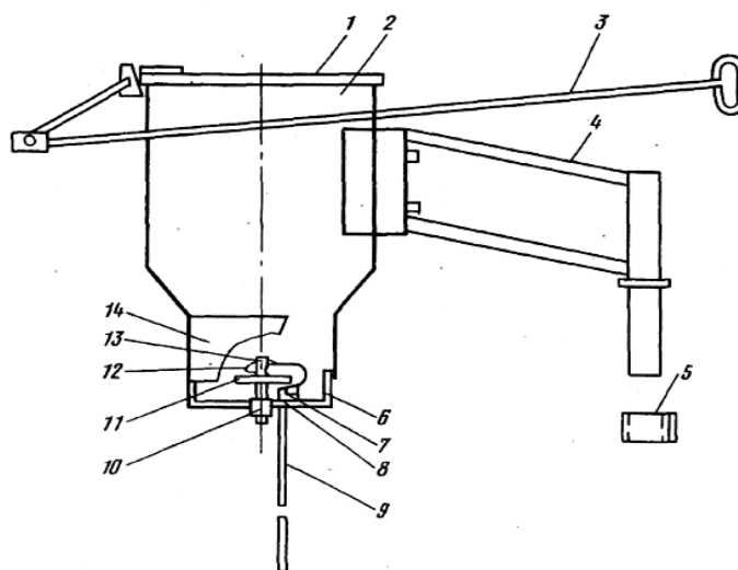
Рис. 7.14. Автокормушка «Рефлекс Т-1-50»:
