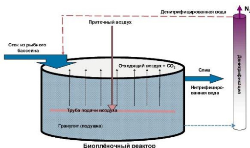
Рис. 5.11. Принцип действия биофильтра (биологическая нитрификация / денитрификация)
