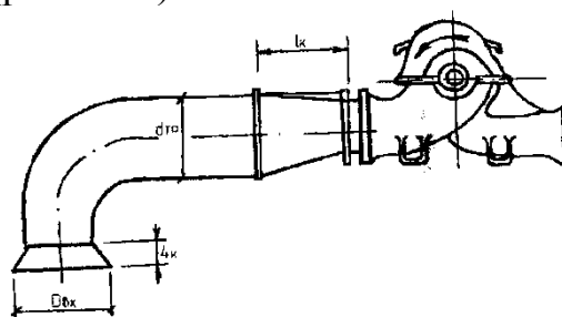
Рис. 4.10. Схема всасывающей трубы насоса
