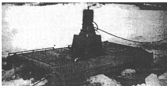
Рис. 6.13. Турбоаэратор Н-19-ИАК
