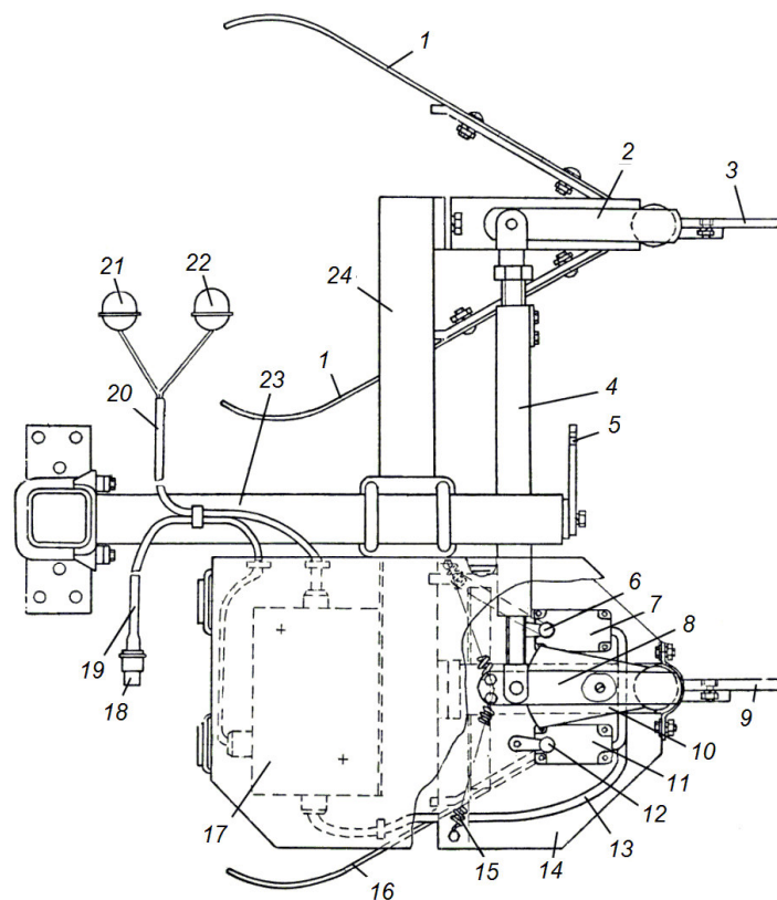
Рис. 2. Система вождения по рядкам: 1, 16 – щупы; 2, 8 – рычаги; 3, 9 – делители ботвы; 4 – шатун; 5 – визир; 6, 12 – толкатели; 7, 11 – выключатели; 10 – пластина; 13 – жгут выключателей; 14 – кожух; 15 – пружина; 17 – блок сигнализации; 18 – вилка питания; 19 – кабель питания; 20 – жгут фонарей; 21, 22 – фонари; 23 – кронштейн удерживающий; 24 – рамка
