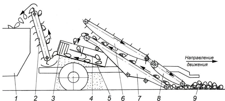
Рис. 6. Технологическая схема работы подборщика-погрузчика корнеплодов ППК-6: 1 – транспортное средство; 2 – погрузочный транспортер; 3 – отсекающий; 4 – амортизатор; 5 – сепарирующий ротор; 6 – прижимной транспортер; 7 – подбирающий транспортер; 8 – передний транспортер; 9 – корнеплоды
