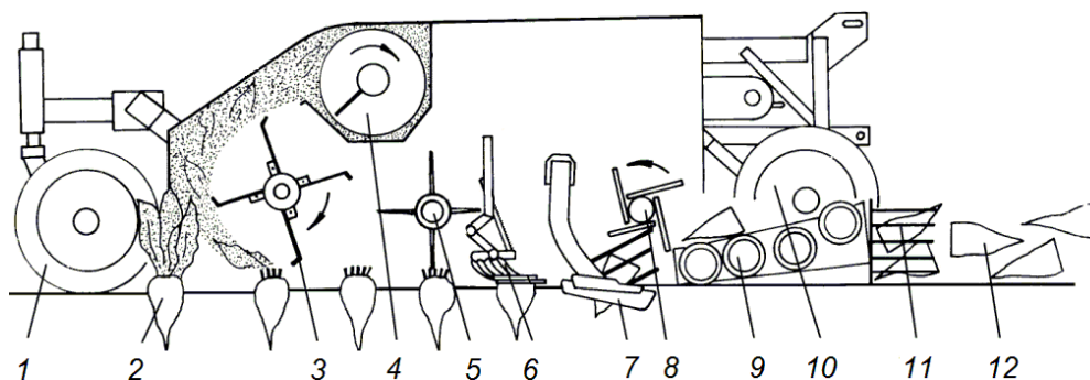
Рис. 1. Схема технологического процесса комбайна КСН-6:
