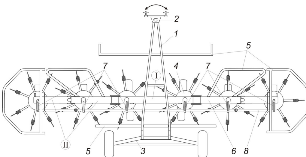
Рис. 6. Схема ворошителя-вспушителя роторного ВВР-7,5 в рабочем положении: 1 – рама; 2 – навесное устройство; 3 – колесный ход; 4 – роторы; 5 – защитные ограждения; 6 – поперечный брус; 7 – рычаги; 8 – тяга
