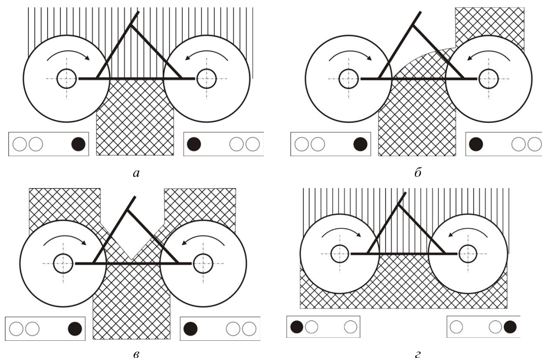
Рис. 3. Варианты установки копилов при выполнении технологических операций: а – сгребание; б – оборачивание вала; в – сдваивание валков; г – ворошение; ● ○ ○ – положение фиксатора рукоятки копира
