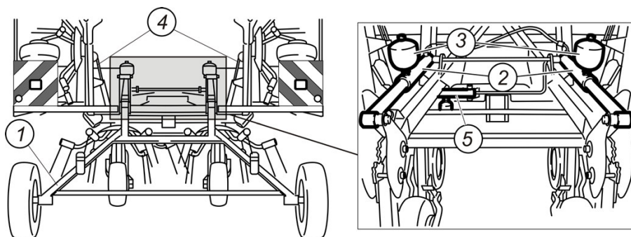
Рис. 7. Схема расположения гидроцилиндров колесного хода: 1 – колесный ход; 2, 4, 5 – гидроцилиндры; 3 – пневмоаккумуляторы
