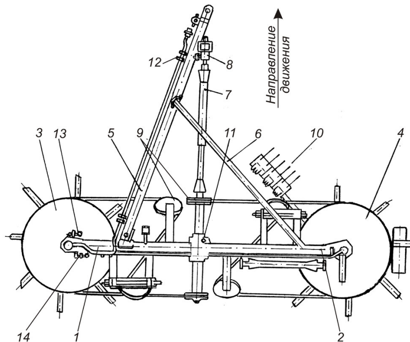
Рис. 1. Схема граблей ГВР-630 (рабочее положение):
