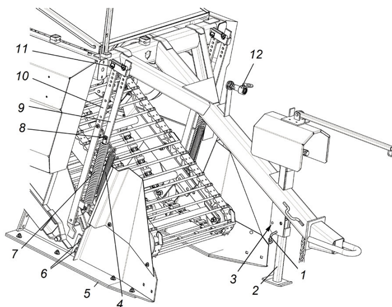
Рис. 8. Передняя часть подборщика-погрузчика: 1 – фиксатор; 2 – опора стояночная; 3 – отверстие; 4, 7 – пружины; 5 – копир; 6, 8 – болты; 9, 10 – пластины; 11 – ось; 12 – полумуфта гидравлическая
