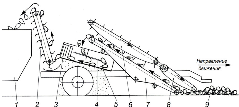
Рис. 6. Технологическая схема работы подборщика-погрузчика корнеплодов ППК-6:
