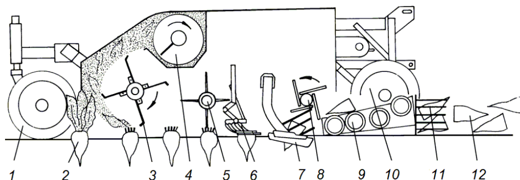
Рис. 1. Схема технологического процесса комбайна КСН-6:
