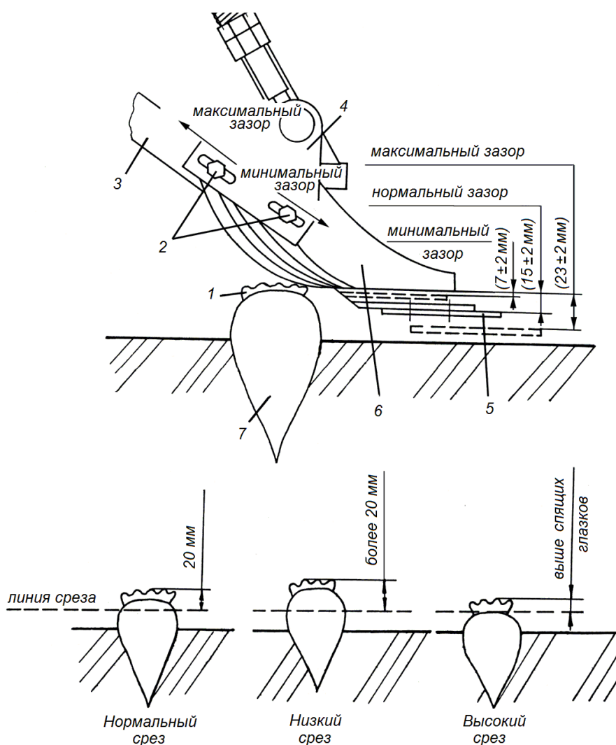
Рис. 5. Установка зазора между ножом и копиром: 1 – черешок корнеплода; 2 – болты; 3 – держатель ножа; 4 – опора ножа; 5 – нож; 6 – копир; 7 – корнеплод
