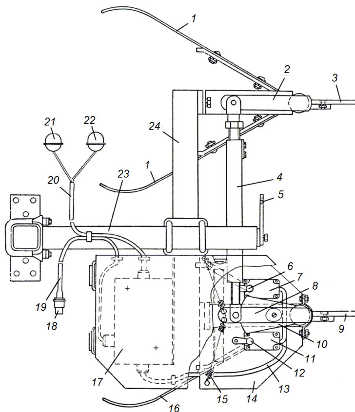
Рис. 2. Система вождения по рядкам:
