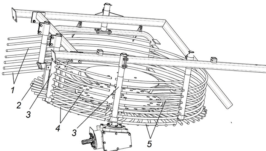
Рис. 7. Сепарирующий ротор с ограждением: 1 – длинная секция; 2 – ротор; 3 – стойки; 4, 5 – короткие секции
