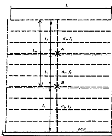
Рис. 8.1. Схема к расчету закрытого коллектора
