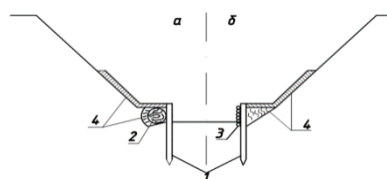
Рис. 8.5. Крепление каналов: а – хворостяным канатом (2); б – плетневой стенкой (3); 1 – кольца; 4 – дерн
