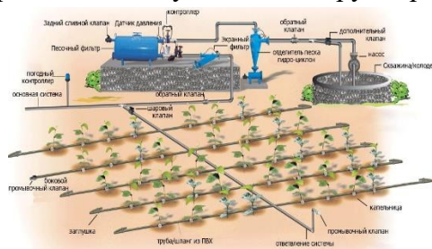
Рис. 23.2. Принципиальная схема системы капельного орошения
