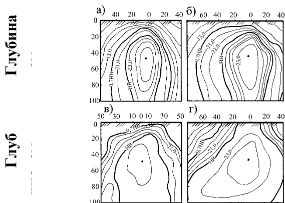
Рис. 23.1. Формирование контуров увлажнения почвы вокруг увлажнителя диаметром 50 мм под действием напора: а – H = 0,25 м; б – H = 0,50 м; в – H = 0,75 м; г – H = 1,0 м
