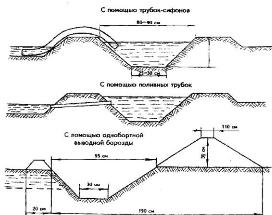
Рис. 22.4. Виды водовыпусков
