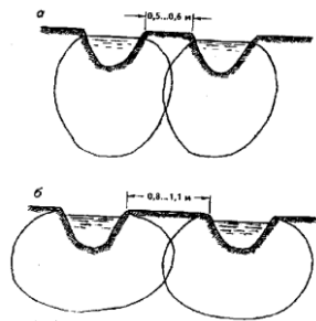
Рис. 22.3. Схемы контуров увлажнения почвы при поливе по бороздам:
