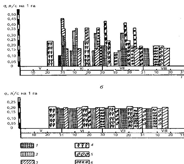
Рис. 22.1. Неукomплектованный (а) и укomплектованный (б) графики полива:
