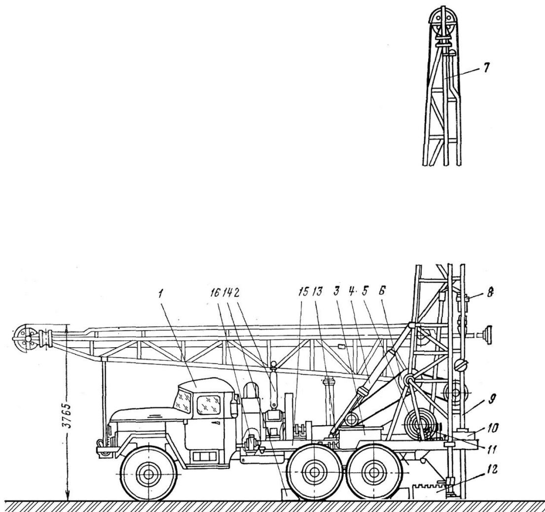
Рис. 5.4 – Установка роторного бурения УРБ 2,5А:
