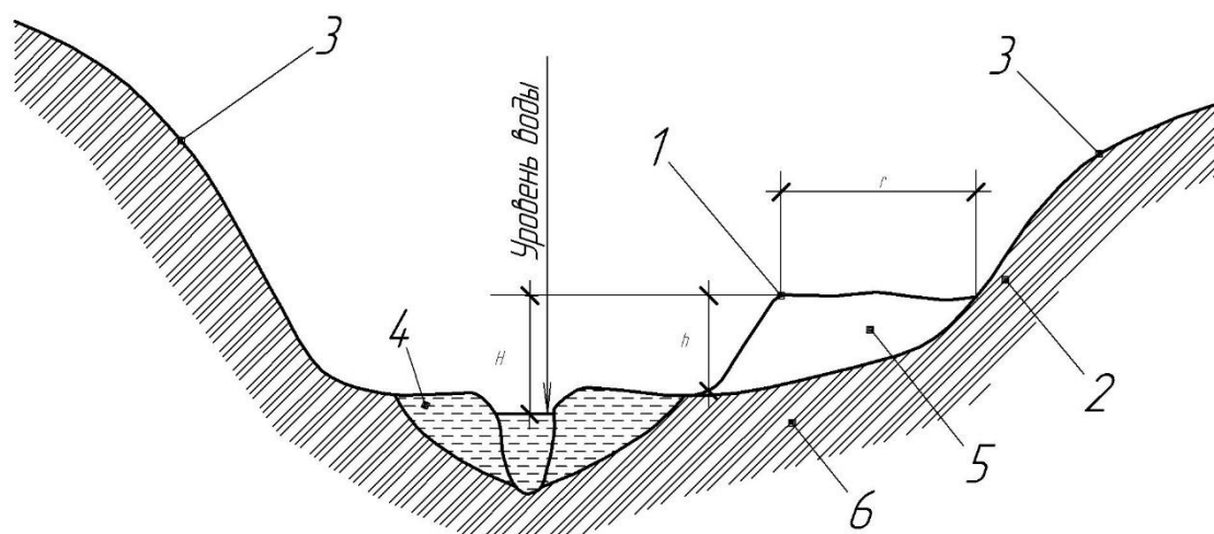
Рис. 5.8 – Элементы террасы:
