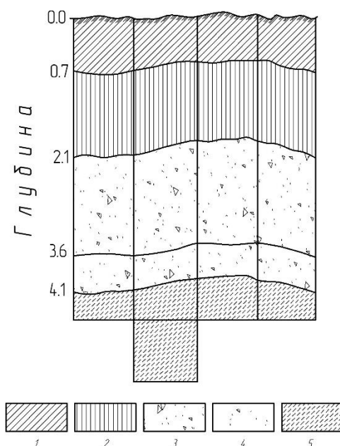
Рис. 5.5 – Развертка шурфа: 1 – суглинок пылеватый; 2 – лессовидный суглинок; 3 – песок с гравием; 4 – песок; 5 — супесь с гравием
