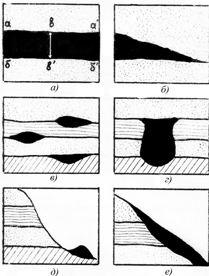
Рис. 3.1. Формы залегания осадочных пород: а) пласт: aa' – кровля пласта, bb' – подошва пласта, vv' – мощность пласта; б) выклинивание пласта; в) линзы; г) карман; д) вал; е) шлейф
