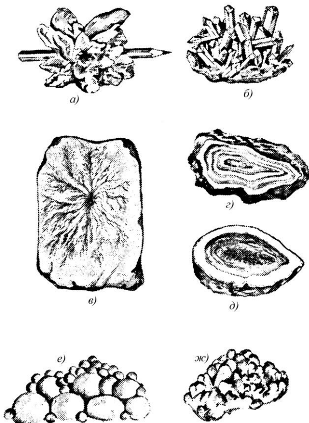
Рис. 1.5. Формы нахождения минералов в природе: а, б) друзы кристаллов гипса и кварца; в) дендрит марганцевых соединений на известняке; г) секрция; д) жеода; е) шаровидные конкреции; ж) почковидные натечные формы
