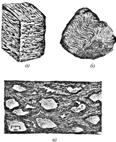
Рис. 4.1. Текстура метаморфических горных пород: а) сланцеватая; б) плойчатая; в) очковая
