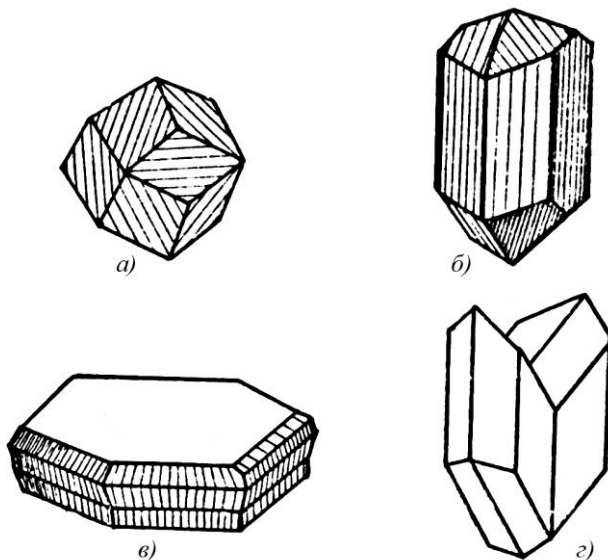
Рис. 1.4. Формы кристаллов минералов: а ) изометрическая (магнетит); б ) вытянутая в одном направлении (антимонит); в ) вытянутая в двух направлениях (хлорит); г ) двойник кристаллов гипса
