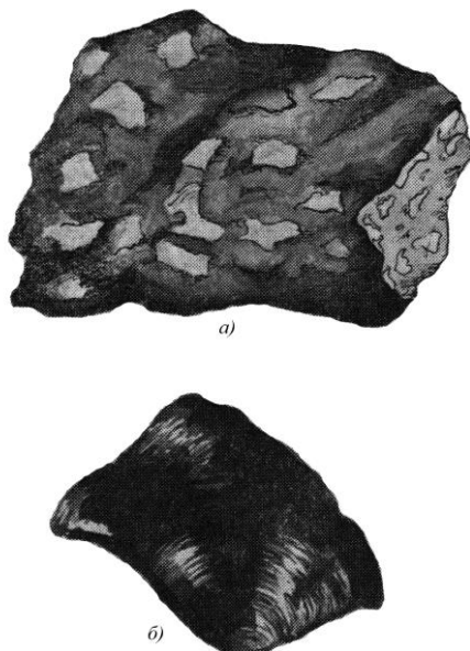
Рис. 2.2. Структура интрузивных пород: а) пегматитовая; б) полнокристаллическая, неравномерно-зернистая (порфировидная); в) полнокристаллическая, равномерно-зернистая
