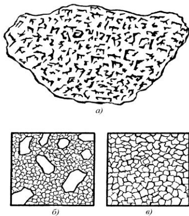
Рис. 2.2. Структура интрузивных пород: а) пегматитовая; б) полнокристаллическая, неравномерно-зернистая (порфировидная); в) полнокристаллическая, равномерно-зернистая
