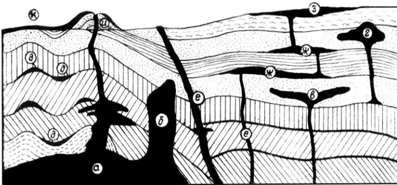
Рис. 2.1. Формы залегания магматических горных пород: а) батолит; б) шток; в) лополит; г) лакколит; д) факолит; е) магматические жилы (дайки); ж) силлы; з) покров; и) вулканический конус; к) лавовый поток
