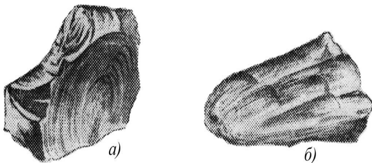
Рис. 1.3. Виды излома минералов: а) раковистый (кварц); б) занозистый (роговая обманка)
