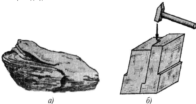
Рис. 1.2. Виды спайности минералов: а) весьма совершенная (слюда); б) совершенная (кальцит)
