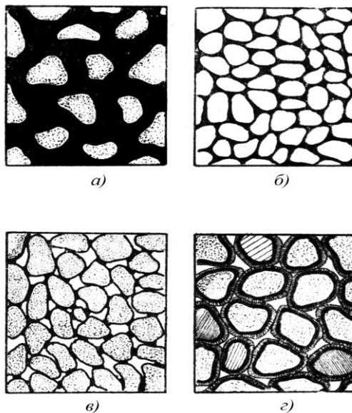
Рис. 3.2. Типы цементации (по М.С. Швецову): а) цемент базальный; б) цемент пор; в) цемент контактовый; з) цемент обрастания
