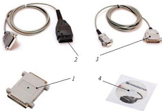
Рис. 2.3. Диагностический сканер «Сканматик»: 1 – адаптер; 2 – кабель OBDII; 3 – кабель подключения к COM-порту компьютера; 4 – диск с программным обеспечением
