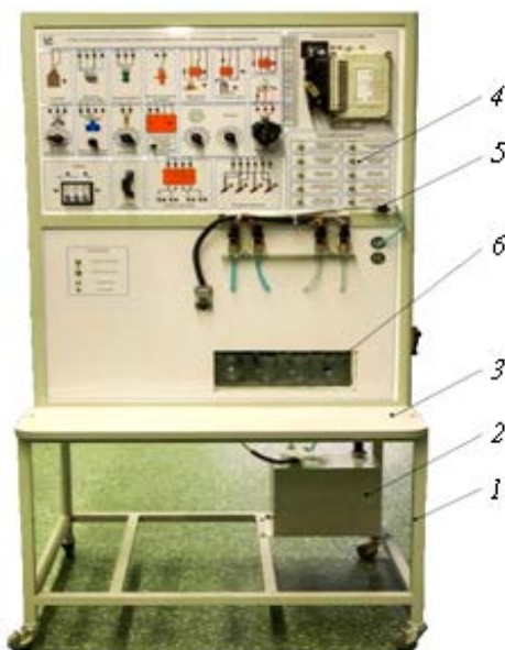
Рис. 2.1. Лабораторный стенд: 1 – рама; 2 – топливный бак с бензонасосом и фильтром; 3 – стол; 4 – панель управления стендом; 5 – топливная рампа с форсунками; 6 – блок мерных мензурок
