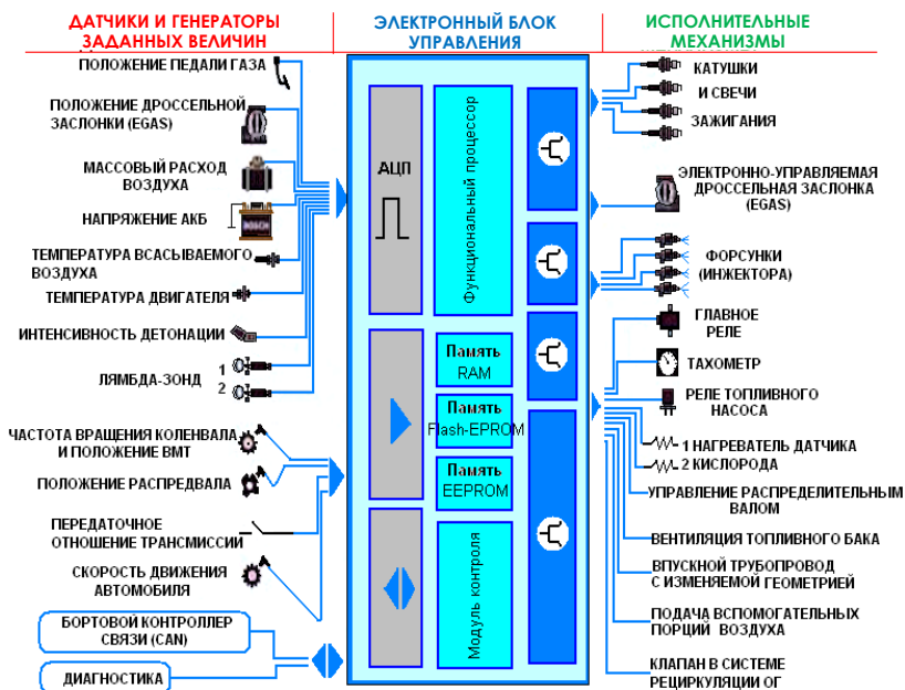
Рис. 1.2. Схема электронной системы управления впрыском
