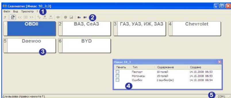
Рис. 2.4. Главное окно программы «Сканматик»: 1 – меню команд; 2 – панель инструментов; 3 – рабочая область программы; 4 – окно отчета; 5 – строка состояния
