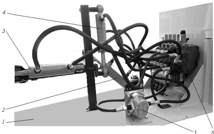
Рис. 3.3. Модуль гидравлики: 1 – рама; 2 – гидроцилиндр подъема плуга; 3 – гидроцилиндр изменения ширины захвата; 4 – гидроцилиндр оборота плуга; 5 – гидромотор; 6 – интегральный распределитель
