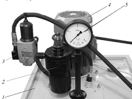
Рис. 3.4. Гидростанция: 1 – бак для масла; 2 – фильтр очистки масла; 3 – редукционный клапан; 4 – электродвигатель привода масляного насоса; 5 – манометр давления масла
