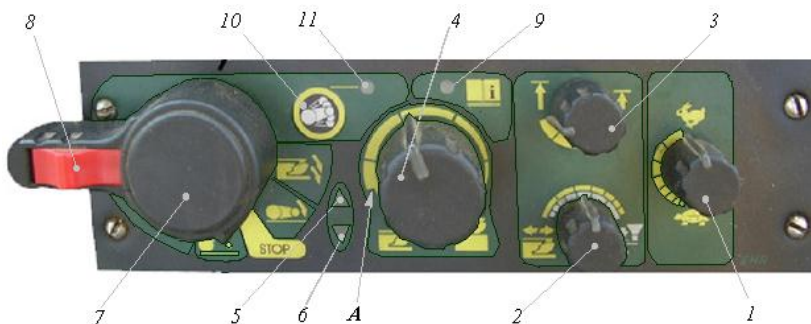
Рис. 1.2. Пульт управления ЗНУ: 1 – рукоятка регулирования скорости опускания; 2 – рукоятка выбора способа регулирования; 3 – рукоятка регулирования ограничения высоты подъема навески; 4 – рукоятка регулирования глубины обработки почвы; 5 – сигнализатор подъема ЗНУ (красного цвета); 6 – сигнализатор опускания НУ (зеленого цвета); 7 – рукоятка управления навесным устройством; 8 – фиксатор блокировки рукоятки управления навесным устройством; 9 – сигнализатор диагностики неисправностей (красного цвета); 10 – кнопка включения режима «демпфирование»; 11 – сигнализатор включения режима «демпфирование» (красного цвета)
