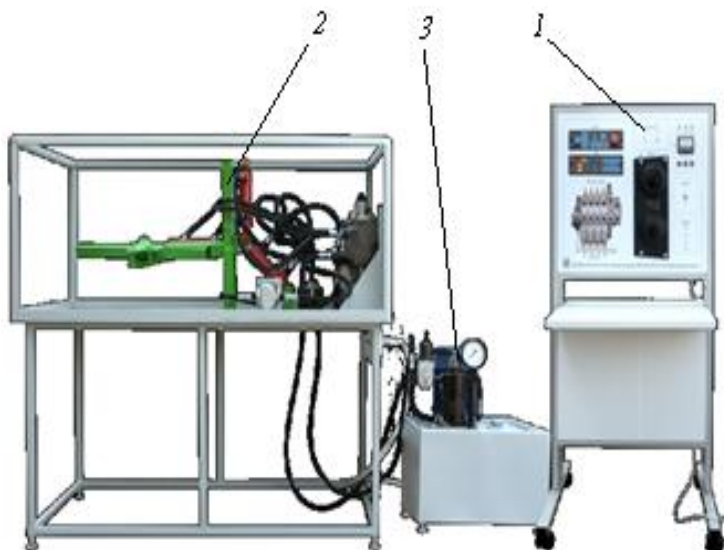
Рис. 3.1. Учебный лабораторный стенд НТЦ-105.000 «Электронная система управления секциями распределителей ЕНС внешних потребителей (БЕЛАРУС-3022.1)»: 1 – модуль электроавтоматики; 2 – модуль гидравлики; 3 – гидростанция
