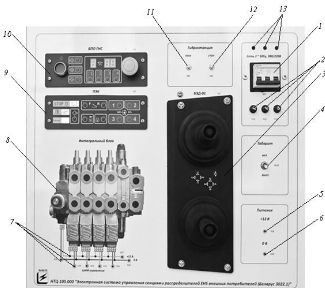
Рис. 3.2. Панель управления стендом (модуль электроавтоматики): 1 – выключатель «сеть»; 2 – предохранитель; 3 – блок джойстиков БЭД-1; 4 – включатель габаритов; 5 и 6 – порты для измерения напряжения питания; 7 – измерительные порты для мультиметра; 8 – интегральный распределительный блок; 9 – панель электронная комбинированная; 10 – блок программирования операций ГНС; 11 – кнопка включения гидростанции; 12 – кнопка выключения гидростанции; 13 – световые индикаторы подключения стенда к сети
