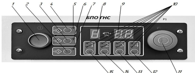
Рис. 2.1. Блок программирования операций ГНС: 1 – выключатель питания БПО ГНС; 2 – кнопка программы № 3; 3 – кнопка программы № 2; 4 – кнопка программы № 1; 5 – сигнализатор программы № 1; 6 – сигнализатор программы № 2; 7 – сигнализатор программы № 3; 8 – цифровой индикатор номера работающей секции гидрораспределителя; 9 – цифровой индикатор величины потока масла по работающей секции; 10 – сигнализаторы подъема и опускания соответствующих секций гидрораспределителя; 11 – выключатель STOP аварийного останова гидрораспределителя; 12 – кнопка выбора секции № 4 гидрораспределителя; 13 – кнопка выбора секции № 3 гидрораспределителя; 14 – кнопка выбора секции № 2 гидрораспределителя; 15 – кнопка выбора секции № 1 гидрораспределителя
