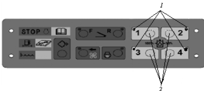
Рис. 1.5. Элементы ПЭК включения и индикации ограничения потока по секциям гидрораспределителя EHS: 1 – сигнализаторы включения ограничения потока по секции гидрораспределителя; 2 – кнопки включения ограничения потока по секции гидрораспределителя
