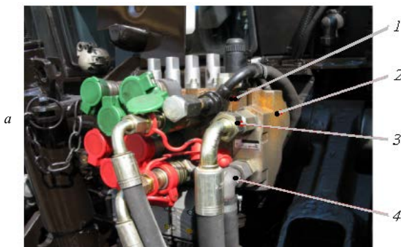
Рис. 1.2. Интегральный блок распределителя: а – вид сзади справа; б – вид слева; 1 – секция управления ЗНУ EHR-23LS; 2 – насосная секция; 3 – напорная магистраль насосной секции; 4 – сливная магистраль насосной секции; 5 – секции EHS (нумерация начинается от секции EHR-23LS); 6 – заглушка фильтра грубой очистки; 7 – концевая плита с редукционным клапаном; 8 – крышка фильтра тонкой очистки; 9 – редукционный клапан; 10 – сигнализаторы неисправностей работы секций EHS
