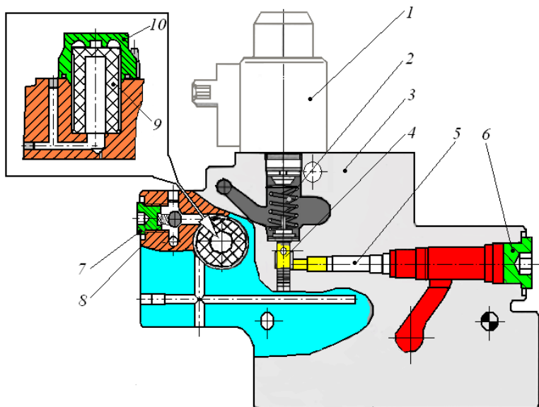
Рис. 1.3. Концевая плита: 1 – включающий электромагнит редукционного клапана; 2 – пружина редукционного клапана; 3 – корпус; 4 – редукционный клапан; 5 – фильтр грубой очистки; 6 – заглушка фильтра грубой очистки; 7 – крышка перепускного клапана фильтра тонкой очистки; 8 – пружина перепускного клапана фильтра тонкой очистки; 9 – фильтр тонкой очистки; 10 – крышка фильтра тонкой очистки
