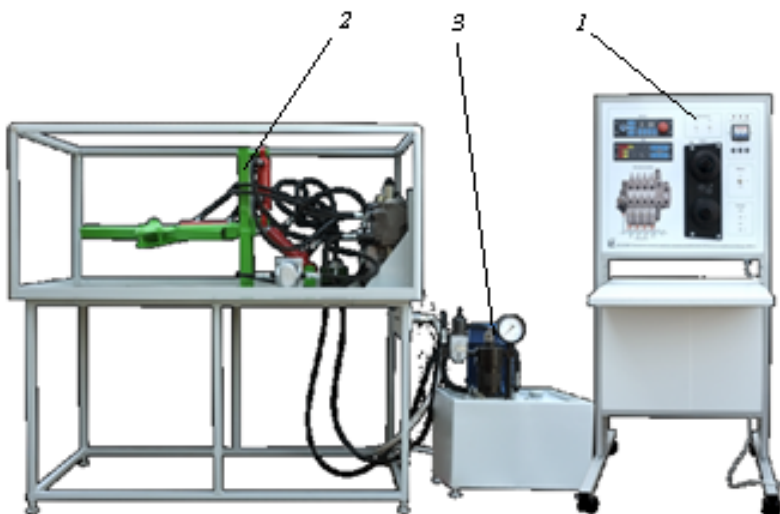
Рис. 3.1. Учебный лабораторный стенд НТЦ-105.000 «Электронная система управления секциями распределителей ЕНС внешних потребителей (БЕЛАРУС-3022.1)»: 1 – модуль электроавтоматики; 2 – модуль гидравлики; 3 – гидростанция
