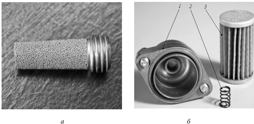
Рис. 1.4. Внешний вид фильтров: a – фильтр грубой очистки; б – фильтр тонкой очистки с крышкой: 1 – крышка фильтра тонкой очистки; 2 – пружина; 3 – бумажный фильтр
