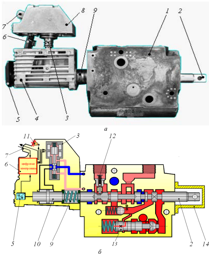
Рис. 1.6. Секция EHS: а – внешний вид (подразобранное состояние); б – внутреннее устройство: 1 – корпус секции EHS; 2 – центральный золотник; 3 – электромагнитный клапан управления; 4 – корпус блока управления секцией EHS; 5 – индуктивный датчик положения; 6 – цифровая электронная плата; 7 – контактный штыревой разъем; 8 – крышка блока управления секцией EHS; 9 – возвратная пружина; 10 – поршень исполнительного механизма; 11 – световой индикатор кодов неисправностей; 12 – запорный клапан; 13 – клапан разности давлений; 14 – защитный колпачок
