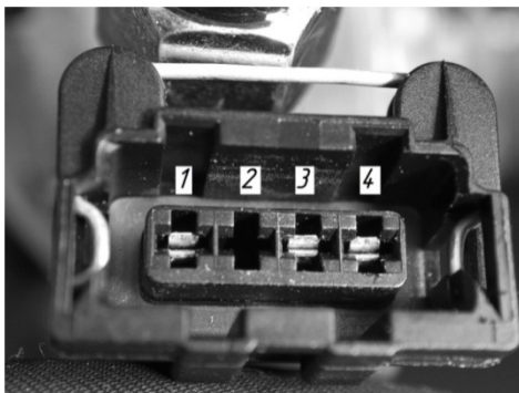
Рис. 1.9. Разъем подключения секции EHS
