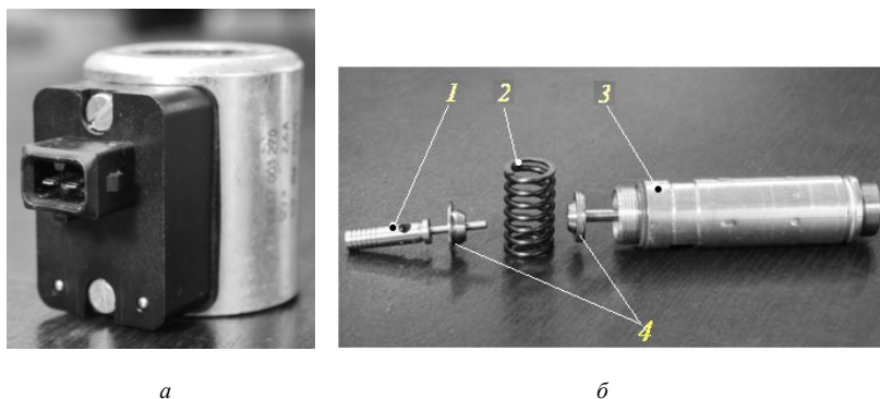
Рис. 1.5. Электромагнитный редукционный клапан: a – электромагнит редукционного клапана; б – редукционный клапан в разобранном виде (без электромагнита): 1 – клапан; 2 – пружина; 3 – сердечник электромагнита; 4 – регулировочные шайбы
