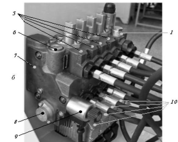
Рис. 1.2. Интегральный блок распределителя: а – вид сзади справа; б – вид слева; 1 – секция управления ЗНУ EHR-23LS; 2 – насосная секция; 3 – напорная магистраль насосной секции; 4 – сливная магистраль насосной секции; 5 – секции EHS (нумерация начинается от секции EHR-23LS); 6 – заглушка фильтра грубой очистки; 7 – концевая плита с редукционным клапаном; 8 – крышка фильтра тонкой очистки; 9 – редукционный клапан; 10 – сигнализаторы неисправностей работы секций EHS
