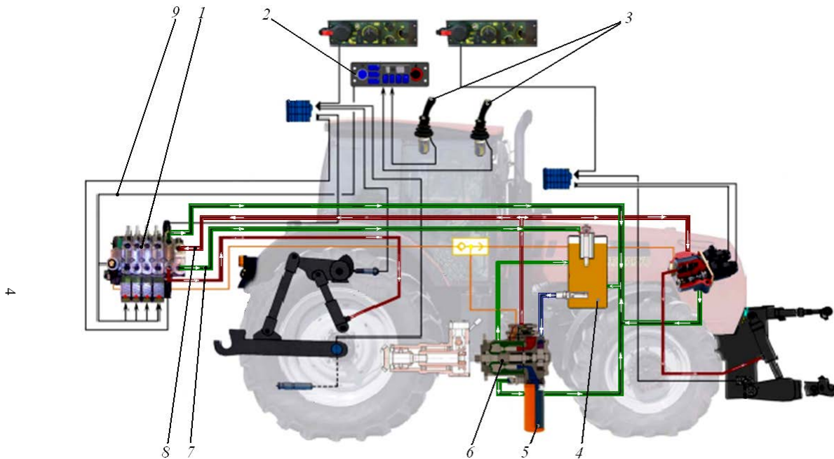
Рис. 1.1. Электрогидравлическая схема гидронавесной системы тракторов марки «Беларус» с джойстиковым управлением (на рисунке обозначены позиции, относящиеся к электрогидравлической системе управления секциями EHS): 1 – интегральный распределитель; 2 – программатор; 3 – джойстики; 4 – маслобак; 5 – фильтр аксиально-поршневого насоса; 6 – аксиально-поршневой насос; 7 – сливная магистраль; 8 – напорная магистраль; 9 – электрические провода, соединяющие программатор и секции EHS
