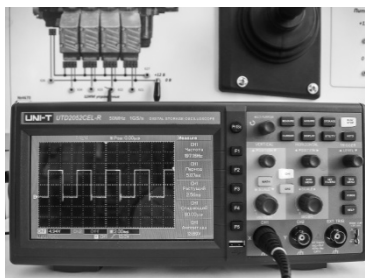
Рис. 3.5. Измерение напряжения: а – мультиметром; б – осциллографом
