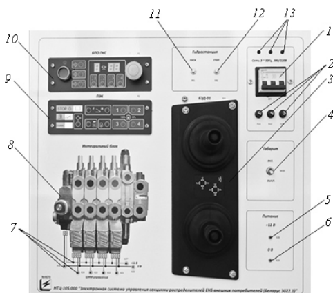
Рис. 3.2. Панель управления стендом (модуль электроавтоматики): 1 – выключатель «сеть»; 2 – предохранители; 3 – блок джойстиков БЭД-1; 4 – выключатель габаритов; 5, 6 – порты для измерения напряжения питания; 7 – измерительные порты для мультиметра; 8 – интегральный распределительный блок; 9 – панель электронная комбинированная; 10 – блок программирования операций ГНС; 11 – кнопка включения гидростанции; 12 – кнопка выключения гидростанции; 13 – световые индикаторы подключения стенда к сети
