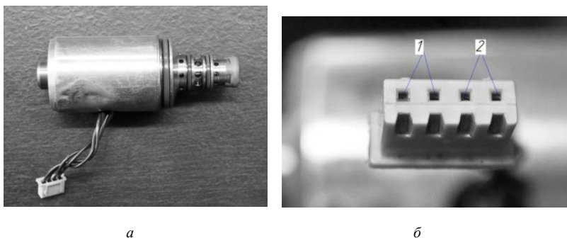
Рис. 1.7. Электромагнитный клапан управления: a – общий вид клапана с соединительными жгутами и разъемом; б – соединительный разъем клапана управления с нумерацией его обмоток
