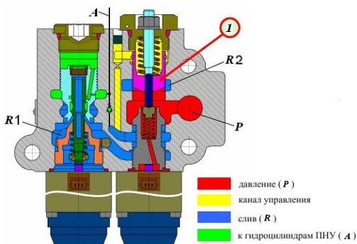
Рис. 18. Регулятор EHR-5LS.
