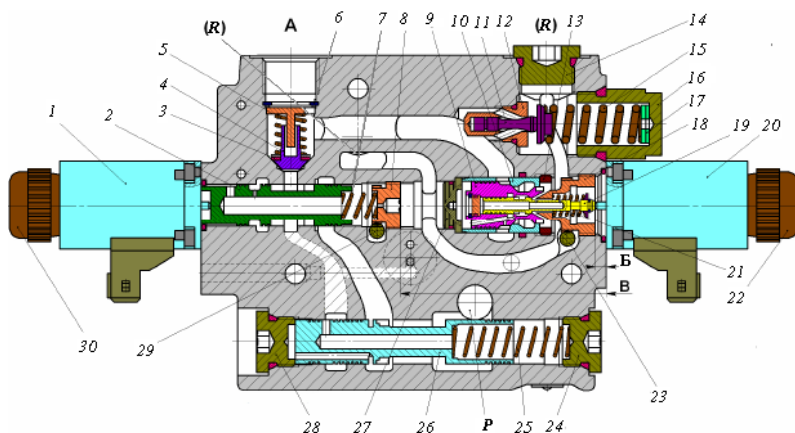
Рис. 10. Устройство регулятора EHR-23LS: 1 – электромагнит подъема; 2 – золотник подъема; 3 – уплотнение запорного клапана; 4 – запорный клапан; 5, 7, 15, 21, 25 – пружины; 6 – стопорное кольцо; 8, 18 – упоры пружин; 9 – клапан опускания; 10 – седло клапана опускания; 11 – противоударный клапан; 12 – седло противоударного клапана; 13 – гайка; 14, 16, 24, 27, 28 – пробки; 17 – регулировочные шайбы; 19 – управляющий золотник клапана опускания; 20 – электромагнит опускания; 22, 30 – колпачки-кнопки; 23, 29 – червяки; 26 – клапан-компенсатор (перепускной клапан); P – давление; R – слив; A – к гидроцилиндрам; B и B – справочные размеры
