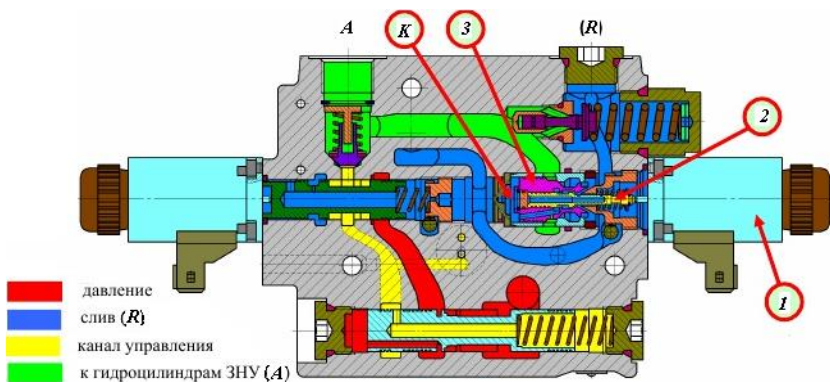
Рис. 13. Регулятор EHR-23LS. Опускание (первая стадия): 1 – электромагнит опускания; 2 – управляющий золотник клапана опускания; 3 – клапан опускания
