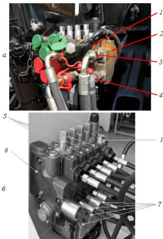
Рис. 4. Интегральный блок распределителя: а – вид сзади справа; б – вид слева; 1 – секция управления ЗНУ EHR-23LS; 2 – насосная секция; 3 – напорная магистраль насосной секции; 4 – сливная магистраль насосной секции; 5 – секции EHS (нумерация начинается от секции EHR-23LS); 6 – концевая плита с редукционным клапаном; 7 – сигнализаторы неисправностей работы секций EHS
