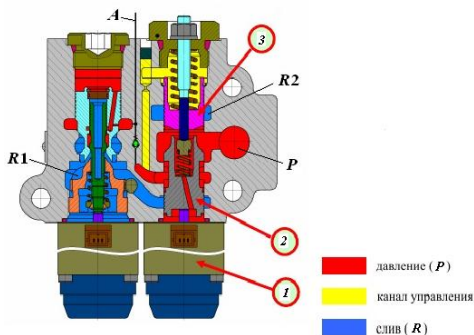
Рис. 19. Регулятор EHR-5LS. Положение «подъем»: 1 – перепускной клапан; 2 – золотник подъема; 3 – перепускной клапан; А – канал, соединенный с гидроцилиндрами ПНУ; R1 – сливной канал; R2 – слив канала управления
