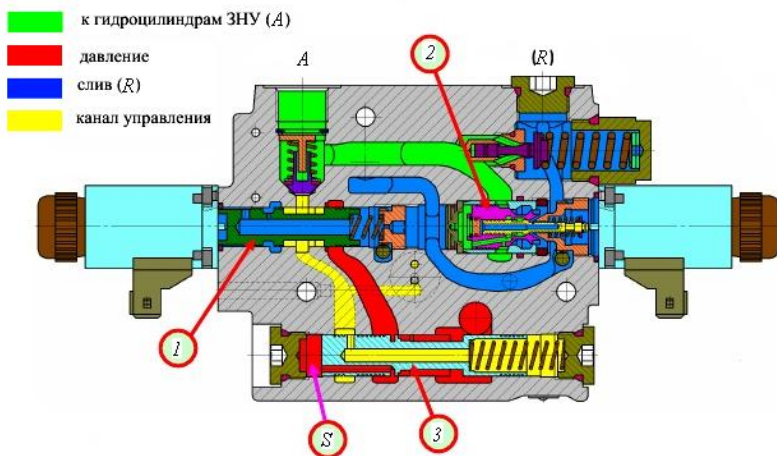
Рис. 11. Регулятор EHR-23LS. Нейтральное положение: 1 – золотник подъема; 2 – клапан опускания; 3 – клапан-компенсатор; S – полость клапана-компенсатора
