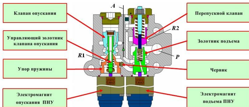
Рис. 17. Устройство регулятора EHR-5LS: P – напорный канал; R1 – сливной канал; R2 – слив канала управления; A – канал подачи масла к гидроцилиндрам ПНУ
