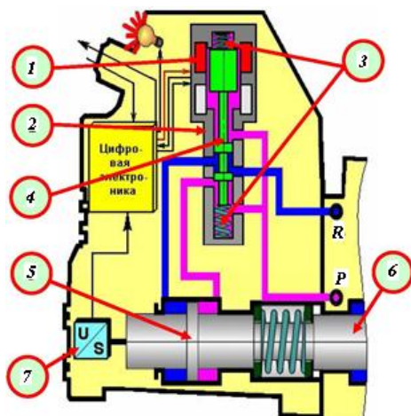
Рис. 8. Работа клапана управления и центральный золотник в положении «опускание» ( P – давление, R – слив); 1 – электромагнит «опускания»; 2 – клапан управления; 3 – возвратные пружины; 4 – направляющий золотник клапана управления; 5 – поршень исполнительного механизма; 6 – центральный золотник; 7 – индуктивный датчик положения
