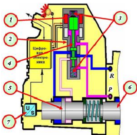
Рис. 9. Работа клапана управления и центральный золотник в положении «плавающее» ( P – давление, R – слив): 1 – электромагнит «плавающее»; 2 – клапан управления; 3 – возвратные пружины; 4 – направляющий золотник клапана управления; 5 – поршень исполнительного механизма; 6 – центральный золотник; 7 – индуктивный датчик положения
