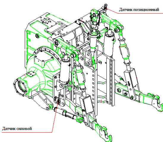
Рис. 2. Схема расположения силового и позиционного датчиков заднего навесного устройства
