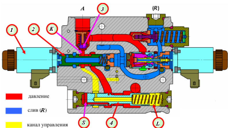
Рис. 12. Регулятор EHR-23LS. Положение «подъем»: 1 – электромагнит подъема; 2 – золотник подъема; 3 – запорный клапан; 4 – клапан-компенсатор
