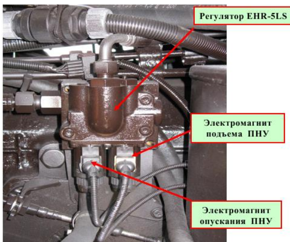
Рис. 22. Установка регулятора EHR-5LS на коробке передач
