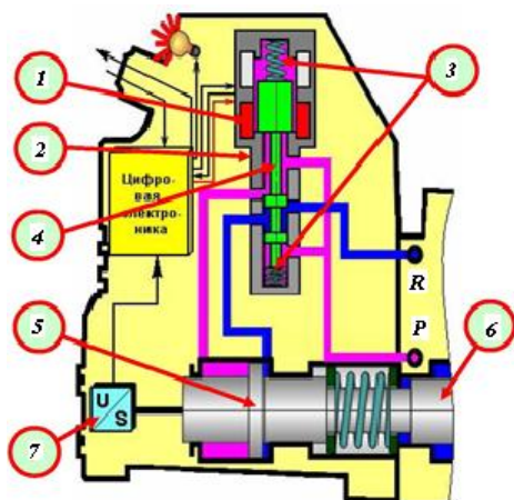
Рис. 7. Работа клапана управления и центральный золотник в положении «подъем» ( P – давление, R – слив); 1 – электромагнит «подъема»; 2 – клапан управления; 3 – возвратные пружины; 4 – направляющий золотник клапана управления; 5 – поршень исполнительного механизма; 6 – центральный золотник; 7 – индуктивный датчик положения
