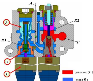
Рис. 21. Регулятор EHR-5LS. Положение «опускание» (вторая стадия): 1 – перепускной клапан; 2 – золотник подъема; 3 – перепускной клапан; A – канал, соединенный с гидроцилиндрами ПНУ; R1 – сливной канал; R2 – слив канала управления
