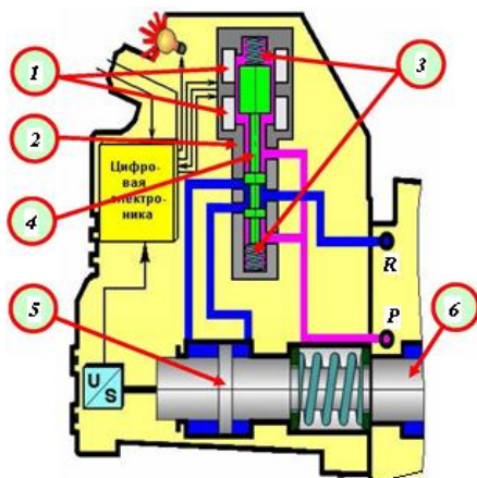
Рис. 6. Работа клапана управления и центральный золотник в положении «нейтраль» ( P – давление, R – слив): 1 – электромагниты; 2 – клапан управления; 3 – возвратные пружины; 4 – направляющий золотник клапана управления; 5 – поршень исполнительного механизма; 6 – центральный золотник
