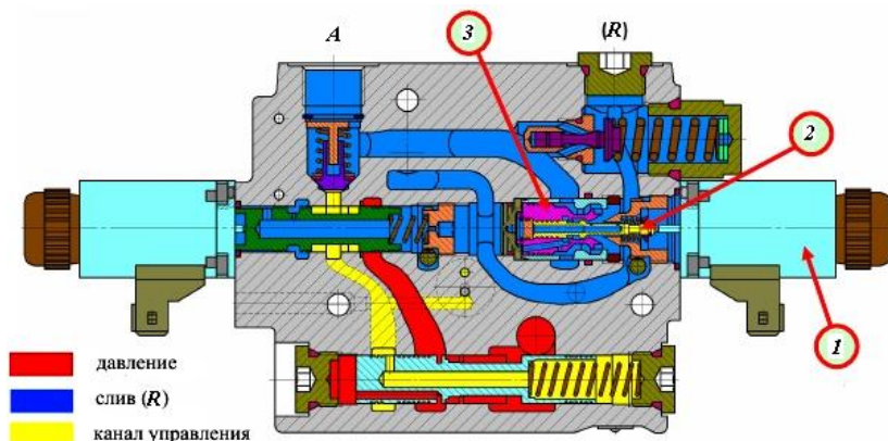
Рис. 14. Регулятор EHR-23LS. Вторая стадия положения «опускание»: 1 – электромагнит опускания; 2 – управляющий золотник клапана опускания; 3 – клапан опускания
