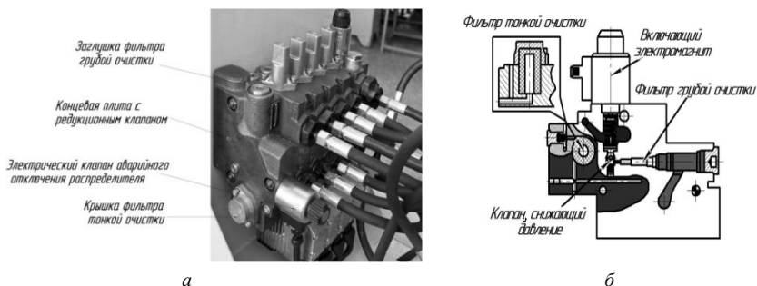
Рис. 15. Концевая плита с редукционным клапаном: а – расположение на интегральном блоке распределителя; б – устройство концевой плиты
