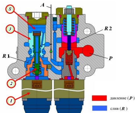
Рис. 20. Регулятор EHR-5LS. Положение «опускание» (первая стадия): 1 – перепускной клапан; 2 – золотник подъема; 3 – перепускной клапан; А – канал, соединенный с гидроцилиндрами ПНУ; R1 – сливной канал; R2 – слив канала управления
