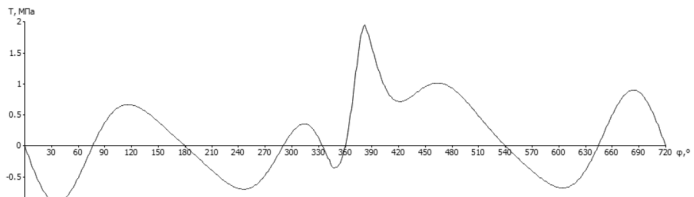
Рис. 2. Диаграмма тангенциальных сил
