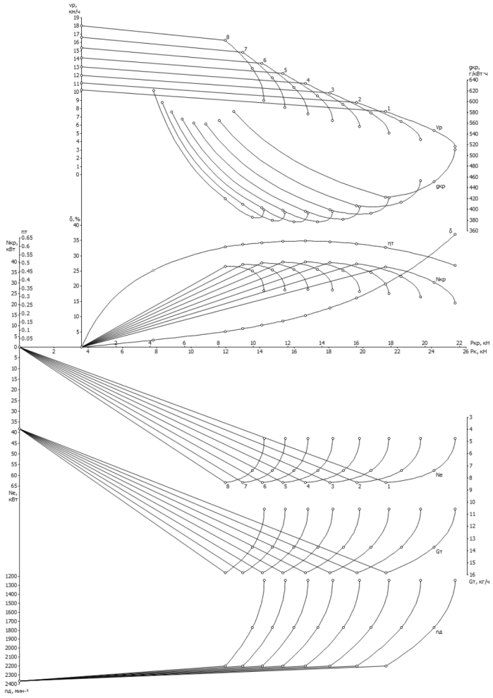
Рис. 5. Тяговая характеристика трактора
