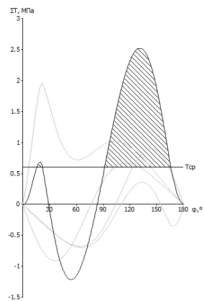
Рис. 3. Диаграмма суммарных тангенциальных сил
