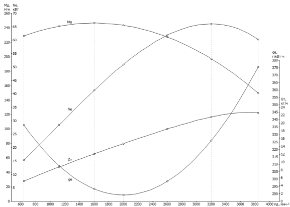
Рис. 4. Скоростная характеристика двигателя
