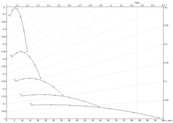
Рис. 5. Универсальная динамическая характеристика автомобиля
