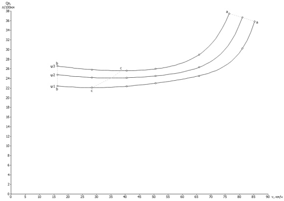
Рис. 6. Экономическая характеристика автомобиля
