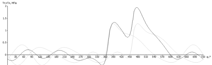
Рис. 2. Диаграмма тангенциальных сил
