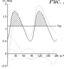
Рис. 3. Диаграмма суммарных тангенциальных сил
