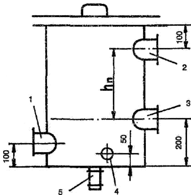
Рис. 8.1 - Открытый расширительный бак
