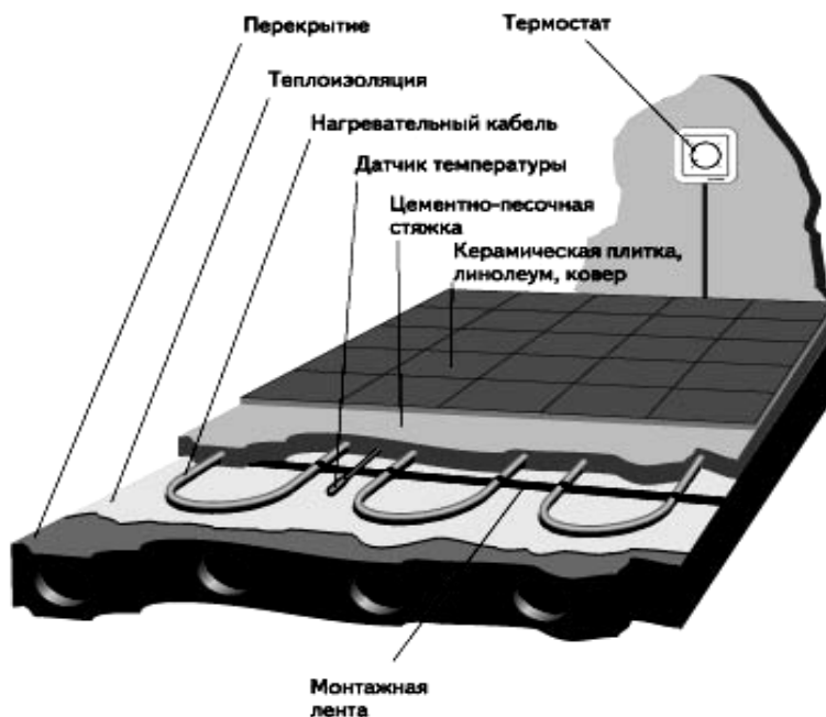
Рис. 11.2 - Конструкция электрического теплого пола
