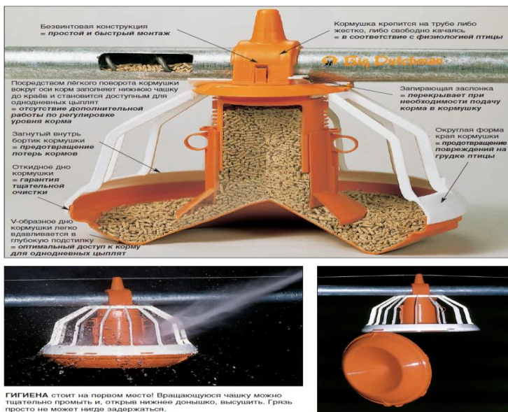
Рис. 57. Кормушки для птицы
