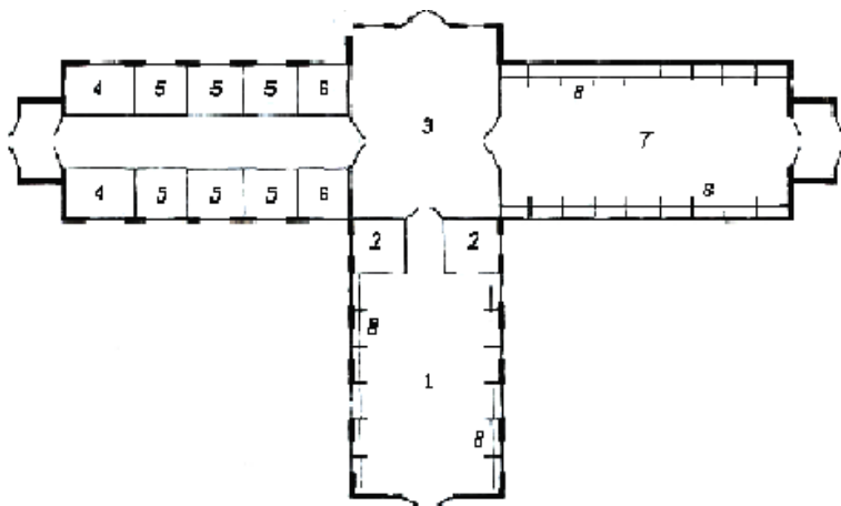
Рис. 90. Конюшня на 12 кобыл:
