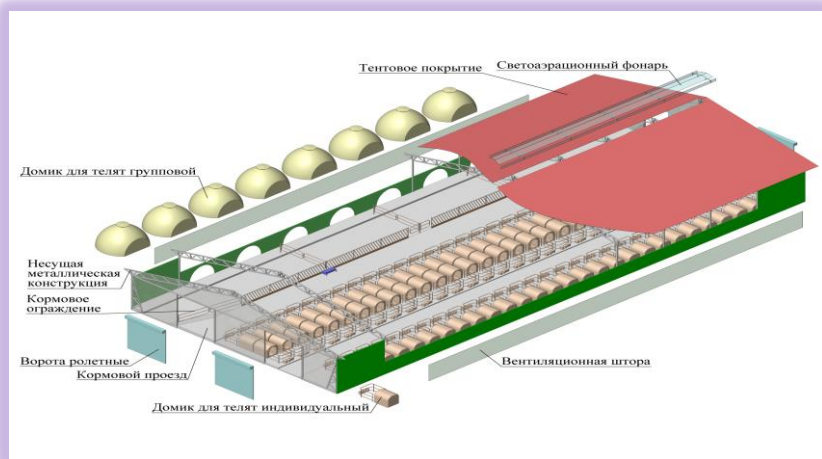
Рис. 24. Генплан телятника профилактория
