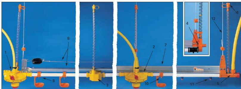
Рис. 60. Система поения птицы
