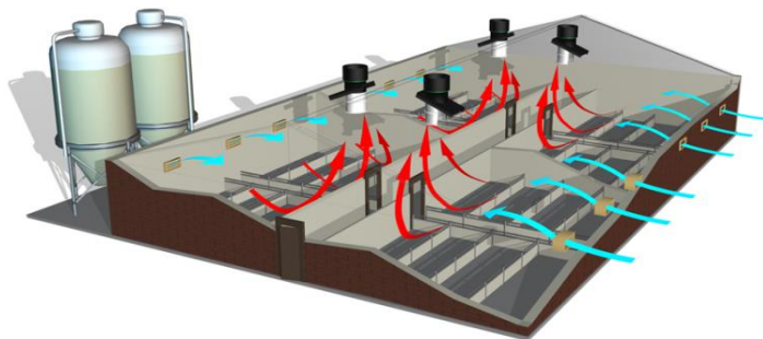
Рис. 37. Схема приточно-вытяжной вентиляции в свинарнике
