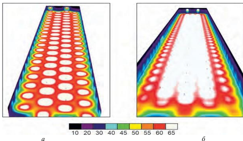
Рис. 5.2. Светотехнический расчет для птичника с напольным содержанием цыплят-бройлеров освещенностью 60 лк, оборудованного (на высоте 3 м) 84 светодиодными светильниками СН500-12-26-Т мощностью 12 Вт (а) и 165 светильниками СН300-6-13-Т 6 Вт (б) с 4 и 5 линиями освещения соответственно
