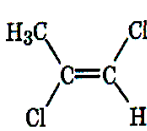
транс -1,2-дихлорпропен
