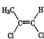
цис -1,2-дихлорпропен
