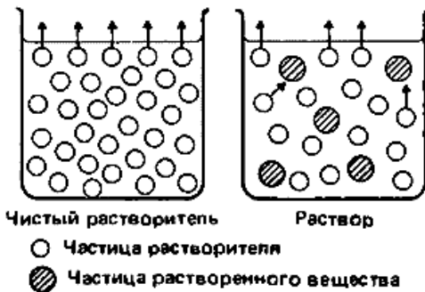
Рис. 9. Частицы нелетучего растворенного вещества препятствуют удалению с поверхности жидкости частиц растворителя и вследствие этого снижают давление пара
