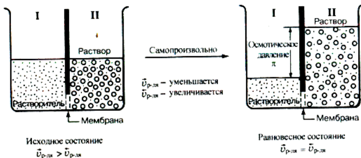
Рис. 3. Осмос в системе растворитель – раствор, разделенные мембраной с избирательной проницаемостью
