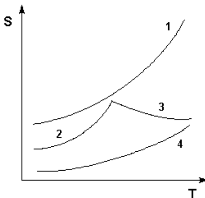
Рис. 2. Кривые растворимости некоторых солей в воде: 1 – \text{KNO}_3 ; 2 – \text{Na}_2\text{SO}_4 \cdot 10\text{H}_2\text{O} ; 3 – \text{Na}_2\text{SO}_4 ; 4 – \text{Ba}(\text{NO}_3)_2
