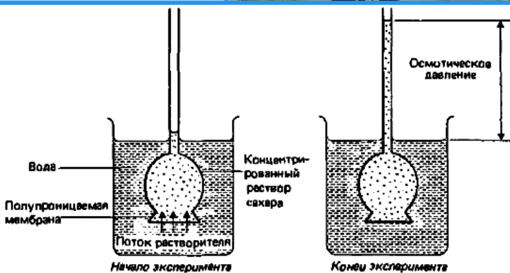
Рис. 7. Эксперимент, показывающий действие осмотического давления
