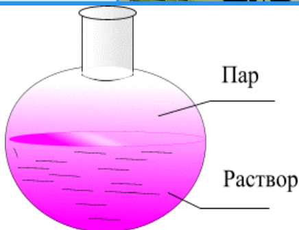
Рис. 8. Схема равновесия двухфазной системы раствор – пар
