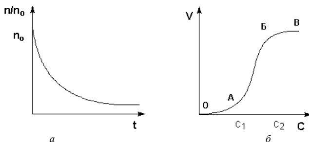
Рис. 7. Коагуляционная кривая (а) и зависимость скорости коагуляции от концентрации (б)
