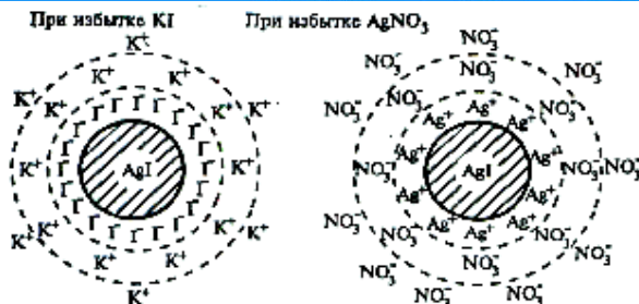
Рис. 3. Структура коллоидных частиц иодида серебра(I)
