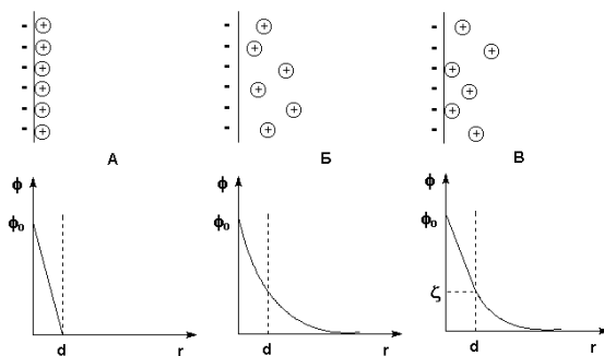
Рис. 5. Строение ДЭС: а – по Гельмгольцу и Перрену; б – по Гуи и Чепмену; в – по Штерну.
