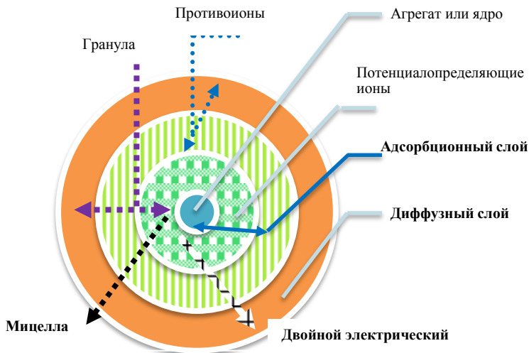
Рис. 2. Мицелла и двойной электрический слой
