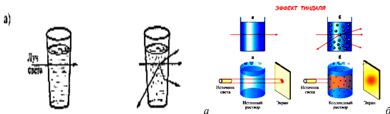
Рис. 4. Эффект светорассеяния при прохождении луча света через коллоидный раствор:
