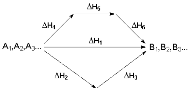
Рис. 2.1. Различные пути обобщенного химического процесса превращения
