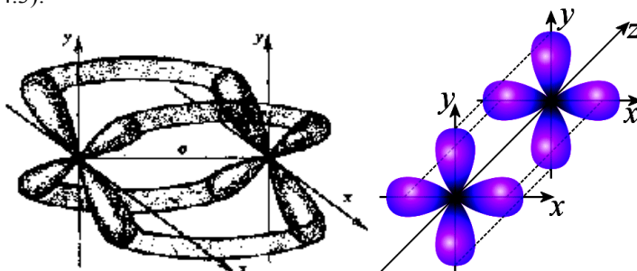
Рис. 4.3. Образование \delta -связи
