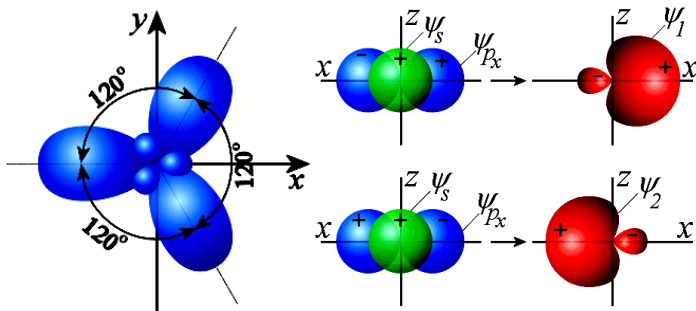
Рис. 4.4. Гибридные орбитали
