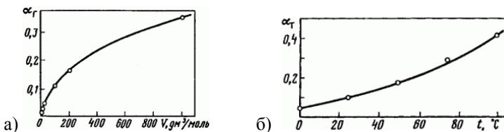
Рис. 9.1. Зависимость степени гидролиза карбоната натрия от разбавления при 20°C (а) и от температуры (б)
