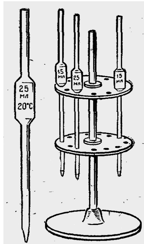
Пипетки Мора
