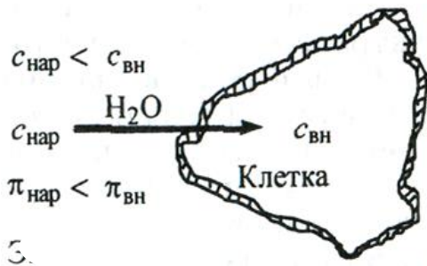
Рис. 3.5. Эндоосмос
