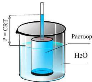
Рис. 3.4. Прибор для определения осмотического давления
