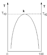
Рис. 3.1. Диаграмма растворимости системы анилин – вода
