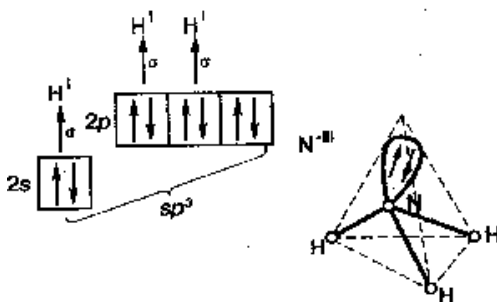
Рис. 4.8. Геометрия молекулы \text{NH}_3
