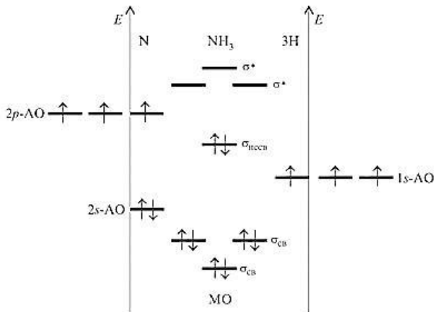
Рис. 4.11. Энергетическая диаграмма образования молекулы NH 3 по методу МО ЛКАО
