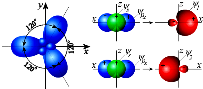
Рис. 4.4. Гибридные орбитали
