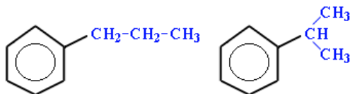
n-Пропилбензол
