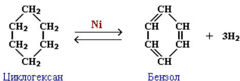
Циклогексан
