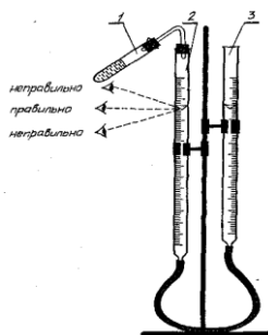
Рис. 1. Прибор для определения молярной массы эквивалента металла
