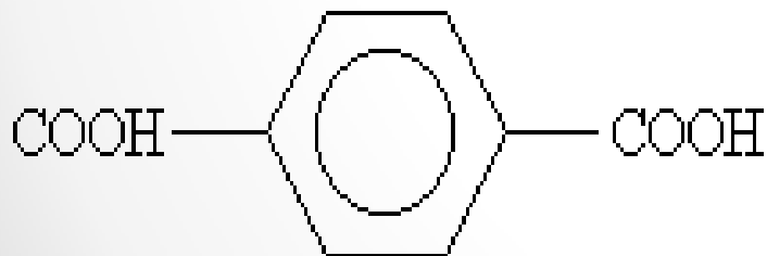
Бензол-1,4- дикарбоновая
