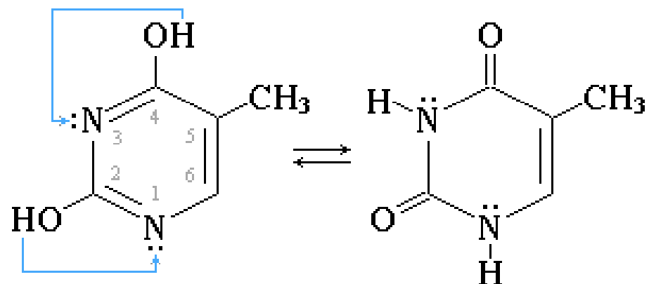
Тимин (2,4-дигидрокси-5-метилпиримидин)
