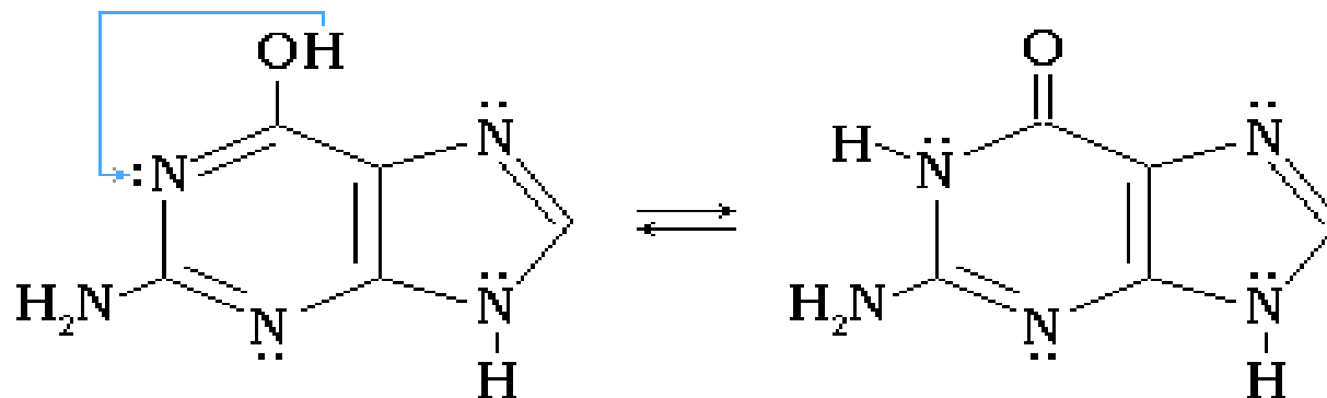
Гуанин (2-амино-6-гидроксипурин)
