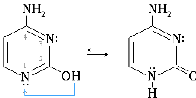
Цитозин (4-амино-2-гидроксипиримидин)
