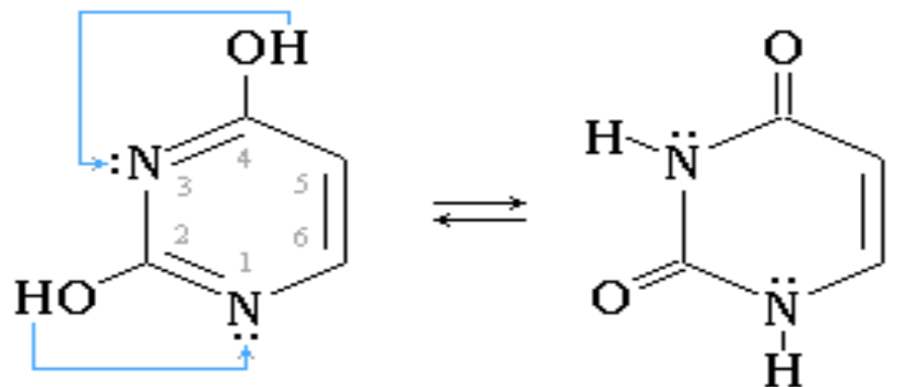
Урацил (2,4-дигидроксипиримидин)
