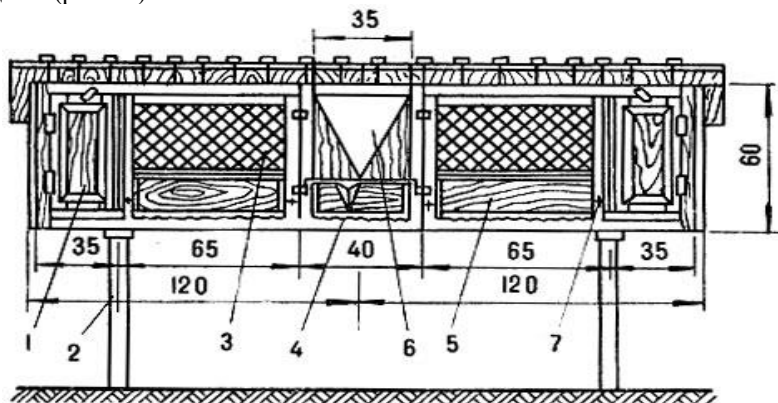
Рис. 67. Двухместная клетка для взрослых кроликов с гнездовым отделением: 1 – дверка в гнездовое отделение; 2 – столб-подставка; 3 – сетчатая дверка; 4 – откидная поилка; 5 – откидная кормушка; 6 – ясли; 7 – ось кормушки
