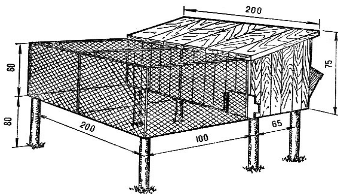
Рис. 68. Двухместная клетка с сетчатым выгулом-вольером
