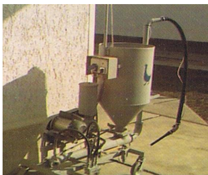
Рис. 36. Машина для принудительного откорма птицы
