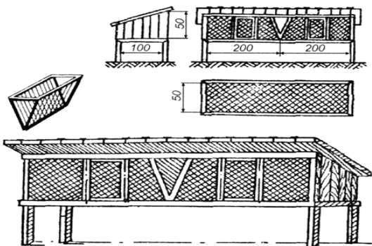
Рис. 69. Групповая клетка для отсаженного молодняка
