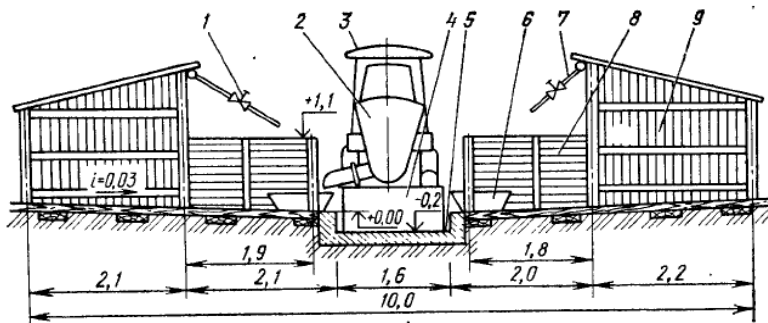
1 – навес для содержания животных; 2 – домик для персонала; 3 – дворовая уборная; 4 – жижеборник; 5 – эстакада для погрузки животных; 6 – дезбарьер; 7 – площадка для навоза; 8 – пожарный резервуар
