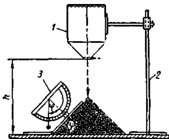
Рисунок 76. Прибор для определения угла естественного откоса зерна при высыпании из воронки: 1 – воронка, 2 – подставка, 3 – линейка с транспортиром и отвесом.
