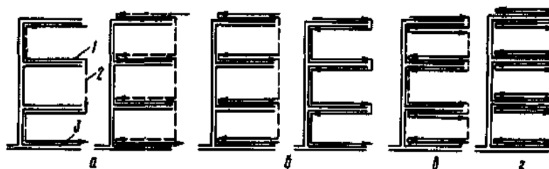
Рис. 11.9. Схемы рабочих перемещений экскаваторов и каналоочистителей: а, б, в, г – соответственно при одном, двух, трех и четырех проходах; 1 и 2 – рабочее и транспортное перемещения; 3 – канал.
