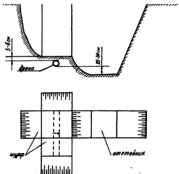
Рис. 11.21. Шурф с отстойником: а – разрез; б – вид сверху; 1 – дрена; 2 – шурф; 3 – отстойник.
