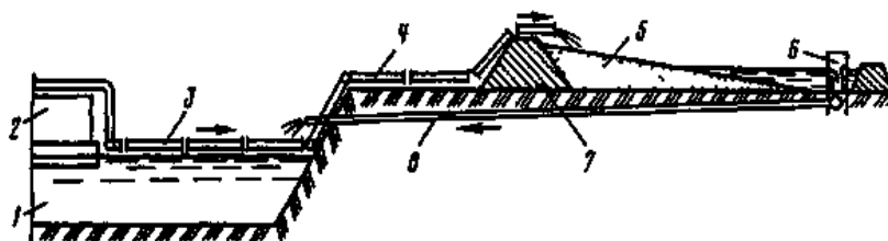
Рис. 11.14. Схема обустройства приканальных площадей при подготовке их для складирования наносов (грунта), удаленных из канала земснарядом: 1 – канал; 2 – земснаряд; 3 и 4 – плавучий и береговой пульпопроводы; 5 – отвал удаленных из канала наносов (грунта); 6 – водосбросной колодец; 7 – дамбы обвалования; 8 – водосбросная труба (лоток).
