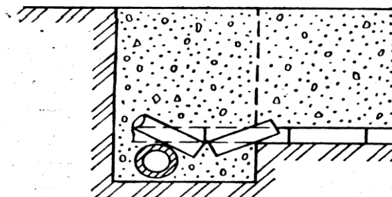
Рис. 10.5. Повреждение сопряжения дрены с коллектором
