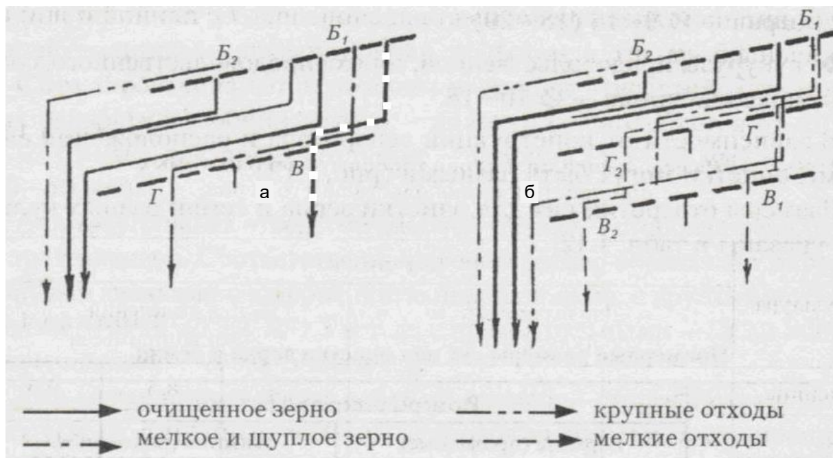
Рисунок 60. Схема расположения решет в зерноочистительных машинах: а – первичная очистка; б – вторичная очистка
