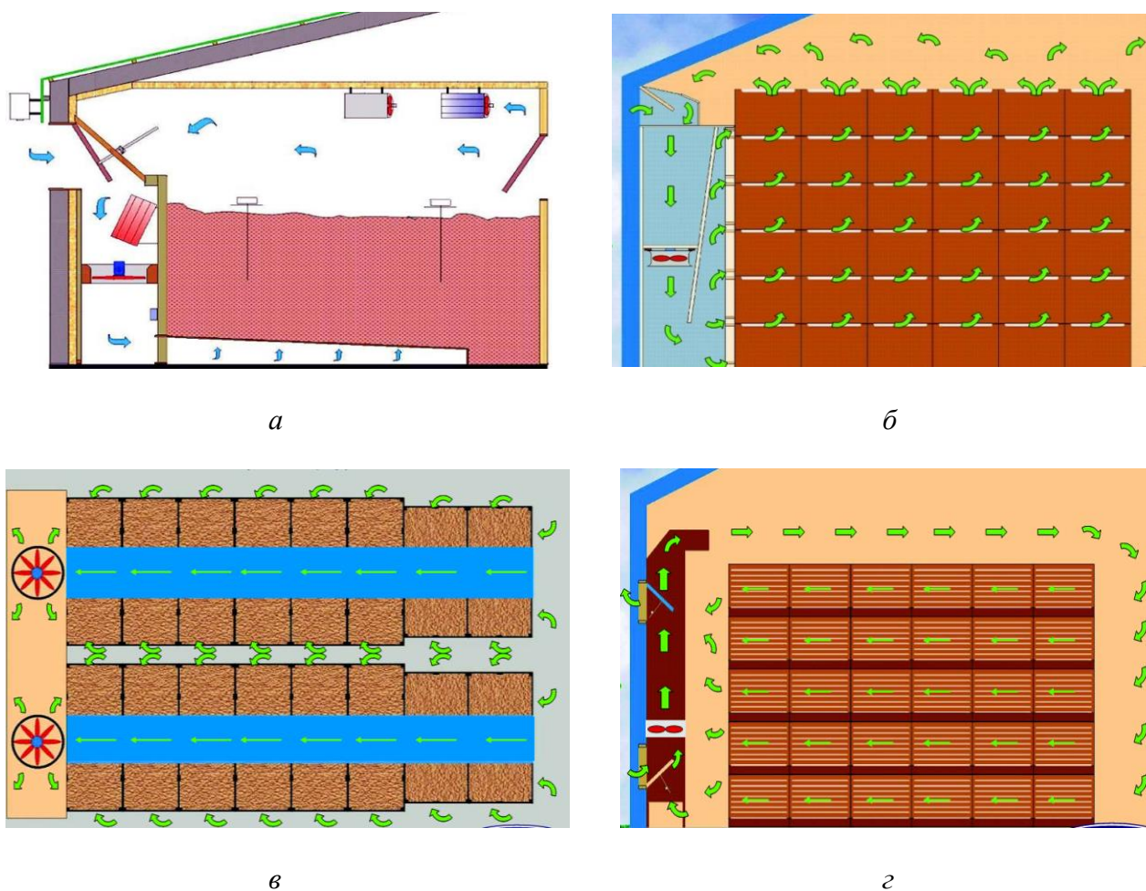
Рис. 6. Системы активной вентиляции хранилищ: а – напольные каналы (при навалном хранении); б – стена давления; в – система всасывания (вид сверху); г – объемное вентилирование
