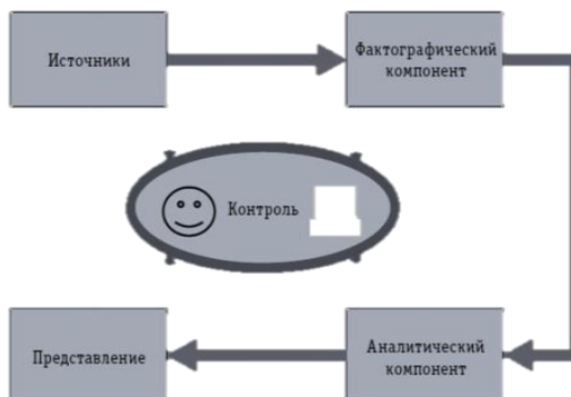
Рис. 11.4. Функциональная схема факто-аналитической программной системы
