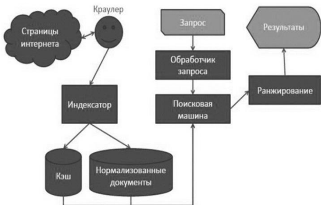
Рис. 11.2. Общая структура системы информационного поиска
