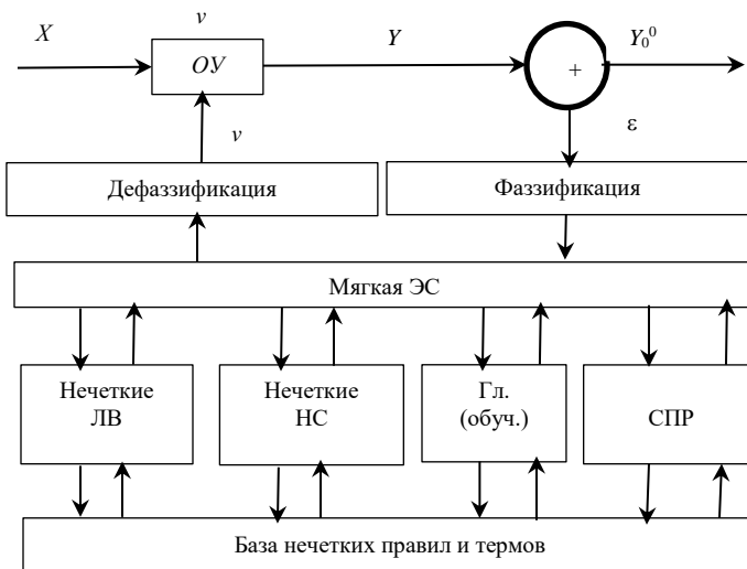
Рис. 10.3. Мягкая экспертная система
