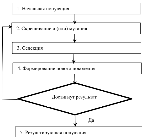
Рис. 14.3. Алгоритм эволюции
