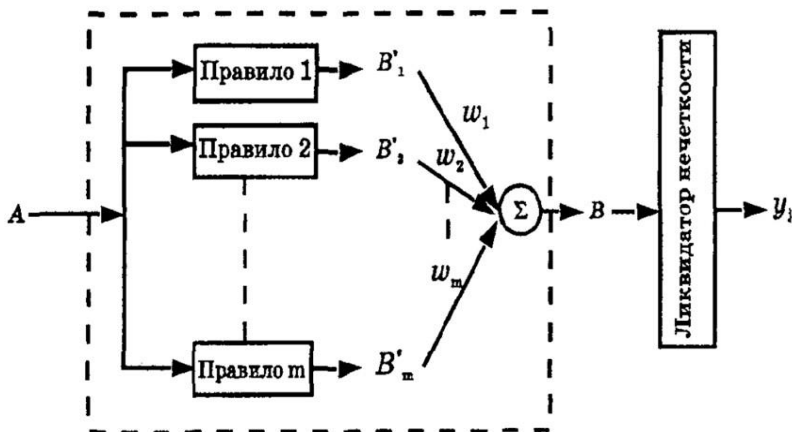
Рис. 8.2. Архитектура системы нечетких правил
