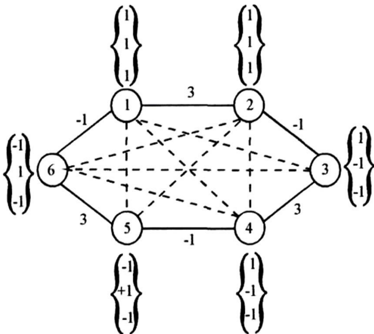
Рис. 5.2. Нейронная сеть Хопфилда
