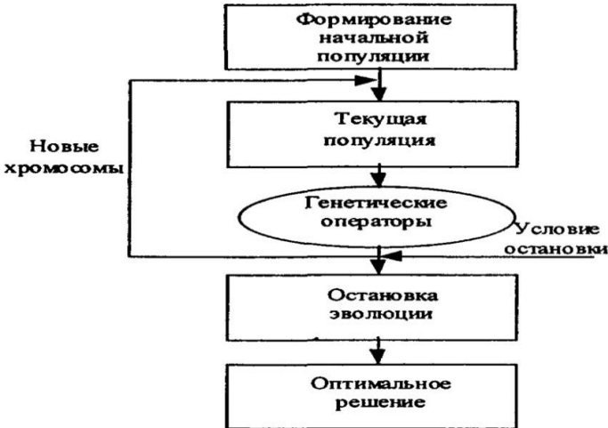
Рис. 9.2. Генетический алгоритм
