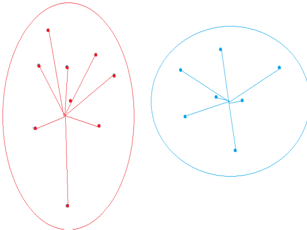
Рис. 7.4. Метод Варда
