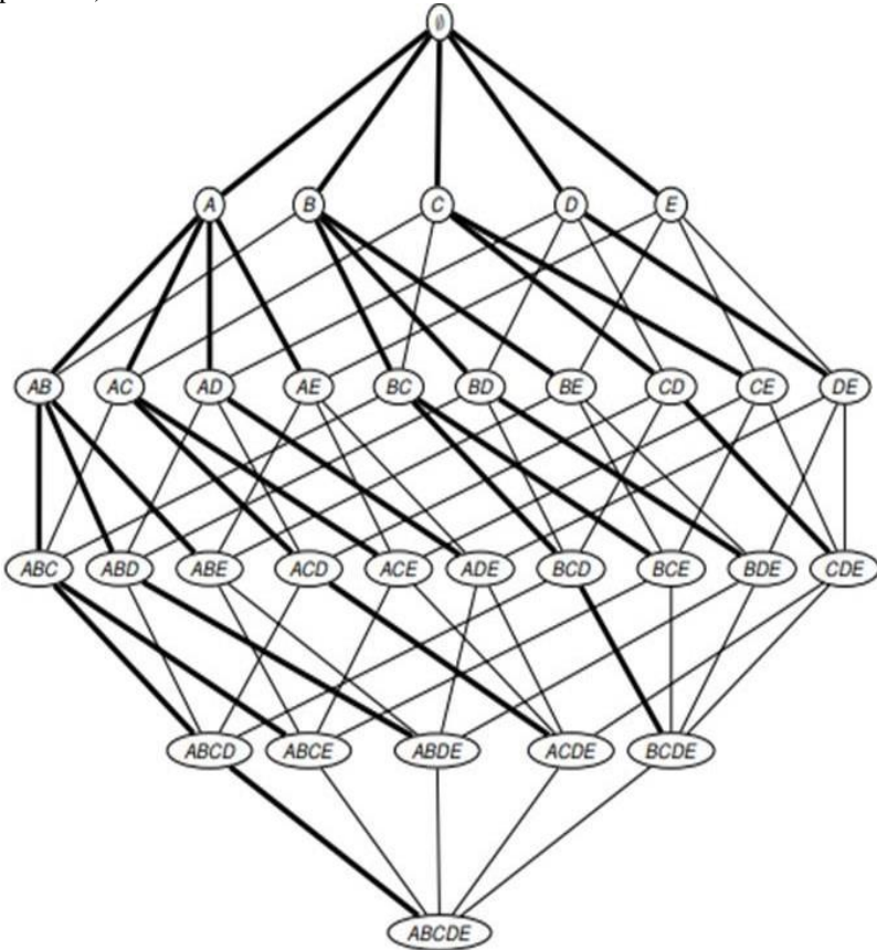
Рис. 8.1. Алгоритм Apriori
