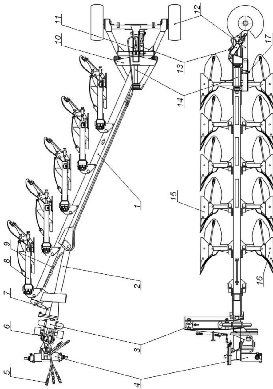
Рис. 6. Плуг пятикорпусный полунавесной оборотный ППО-5-40: 1 – рама; 2 – балка тяговая; 3 – механизм оборота рамы; 4 – навеска; 5 – гидросистема; 6 – фиксатор; 7 – галтель; 8 – предохранитель; 9 – трубопровод; 10 – цилиндр; 11 – ход колесный; 12 – ход колесный; 13 – механизм регулировки глубины вспашки задними корпусами; 14 – ось; 15 – корпус левооборачивающий; 16 – корпус правооборачивающий; 17 – болт регулировочный
