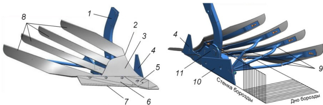
Рис. 2. Корпус плуга в сборе со стойкой: 1 – стойка; 2 – полевой обреза; 3 – грудь отвала; 4 – нож полевой доски; 5 – долото; 6 – лемех; 7 – лезвие лемеха; 8 – пластины отвала; 9 – распорки; 10 – полевая доска; 11 – башмак
