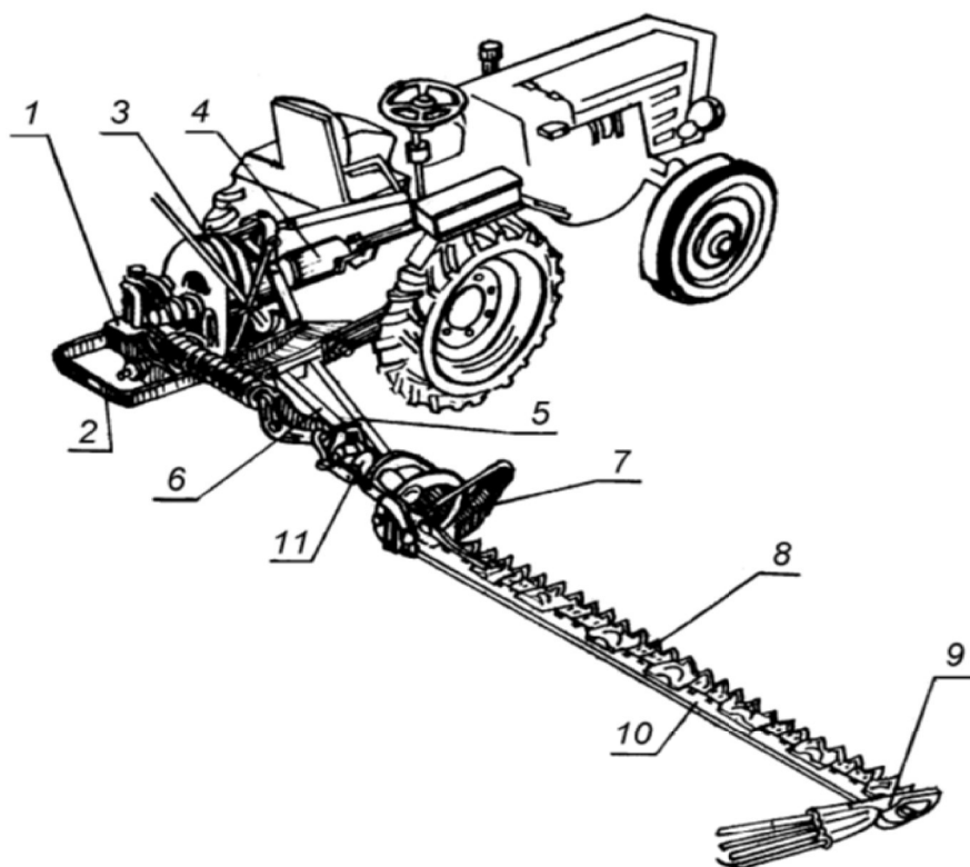
Рис. 1. Общий вид косилки КС-2,1:
