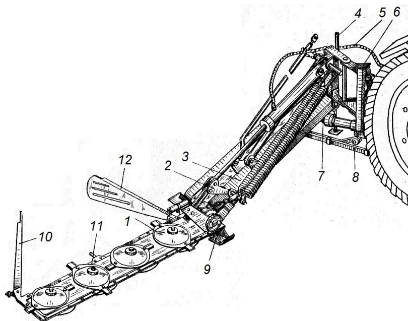
Рис. 8. Общий вид косилки КДН-210:
