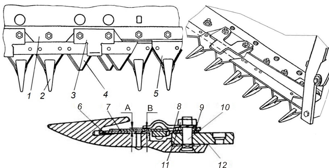
Рис. 6. Сегментно-пальцевый режущий аппарат косилки КПП-4,2: 1 – пальцевый брус; 2 – палец; 3 – прижим; 4 – правый нож; 5 – левый нож; 6 – противорежущая пластина; 7 – сегмент; 8 – пластина трения; 9, 12 – регулировочные прокладки; 10 – болт; 11 – гайка; А – зазор между сегментом и прижимом; В – зазор между сегментом и противорежущей пластиной
