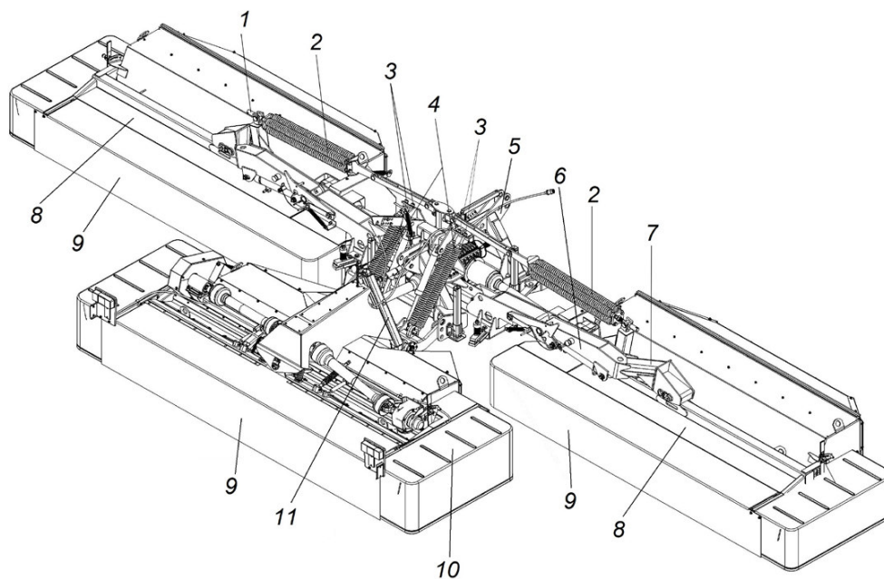
Рис. 11. Общий вид косилки КПр-9:
