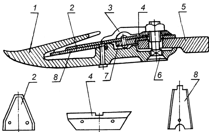
Рис. 2. Режущий аппарат косилки КС-2,1:
