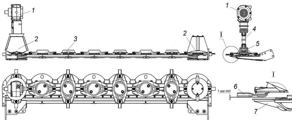
Рис. 13. Режущий брус:
