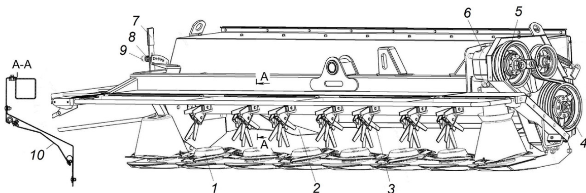
Рис. 12. Боковая секция:
