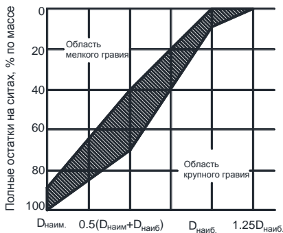
Рис. 6.3. График зернового состава щебня (гравия)
