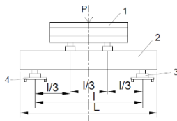
Рис. 7.4. Схема испытания бетонных образцов на растяжение при изгибе: 1 – траверса; 2 – испытательная призма; 3 – неподвижная опора; 4 – подвижная опора
