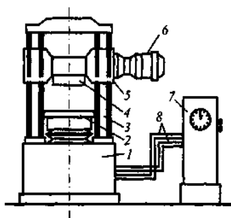
Рис. 4.16. Гидравлический пресс: 1 – чугунная станина; 2 – нижняя опора; 3 – стальные колонны; 4 – верхняя опорная плита; 5 – траверса; 6 – образец; 7 – электродвигатель; 8 – пульт управления; 8 – маслопроводы
