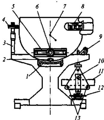
Рис. 4.15. Испытательная машина МИИ-100: 1 – шкала; 2 – стрелка; 3 – амортизатор; 4 – шайба; 5 – прорезь; 6 – груз; 7 – рукоятка управления; 8 – счётчик; 9 – коромысло; 10 – валик; 11 – образец балочка; 12 – маховичок; 13 – опоры
