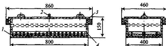
Рис. 4.5. Ванна с гидравлическим затвором: 1 – ванна; 2 – пробка; 3 – гидравлический затвор; 4 – решётка для образцов
