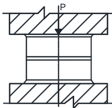
Рис. 2.3. Схема испытания кирпича на сжатие
