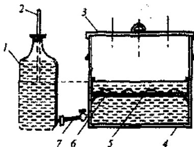
Рис. 4.6. Пропарочный бачок: 1 – сосуд с водой; 2 – подвижная линейка для регулирования уровня воды в бачке; 3 – крышка; – бачок; 5 – съёмная решётка; 6 – лепёшки из цементного теста; 7 – резиновая трубка
