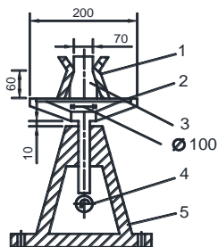
Рис. 4.11. Встряхивающий столик и форма-конус: 1 – форма; 2 – стекло; 3 – ось с горизонтальным диском; 4 – кулачок; 5 – чугунная станина
