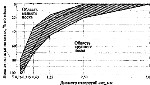
Рис. 6.1. График зернового состава песка
