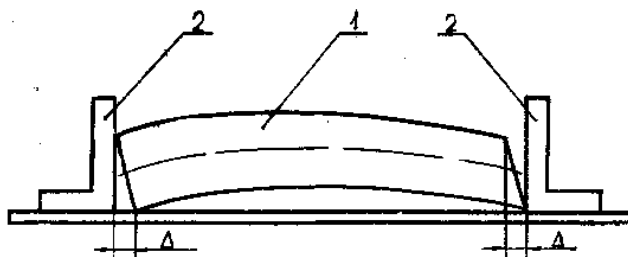
Рис. 3.2. Измерение искривления поверхности трубы: 1 – труба; 2 – угольник
