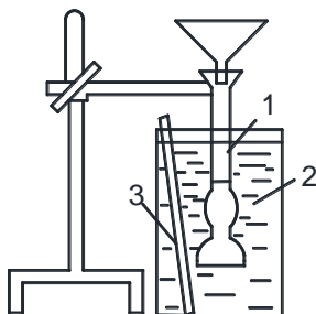
Рис. 1.1. Объеммер Ле Шателье: 1 – объеммер; 2 – сосуд с водой; 3 – термометр
