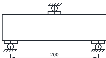
Рис. 2.4. Схема испытания кирпича на изгиб
