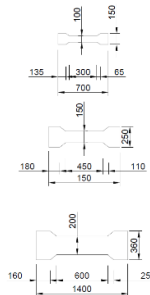
Рис. 7.3. Образцы-восьмёрки
