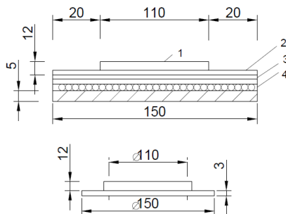
Рис. 8.2. Схема прибора для определения водоудерживающей способности растворной смеси: 1 – металлическое кольцо с раствором; 2 – слой марлевой ткани; 3 – 10 слоев промокающей бумаги; 4 – стеклянная пластинка
