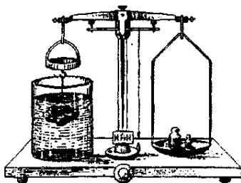
Рис. 1.4. Взвешивание образца на гидростатических весах
