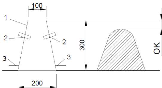
Рис. 7.1. Схема определения подвижности бетонной смеси: 1 – конус; 2 – ручки; 3 – опоры; 4 – осадка конуса
