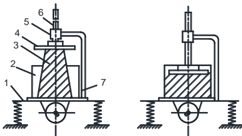
Рис. 7.2. Схема определения жёсткой бетонной смеси: a – прибор в исходном состоянии ( 1 – виброплощадка; 2 – цилиндр; 3 – конус с бетонной смесью; 4 – диск с отверстиями; 5 – втулка; 6 – штанга); б – прибор после окончания вибрирования
