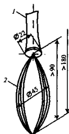
Рис. 5.2. Ручная мешалка: 1 – ручка; 2 – петли
