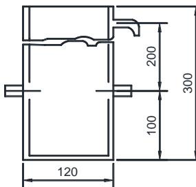
Рис. 6.2. Сосуд для отмучивания песка
