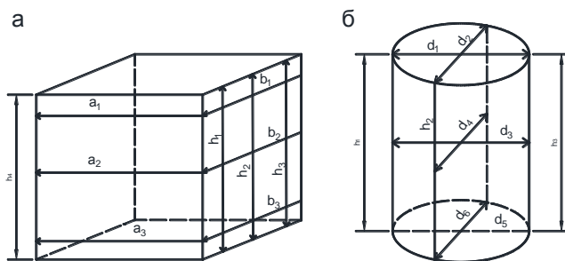
Рис. 1.2. Схемы измерения объема образца: а – кубической формы; б – цилиндрической формы
