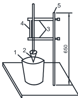
Рис. 8.1. Прибор для определения подвижности растворной смеси: 1 – ведро; 2 – конус; 3 – кронштейн; 4 – линейка; 5 – стойка
