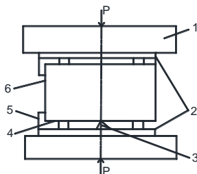
Рис. 2.2. Схема раскалывания кирпича на прессе: 1 – плита прессы; 2 – основание; 3 – металлический нож; 4 – резиновые прокладки; 5 – упор; 6 – образец
