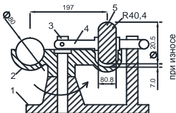
Рис. 4.10. Лабораторная мешалка: 1 – станина; 2 – смесительная чаша; 3 – ось чаши; 4 – откидная траверса; 5 – валик для перемешивания раствора
