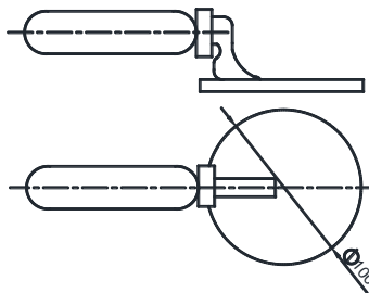
Рис. 4.4. Стандартная лопатка цемента и гипса
