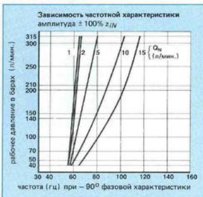
Рис. 29: Зависимость фазовой характеристики (амплитуда \pm 100\% z_{1N} )
