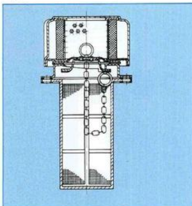
Рис. 26: Заправочный и вентиляционный фильтр в разрезе
