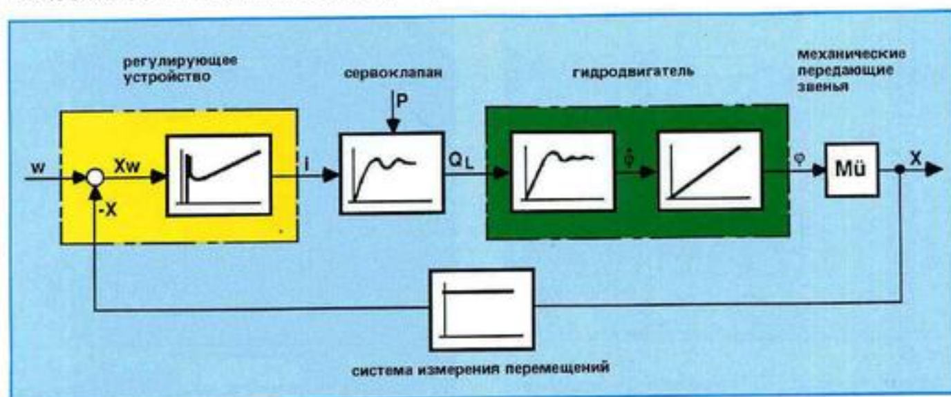
Рис. 50: Блок-схема регулируемого по положению электропривода
