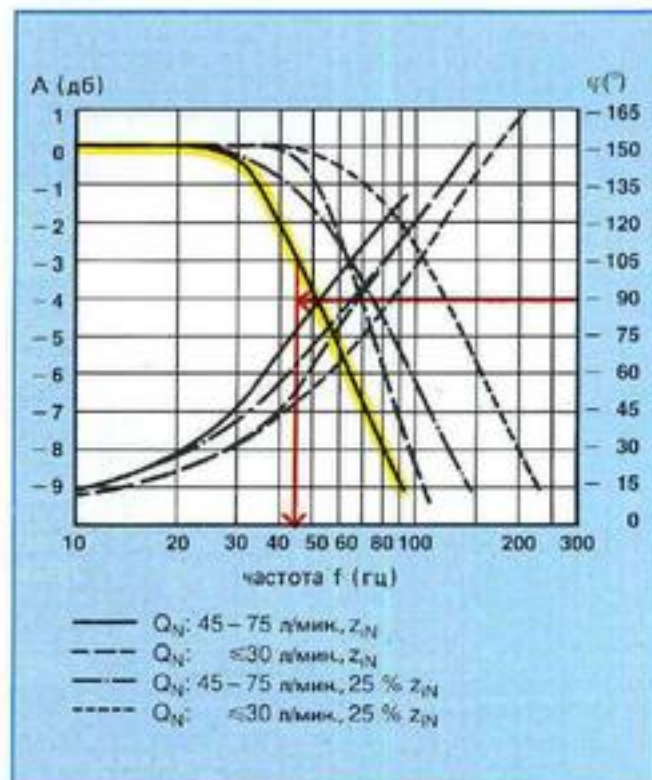
Рис. 17: Типичное изображение частотной характеристики для сервораспределителей с механич. обратной связью
