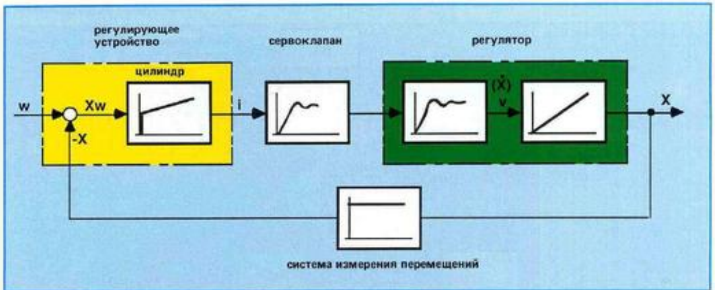
Рис. 51: Блок-схема регулируемого по положению привода цилиндра
