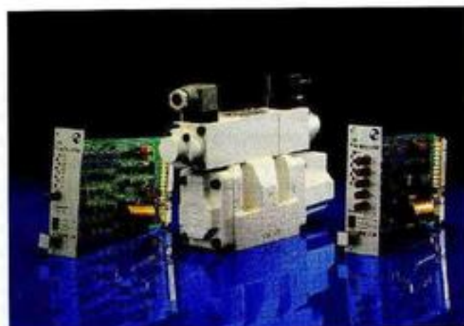
Рис. 31: Пропорциональный распределитель непрямого действия типа 4WRZ, электроника управления
