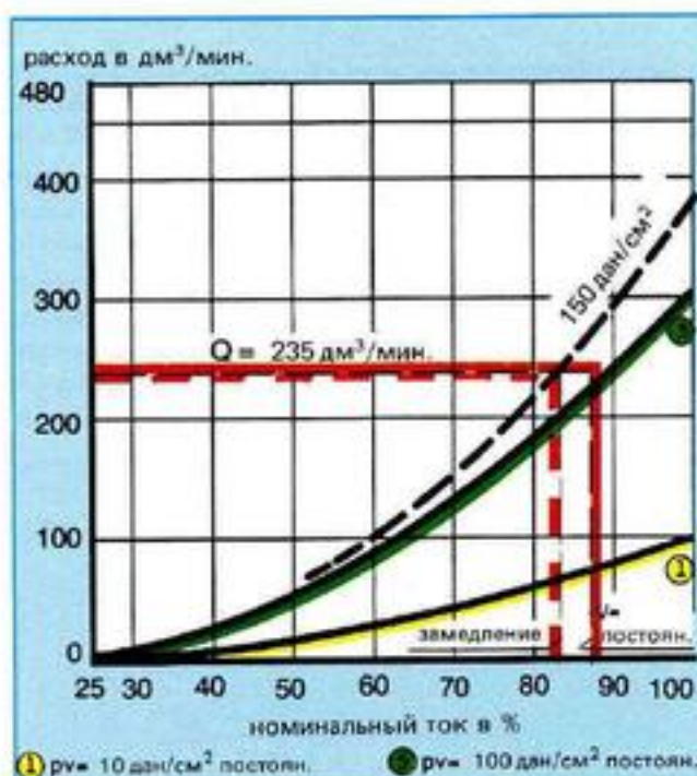
Рис. 14: График характеристика Q - I для номинального расхода в 100 \text{ дм}^3/\text{мин.} при потере давл. клап. в 10 \text{ дн}/\text{см}^2
