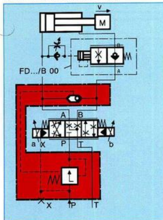
Рис. 13: Тормозной клапан как подпора
