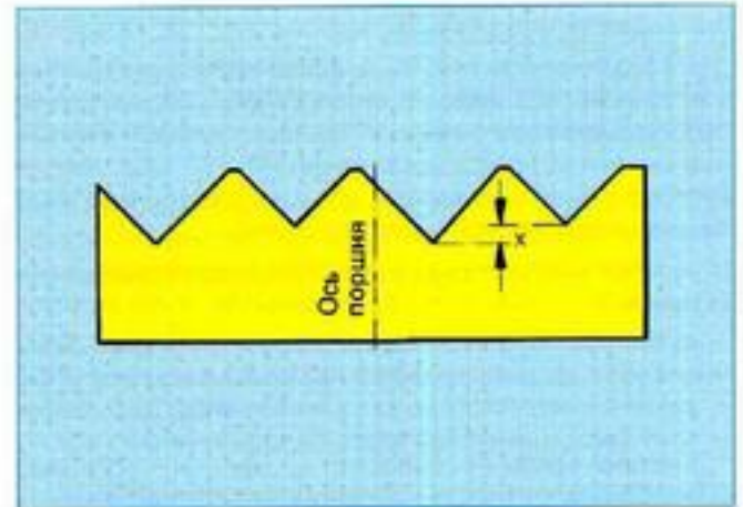
Рис. 10: Смещенные дросселирующие пазы по окружности поршня и длинный ход поршня обеспечивают хорошую разрешающую способность
