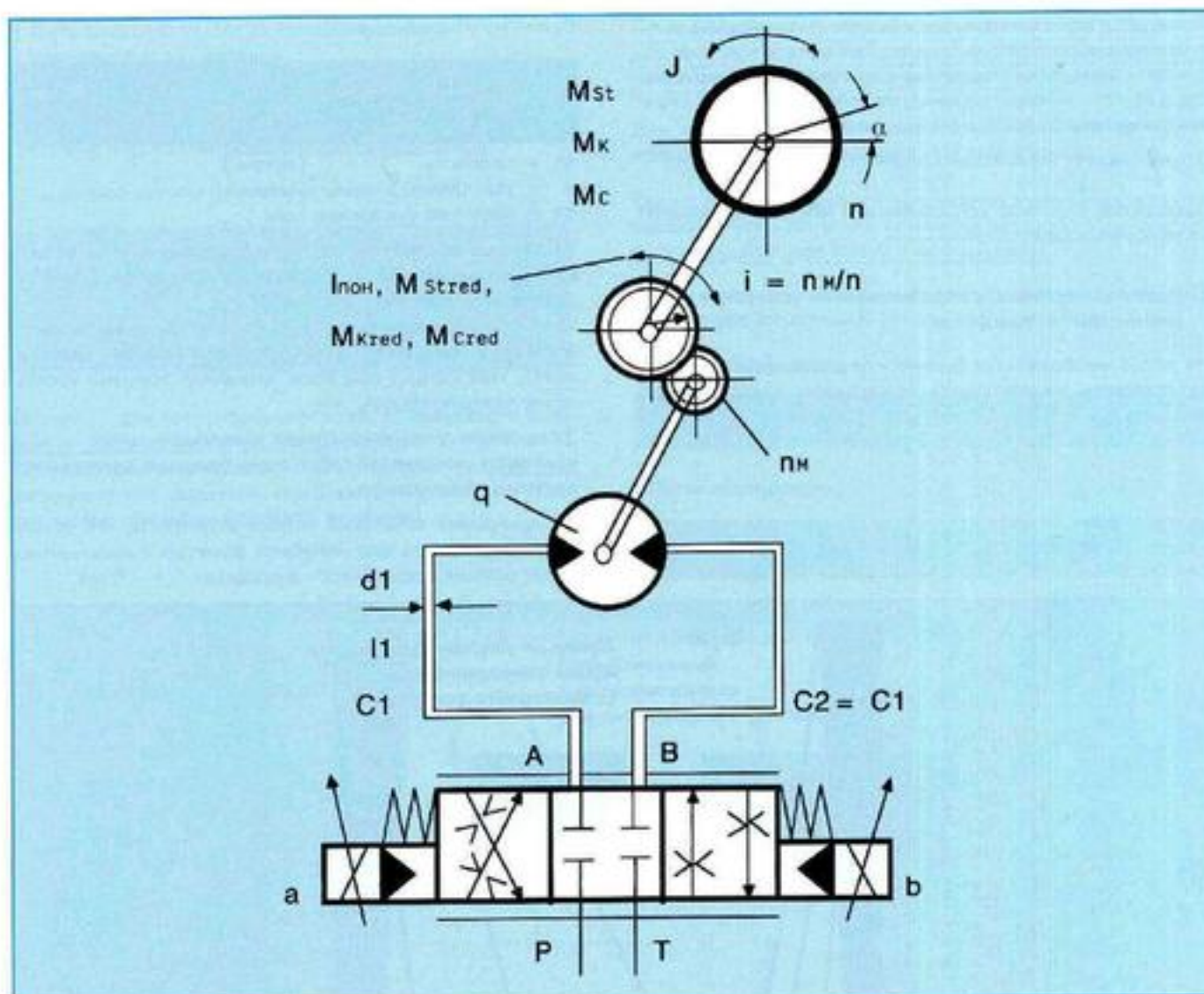
Рис. 5: Приводы двигателем вращательного движения
