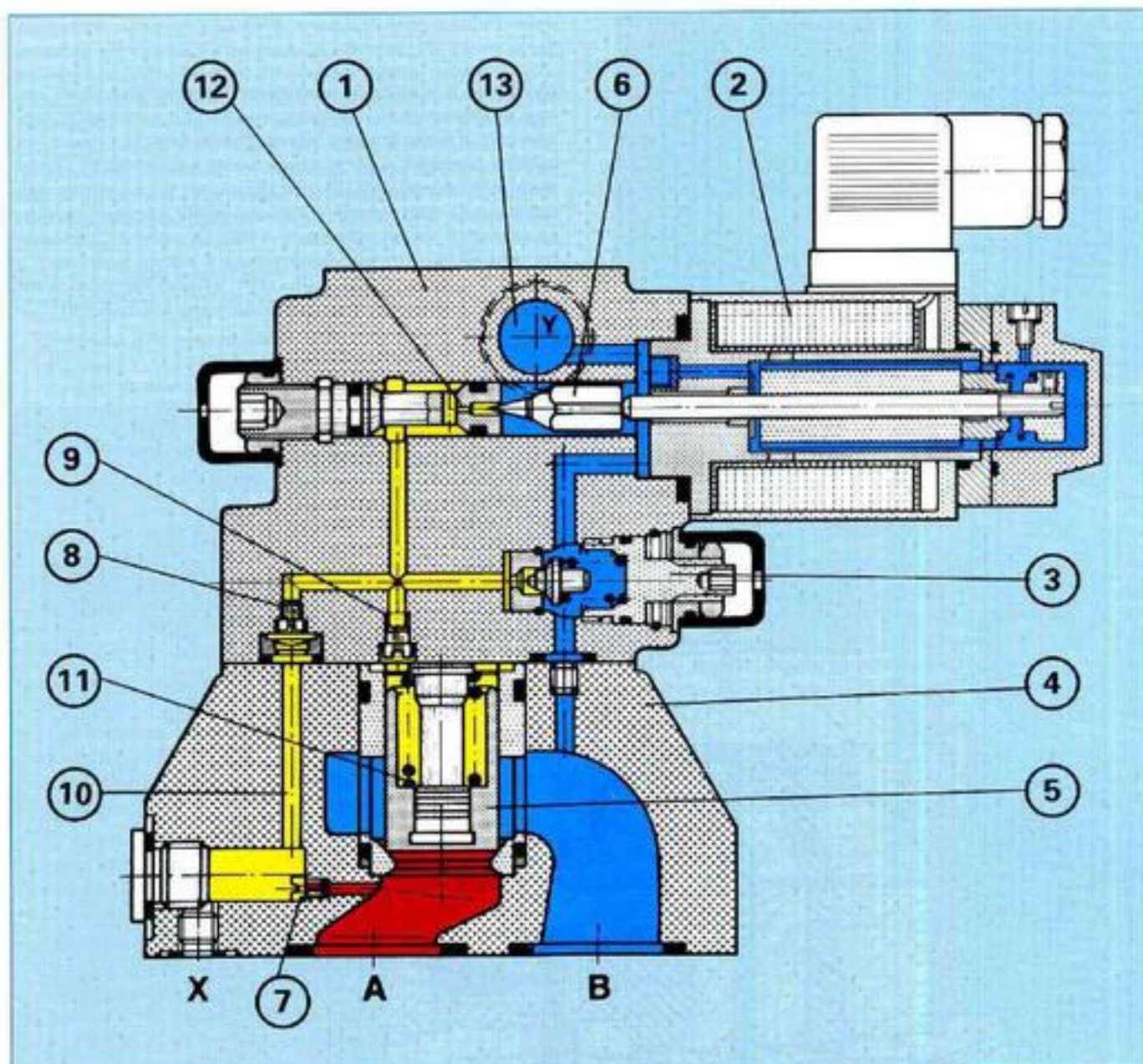
Рис. 44: Пропорциональный клапан для ограничения давления непрямого действия с предохранительным устройством от максимального давления типа DBEM
