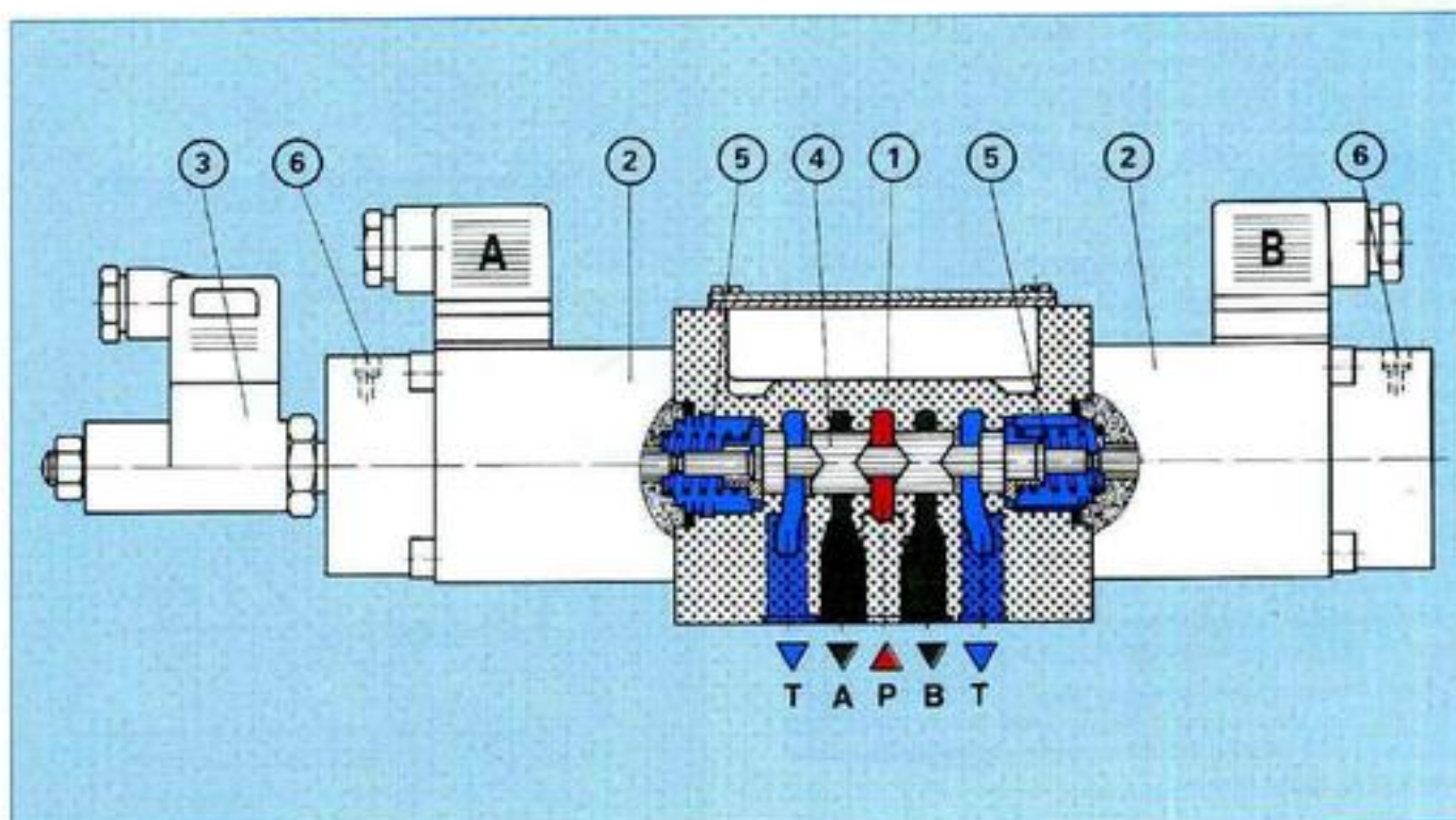
Рис. 6: Пропорциональный распределитель прямого действия с электрической обратной связью
