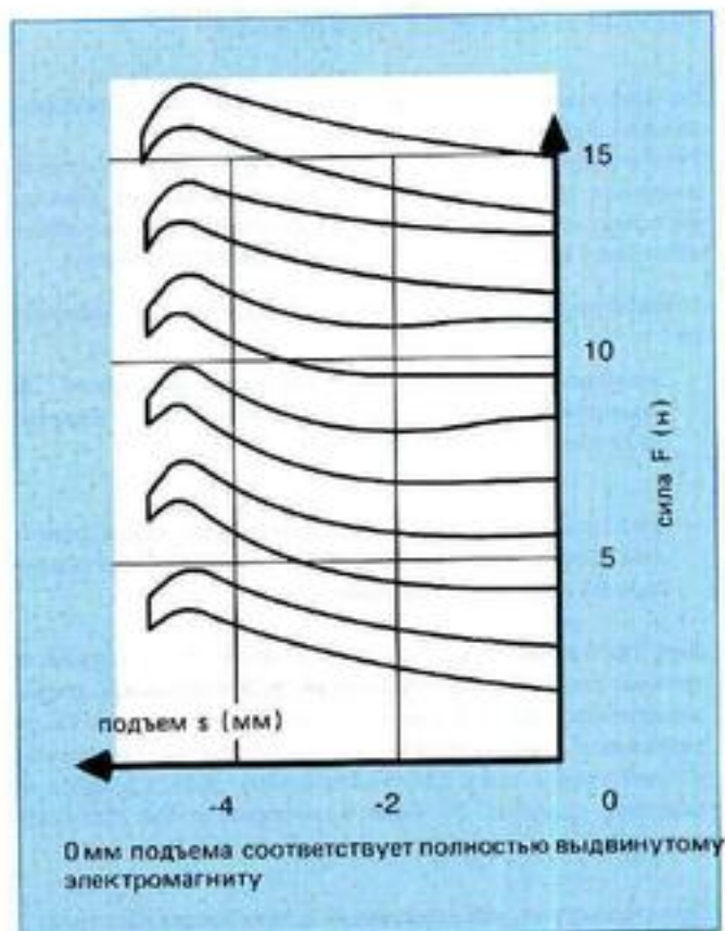
Рис. 3: Графическая характеристика, электромагнит, регулируемый по подъему
