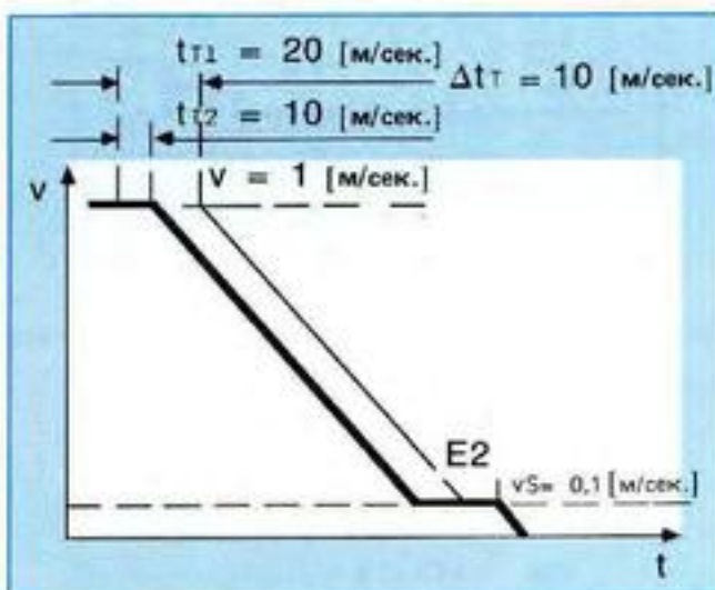
Рис. 20: Путь замедления при изменении времени запаздывания
