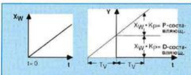
Рис. 47а: Характеристика PD-T1-регулятор
