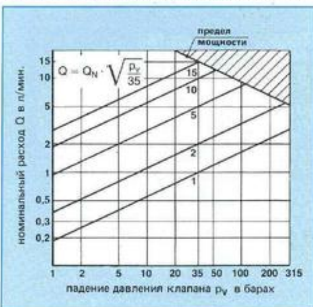
Рис. 28: Расходная характеристика при наличии нагрузки при z_{1N} (выше предела мощности зависимость между Q и p_v будет негативной)
