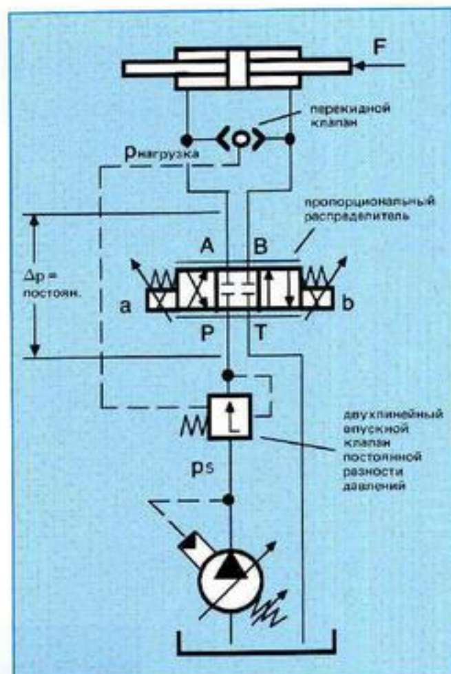
Рис. 2: Пример переключения
