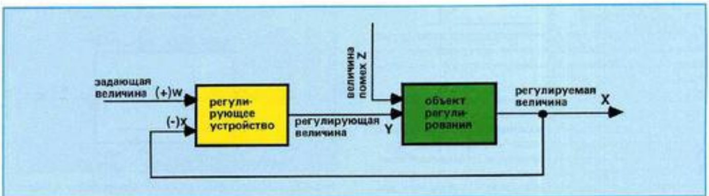
Рис. 11: Принципиальная схема соединений контура регулирования
