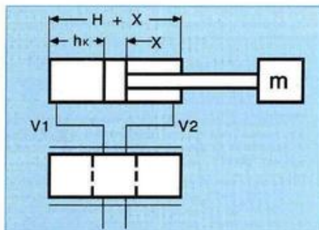
Рис. 7: Определение собственной частоты посредством дифференциального цилиндра
