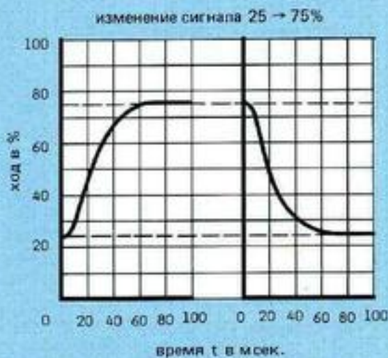
Рис. 15: Переходная функция при скачкообразном, электрическом, входном сигнале, изменение сигнала 25 → 75%
