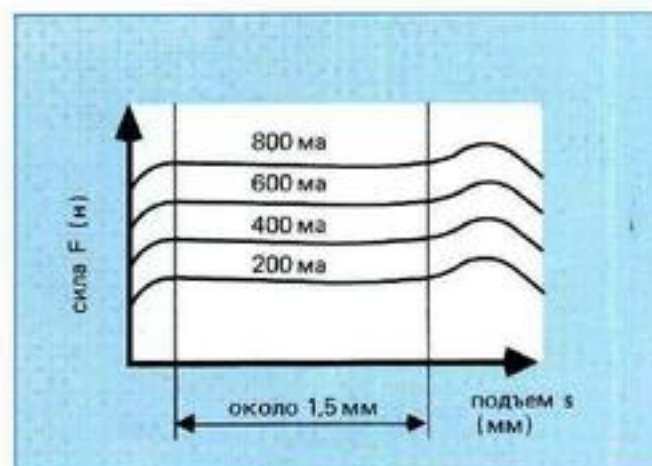
Рис. 2: Графическая характеристика "сила - подъем"
