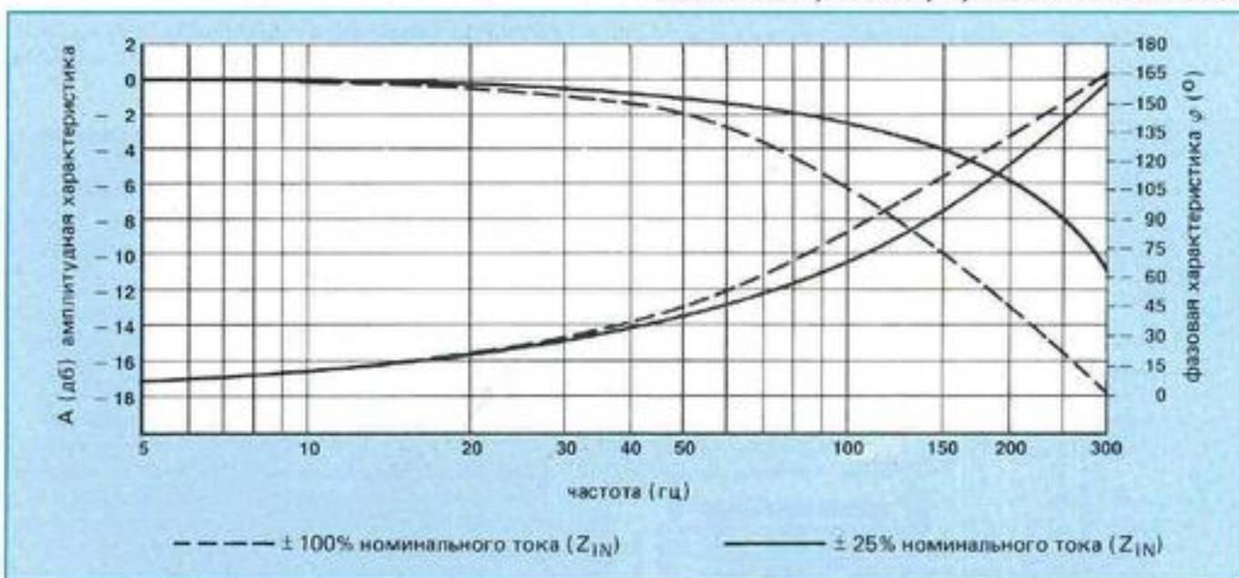
Рис. 27: типичное изображение фазовой характеристики при p = 315 бар и Q_N = 15 л/мин.
