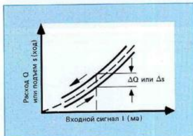
Рис. 8: Гистерезис
