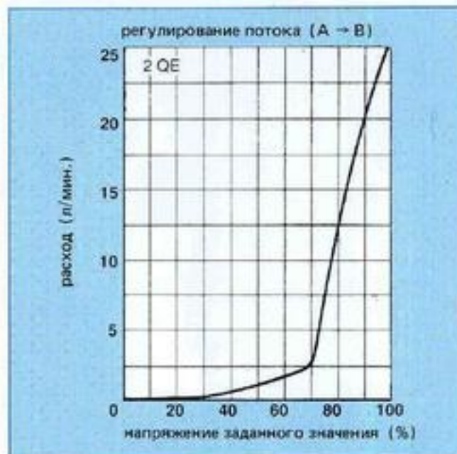
Рис. 54: Зависимость расхода от напряжения заданного значения при клапанах с прогрессивной характеристикой и скачком ускоренного хода
