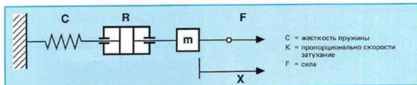
Рис. 29: Пример для P-T 2 -звена
