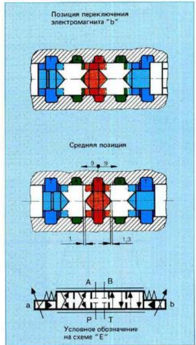
Рис. 12: Перекрывание пропорционального распределителя ДУ25, условное обозначение на схеме "Е" (закрытая средняя позиция)
