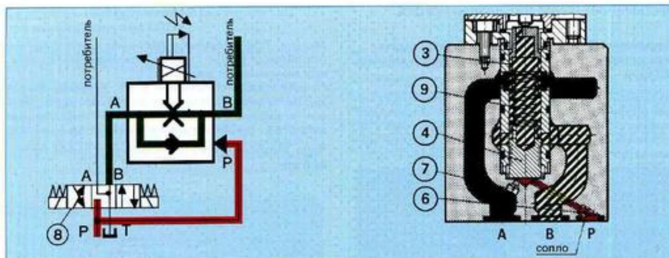
Рис. 52: Внешнее запертие клапана постоянной разности давлений
