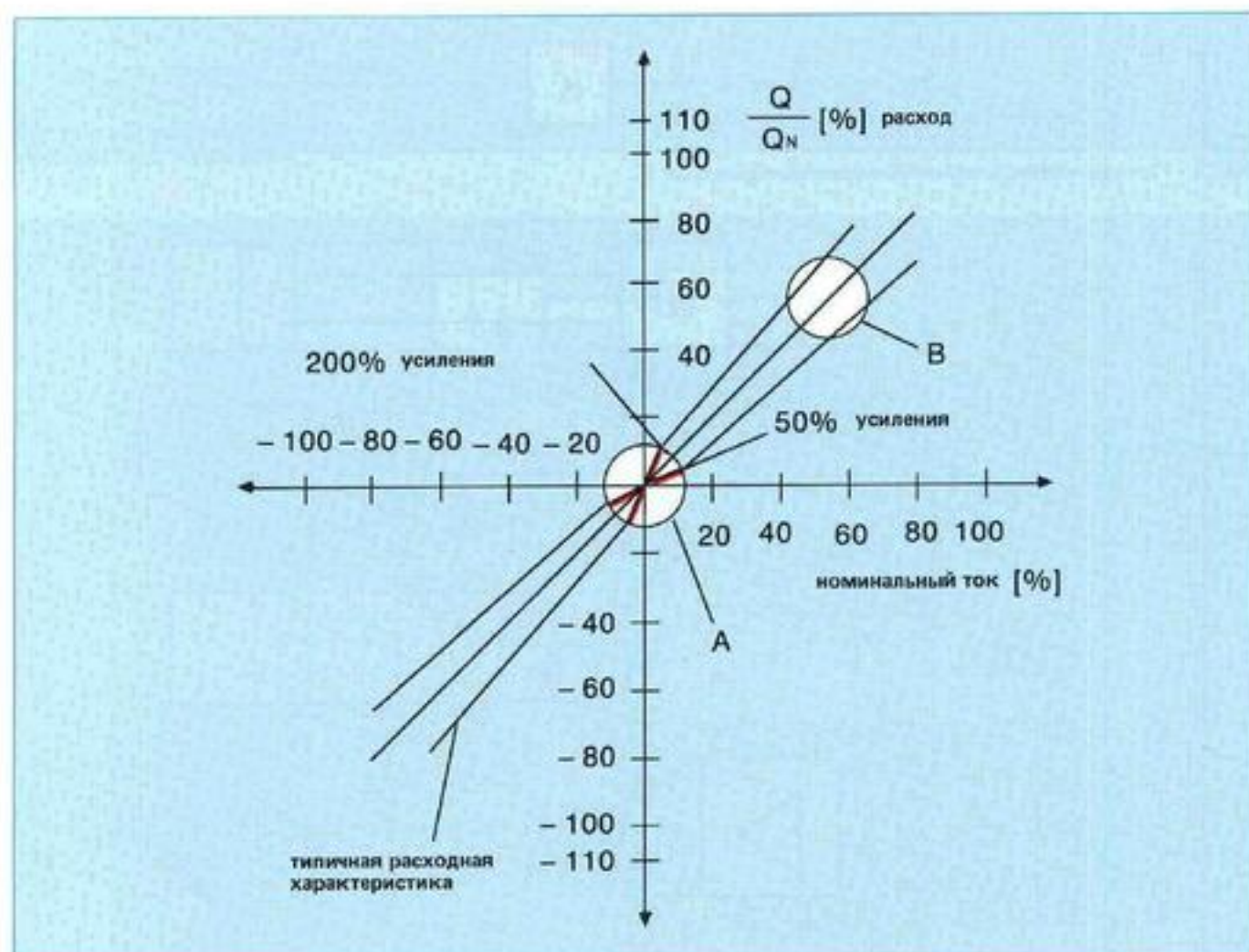
Рис. 5: Расходная характеристика
