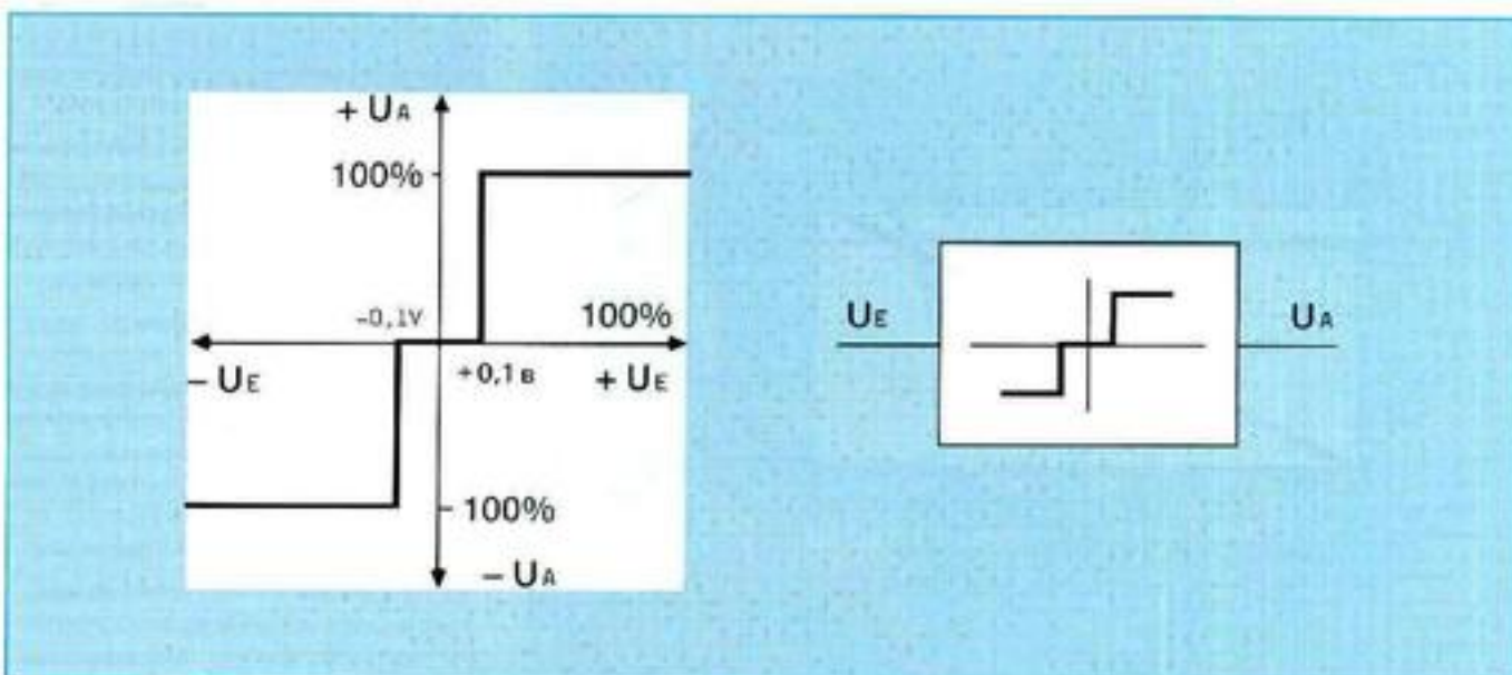
Рис. 9: Образователь скачкообразной функции
