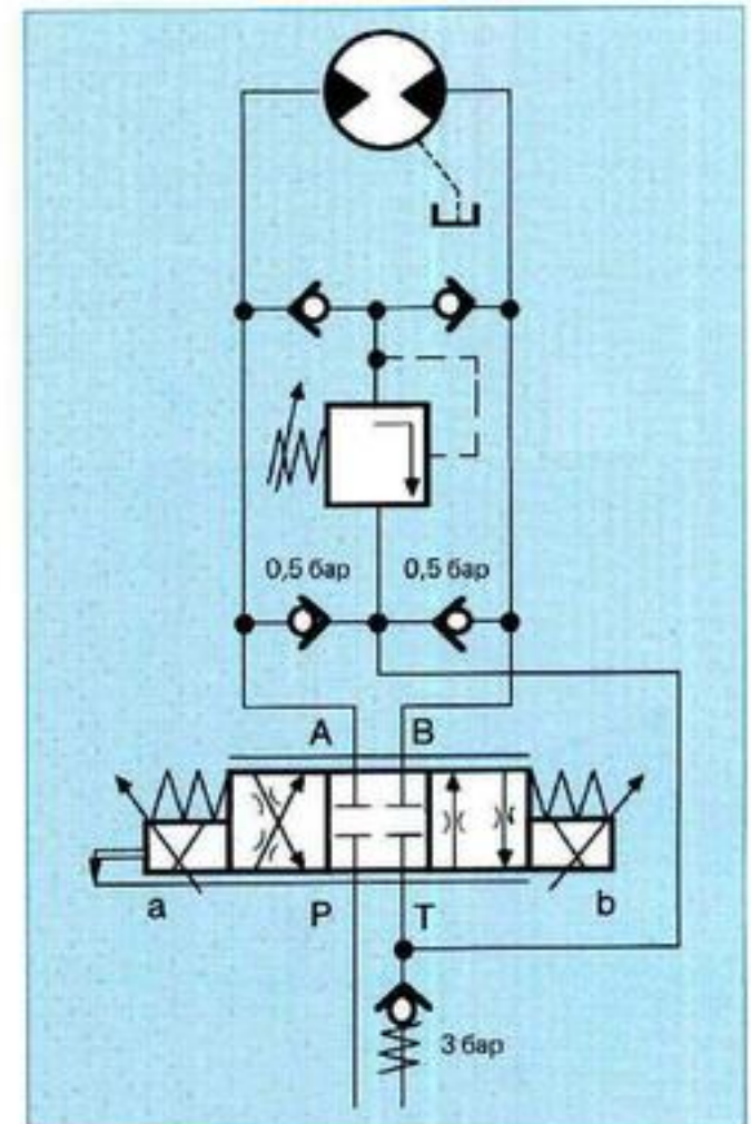
Рис. 20: Поршень E с гидродвигателем
