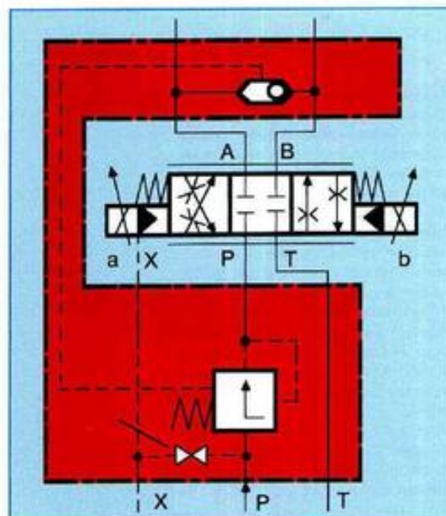
Рис. 8б: Пропорциональный распределитель непрямого действия 4WRZ с впускным клапаном постоянной разности давлений ZDC — впуск управляющего масла снаружи — исполнение в промежуточной плите
