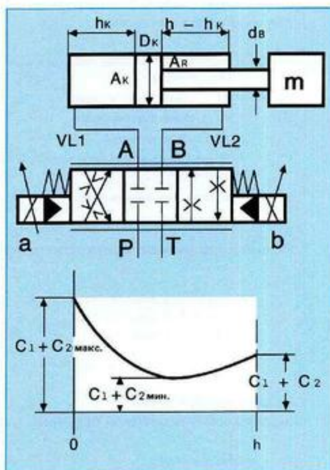
Рис. 25: Дифференциальный цилиндр
