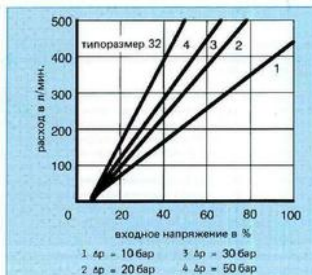
Рис. 59: Расходная характеристика, линейная
