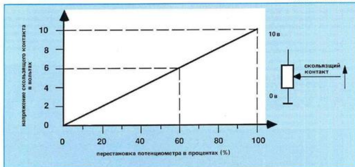
Рис. 84: Потенциометр
