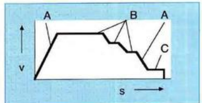
Рис. 38: Диаграмма "скорость - перемещение"
