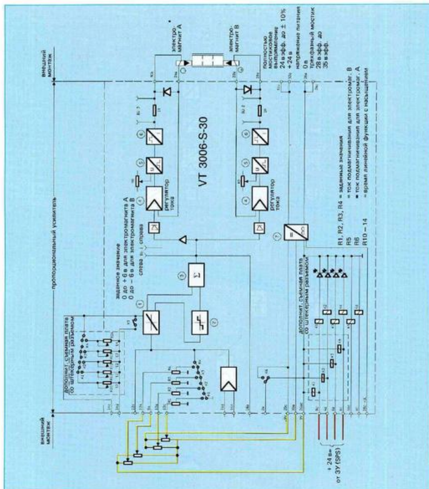
Рис. 25: Монтажная схема соединений
