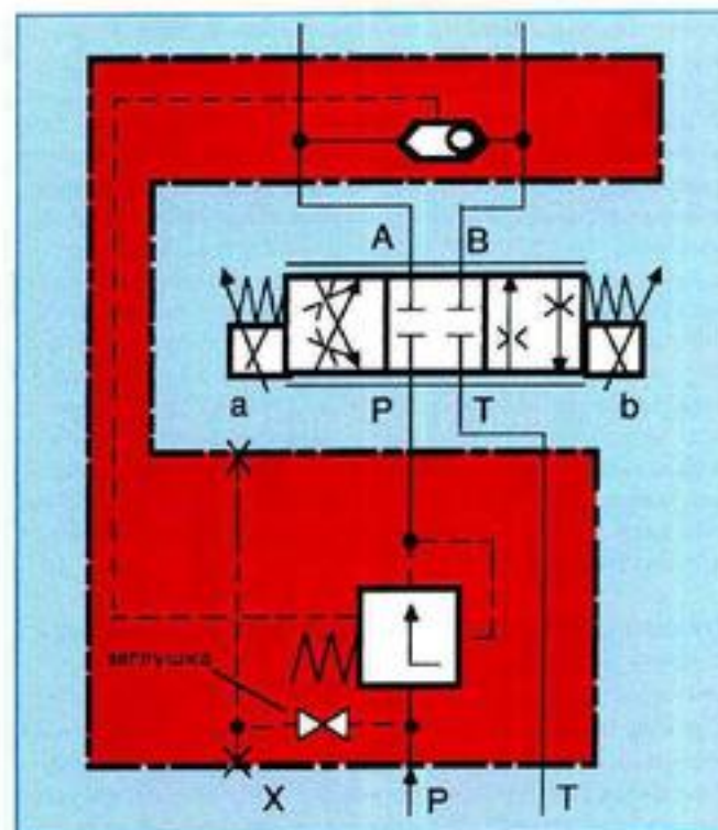
Рис. 8а: Пропорциональный распределитель прямого действия 4WRE с впускным клапаном постоянной разности давлений ZDC — впуск управляющего масла снаружи — исполнение в промежуточной плите
