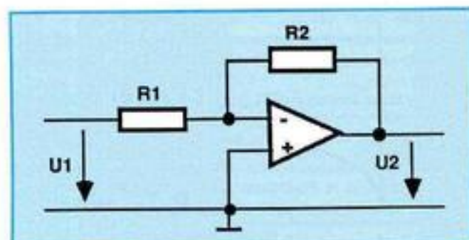
Рис. 17: Усилитель с монтажом на сопротивлениях
