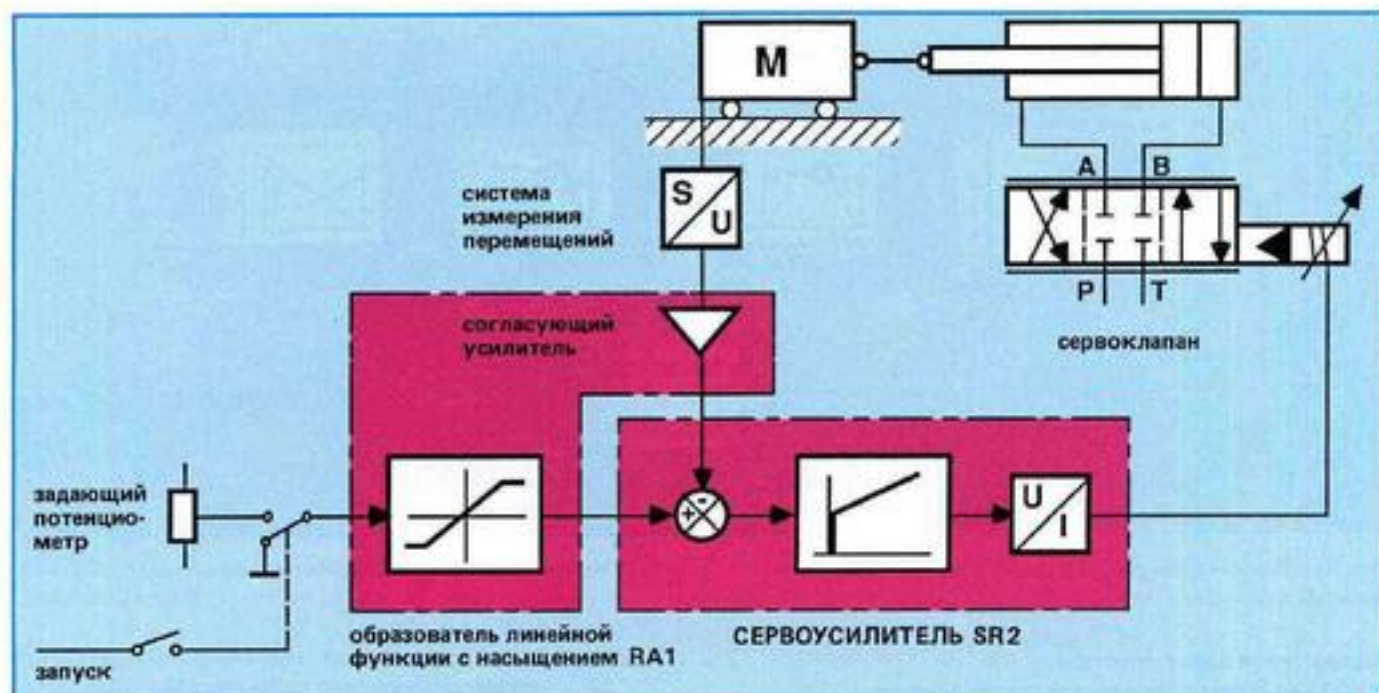
Рис. 52: Пример контура регулирования по положению
