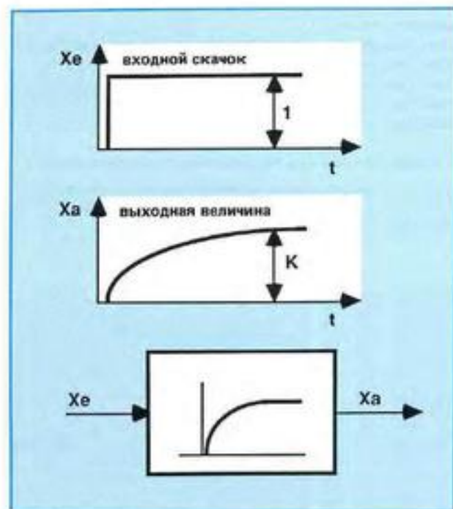
Рис. 13: Пример характеристики переходного процесса
