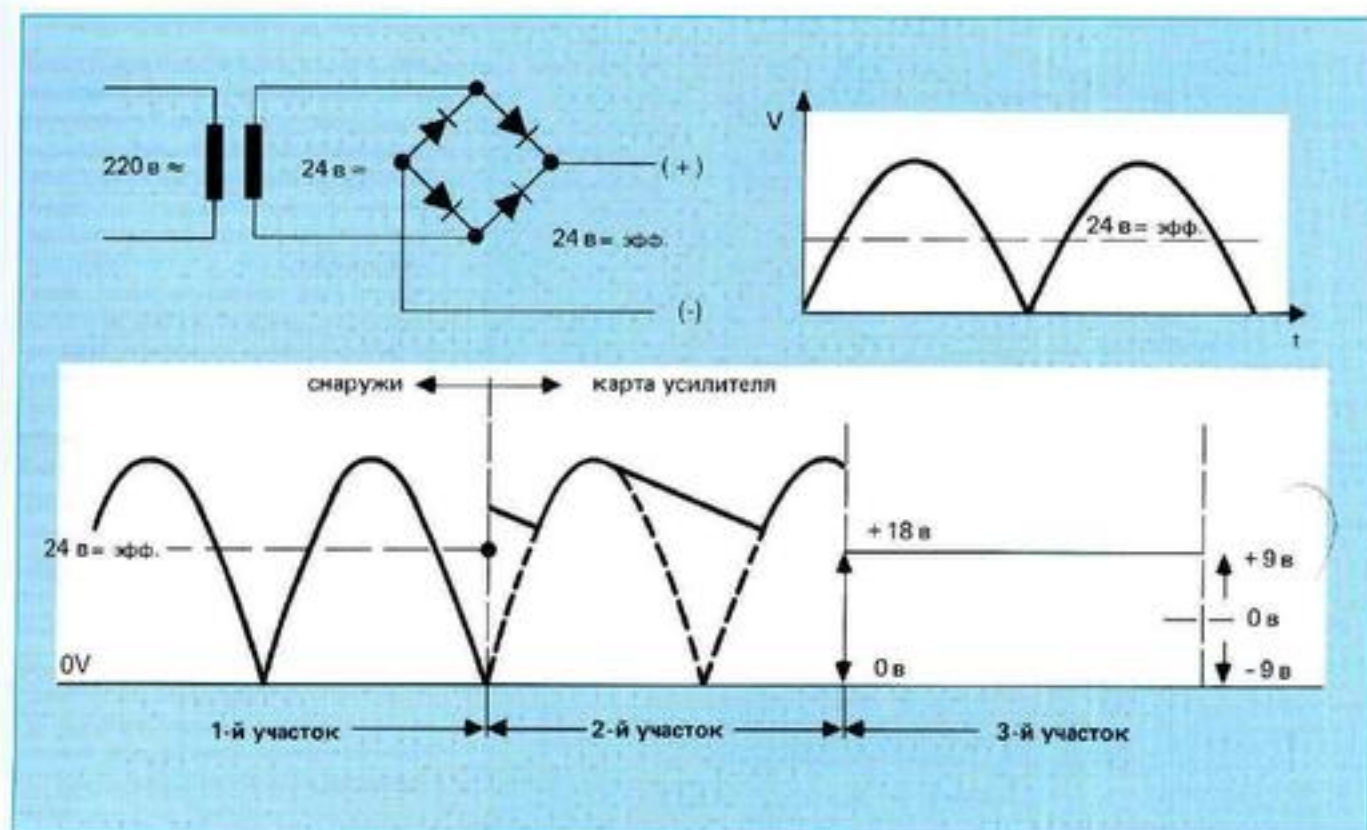
Рис. 8: Однофазное двухполупериодное выпрямление
