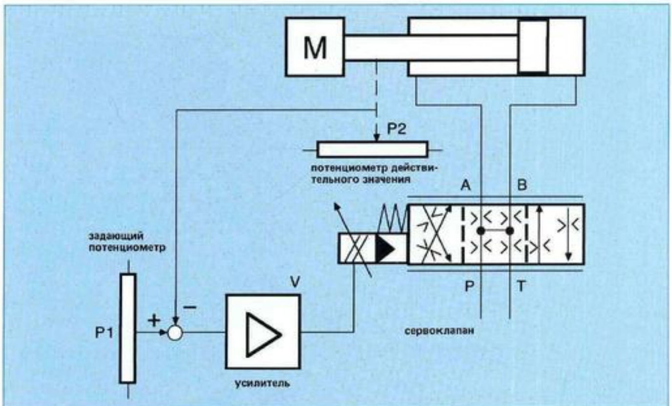
Рис. 4: Контур регулирования с помощью сервоклапана
