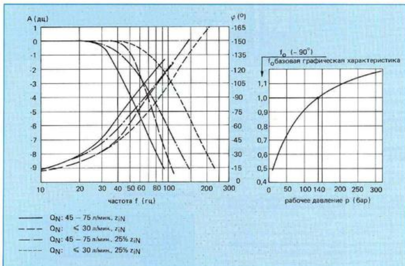
Рис. 10: Типичное изображение базовой частотной характеристики (слева) и зависимость частоты от рабочего давления (справа) для сервоклапанов с механической обратной связью
