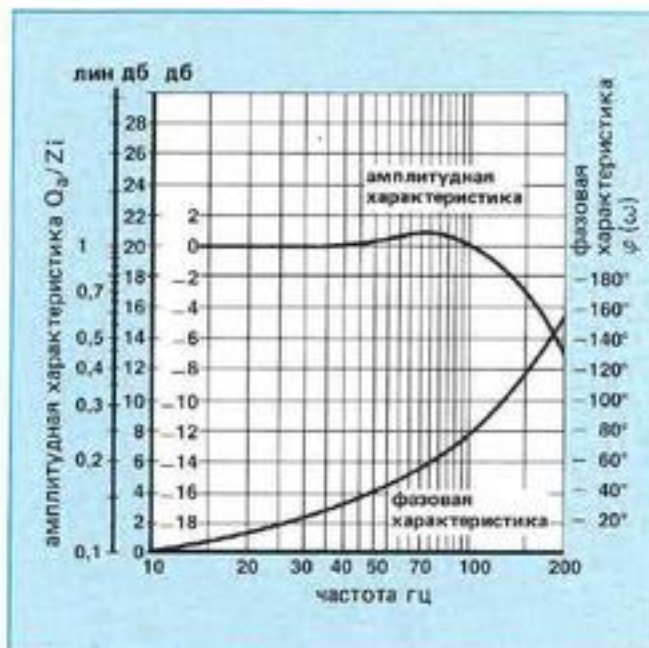
Рис. 13: Диаграмма Бode
