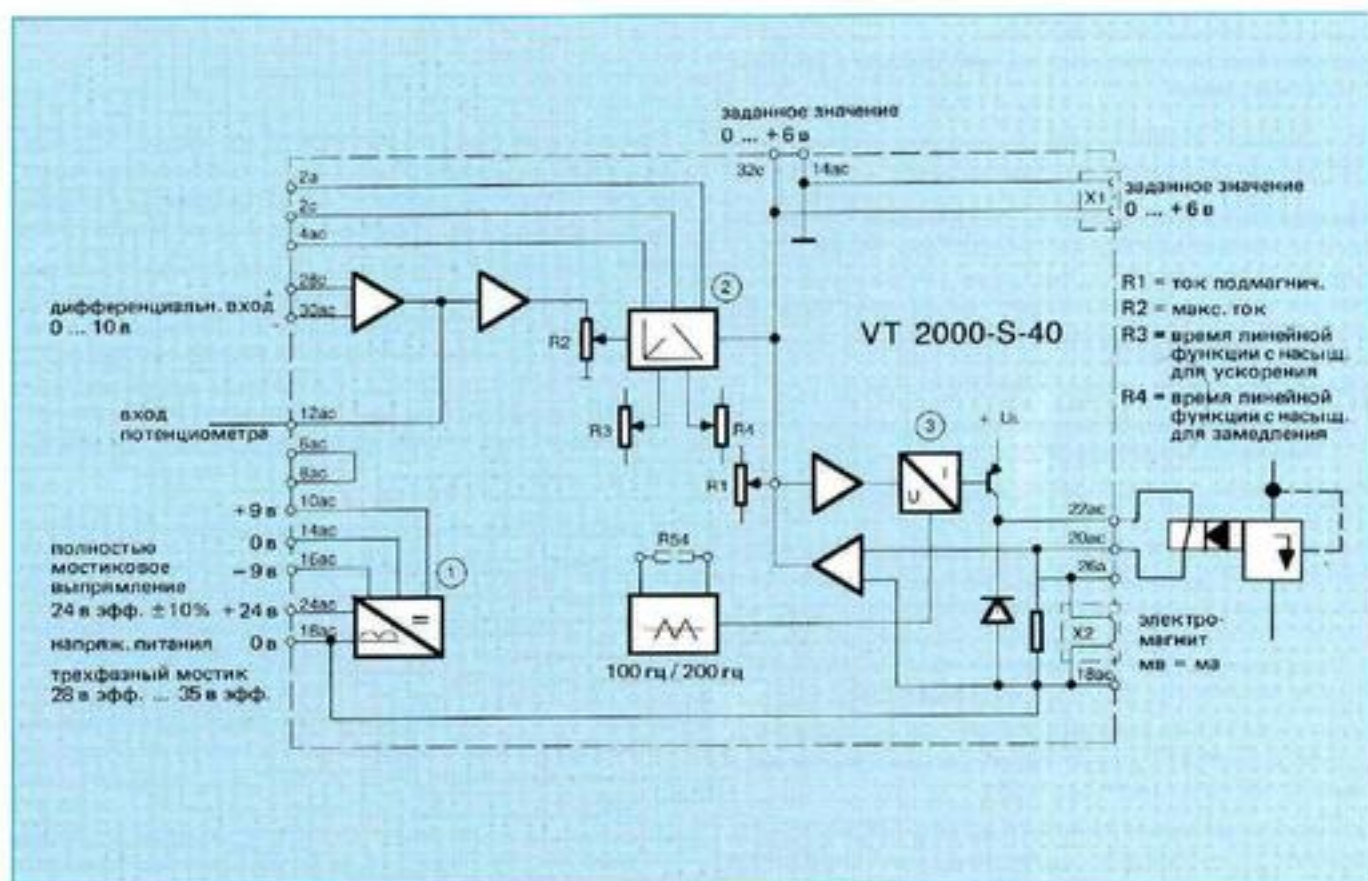
Рис. 17: Занятость присоединений пропорционального усилителя типа VT2000 S40
