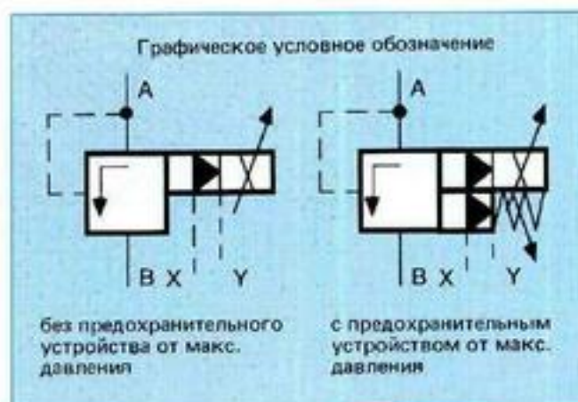
Рис. 44: Пропорциональный клапан для ограничения давления непрямого действия с предохранительным устройством от максимального давления типа DBEM
