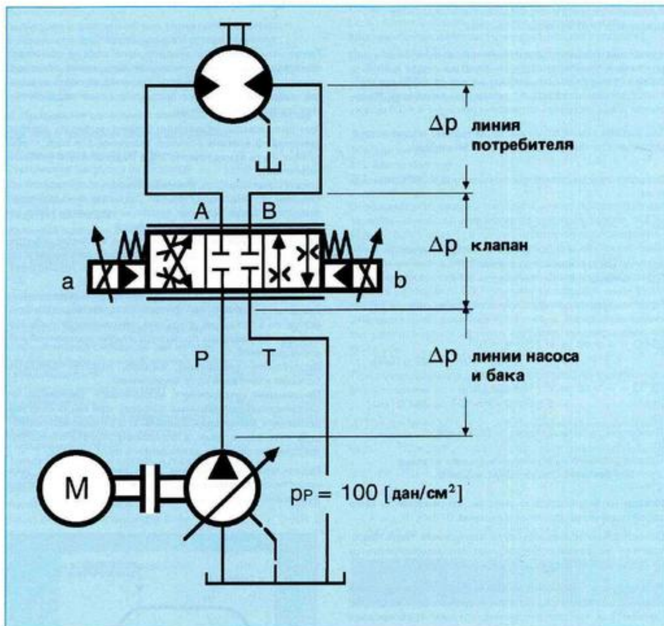
Рис. 21: Потеря давления в одной гидросистеме
