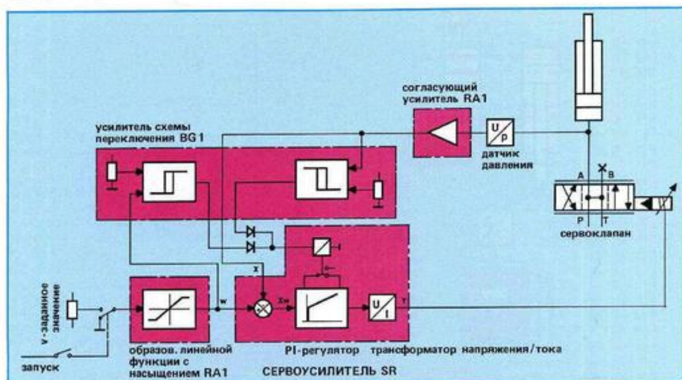
Рис. 57: Пример контура регулирования давления
