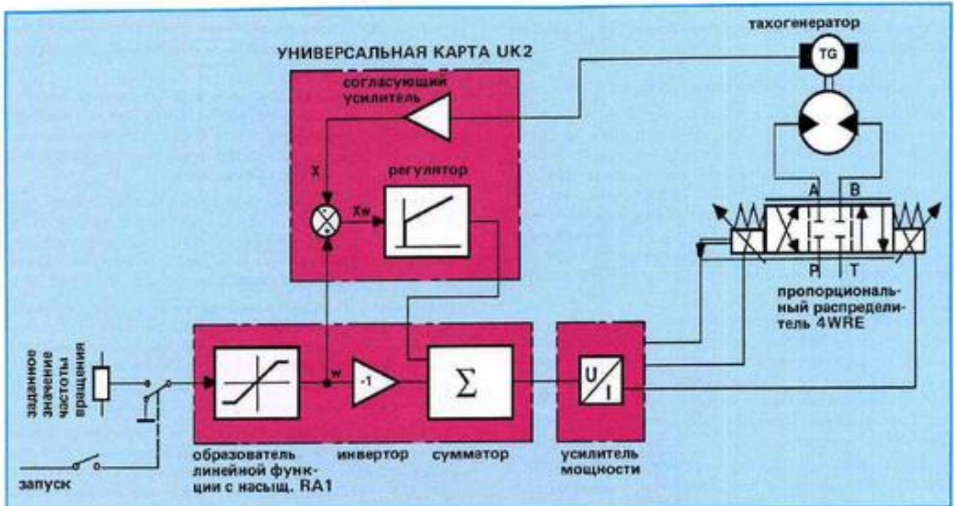
Рис. 54: Пример контура регулиров. частоты вращения
