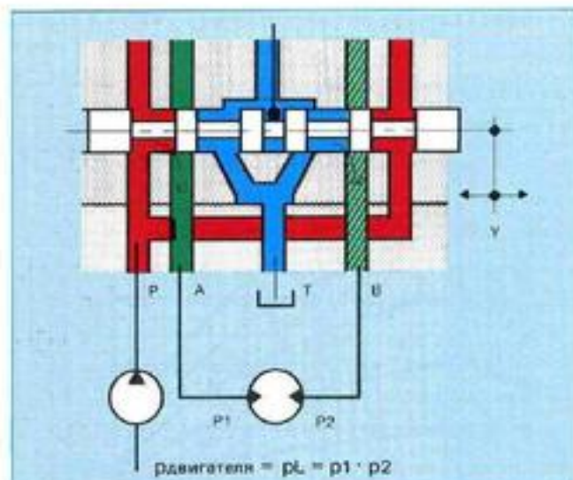
Рис. 10: Четырехкромочное дроссельное управление
