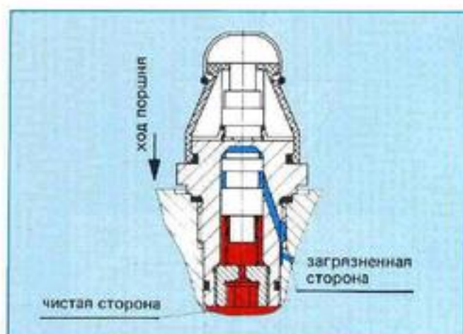
Рис. 23: Оптический индикатор загрязненности фильтра
