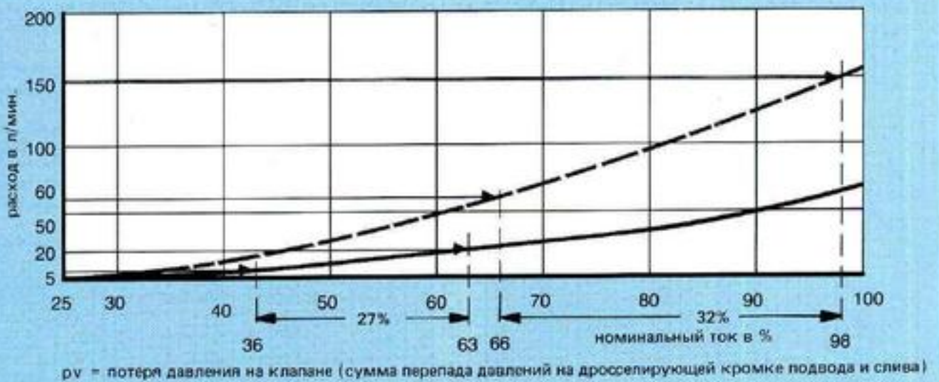
Рис. 14: Характеристика "расход-номинальный ток" для номинального расхода в 64 л/мин. при потери давления на клапане в 10 бар.
