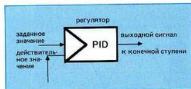
Рис. 10: PID-регулятор
