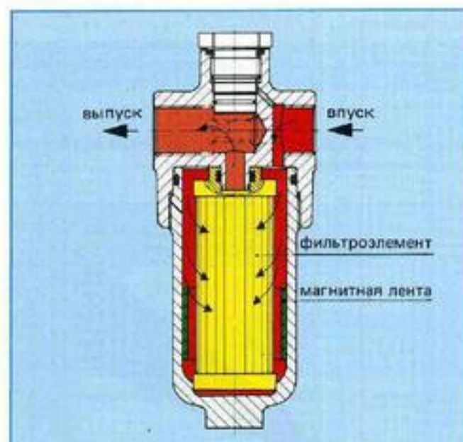
Рис. 19: Напорный фильтр в разрезе (монтаж в линии)
