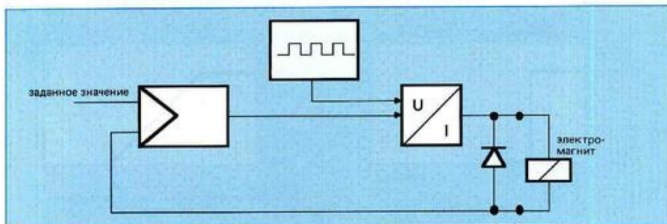
Рис. 4: Импульсно-модулированная конечная ступень
