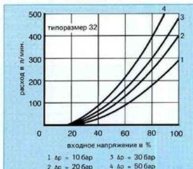
Рис. 58: Расходная характеристика, прогрессивная
