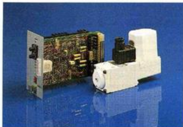
Рис. 26: Одноступенчатый регул. клапан типа 4WS 1EO6
