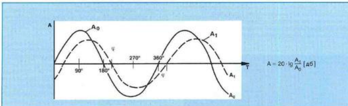
Рис. 15: Затухание амплитуды и смещение фазы
