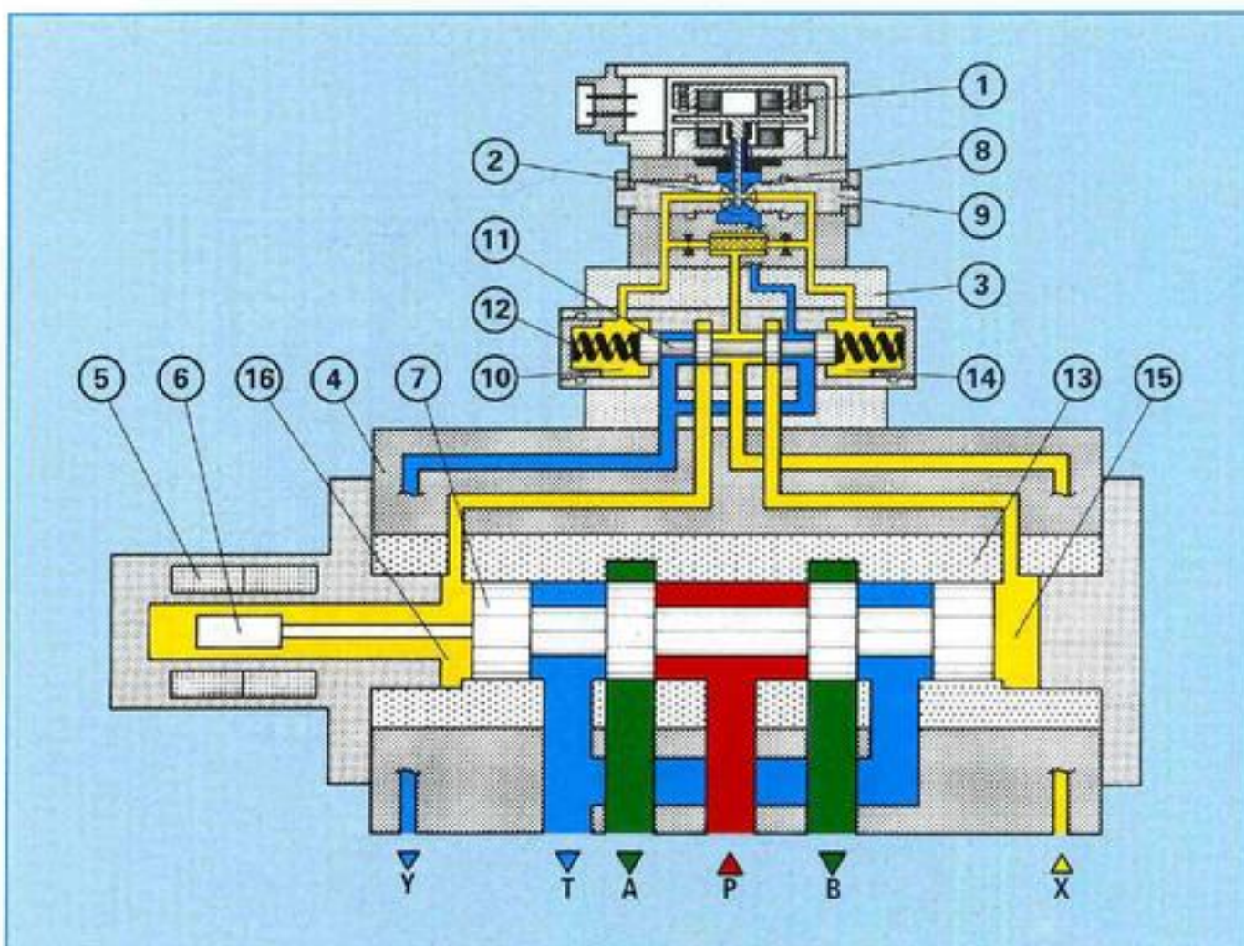
Рис. 24: Трехступенчатый сервораспределитель с электрической обратной связью типа 4WS3EE
