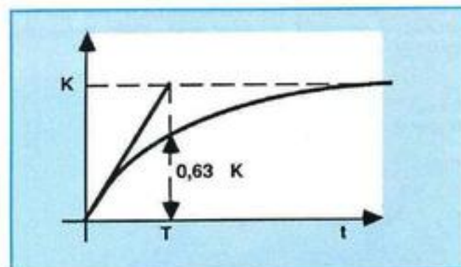
Рис. 27: Переходная характеристика P-T 1 -звена
