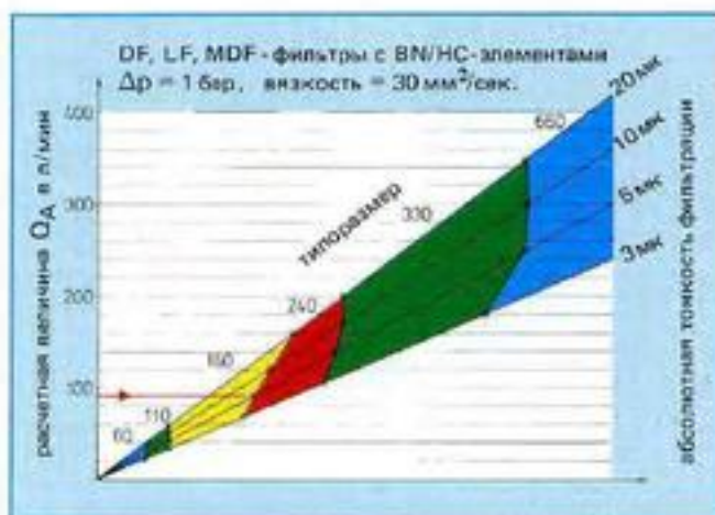
Рис. 16: Диаграмма для определения типоразмеров фильтра при напорных фильтрах
