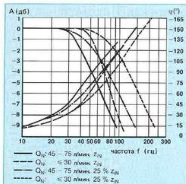
Рис. 14: Частотная характеристика сервоклапана ДУ10 с механической связью
