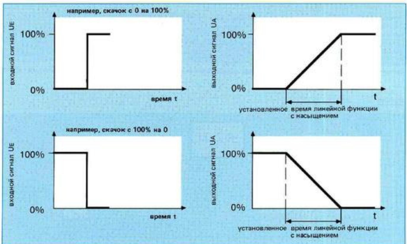
Рис. 2: Скачкообразный сигнал, время линейной функции с насыщением
