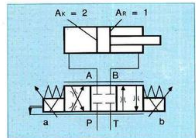
Рис. 21: Поршень E1 с дифференциальным цилиндром
