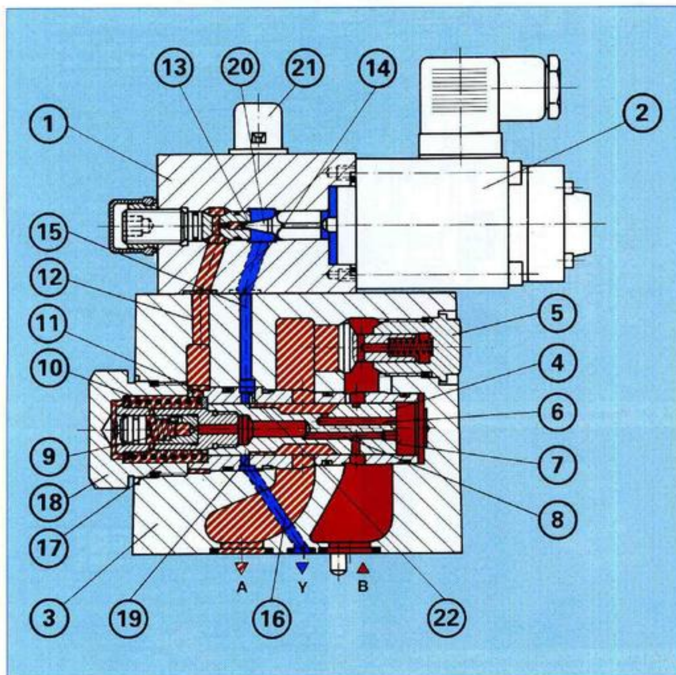
Рис. 45: Пропорциональный редукционный клапан непрямого действия типа DRE 10
