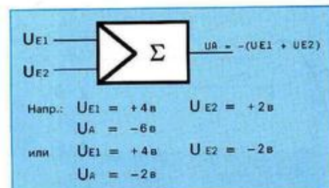
Рис. 11: Сумматор
