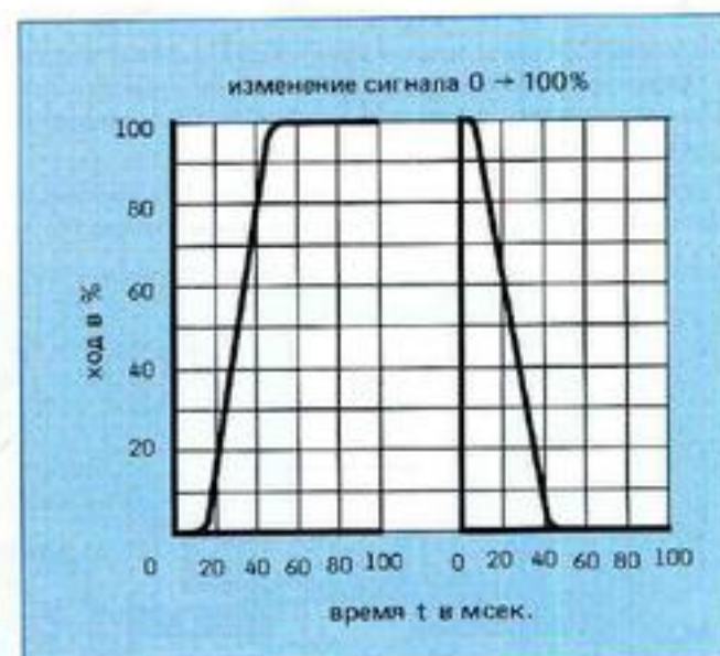
Рис. 32: Переходная функция при скачкообразном электрическом входном сигнале
