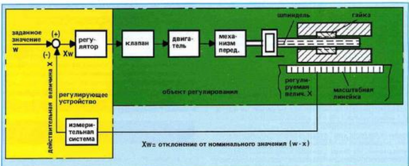
Рис. 12: Пример регулирования положения
