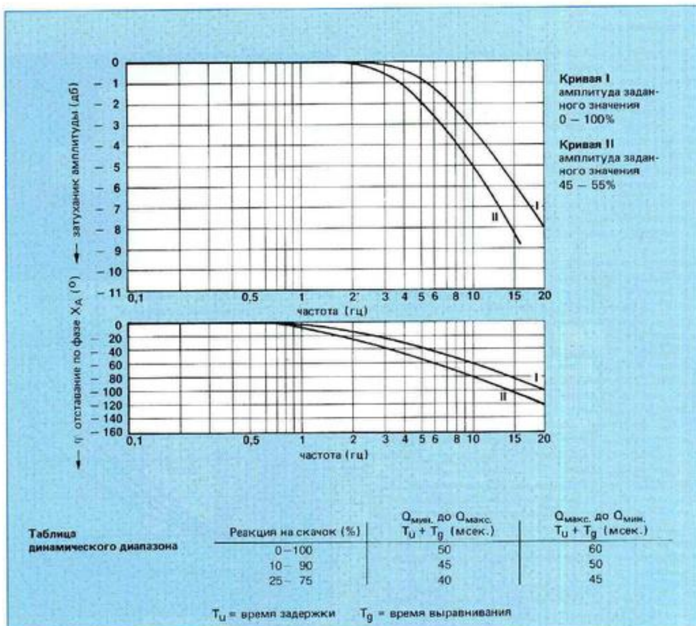
Рис. 55: Частотная характеристика
