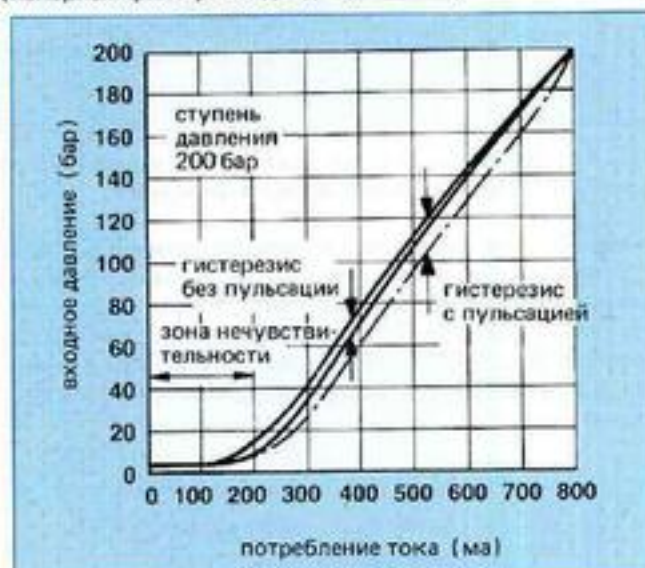
Рис. 42: Зависимость входного давления от потребления тока
