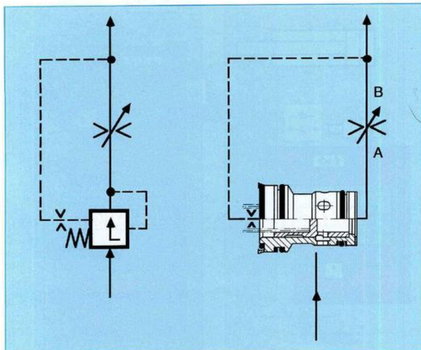
Рис. 22: Двухлинейный встроенный клапан для компенсации нагрузки
