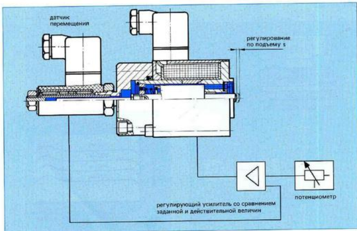
Рис. 4: Регулируемый электромагнит с регулированием по силе
