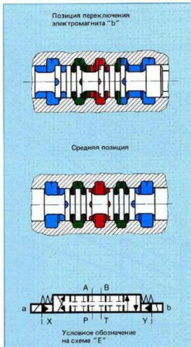
Рис. 11: Перекрывание переключающего распределителя ДУ25, условное обозначение на схеме "Е" (закрытая средняя позиция)
