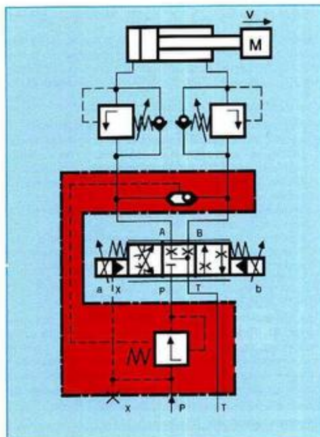
Рис. 12: Напорный клапан как подпора
