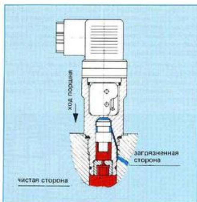
Рис. 22: Электр. индикатор загрязненности фильтра
