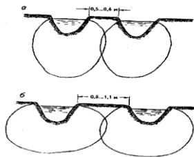
Рис. 4.15. Схемы контуров увлажнения почвы при поливе по бороздам: a – легкие почвы; b – тяжелые почвы
