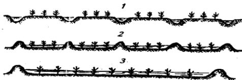
Рис. 4.14. Классификация поверхностных способов полива:
