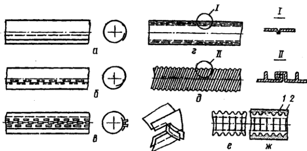
Рис. 3.7. Пластмассовые дренажные трубы: а – пленочные с упруго поджатым швом; б – пленочные со швом «молния»; в – пленочные со швом-перфорацией; г – пленочные гладко-стенные перфорированные; д – пленочные спиральновитые из профилированной ленты; е – гофрированные без защиты; ж – гофрированные, защищенные от заилиenia; 1 – салфетка; 2 – фильтрующий материал
