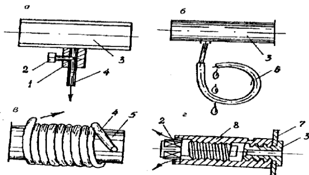
Рис. 4.20. Схема водовыпусков-капельниц:
