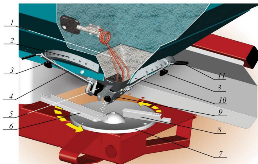
Рис. 8. Рассеивающий узел:
