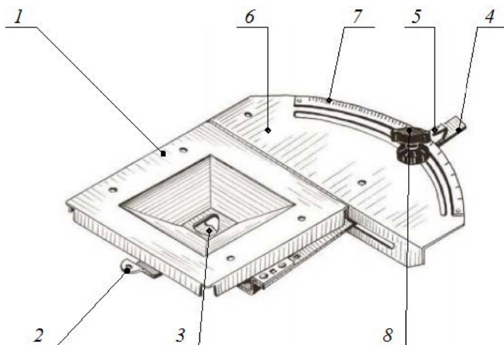
Рис. 5. Дозирующие механизмы: 1 – поддон; 2 – шибберная заслонка; 3 – дозирующая заслонка; 4 – рычаг дозирующей заслонки (дозатора); 5 – указатель дозатора; 6 – сектор; 7 – шкала дозатора; 8 – фиксатор
