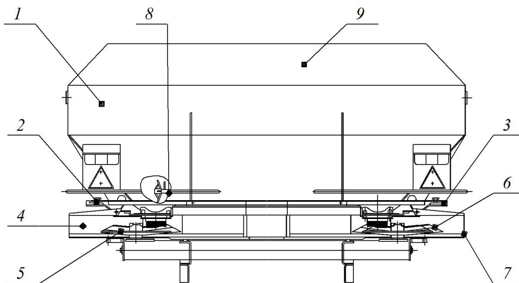
Рис. 2. Общий вид рассейвателя РУ-1600: 1 – бункер с рамой; 2 – механизм дозирующий правый; 3 – механизм дозирующий левый; 4 – отражатель правый; 5 – метатель (рассеивающий диск) правый; 6 – метатель (рассеивающий диск) левый; 7 – отражатель левый; 8 – рыхлитель (сводоразрушитель); 9 – тент
