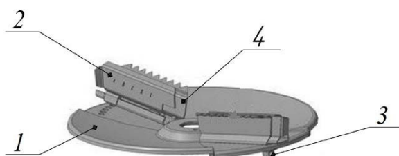
Рис. 4. Метатель (рассеивающий диск): 1 – диск; 2 – лопатка; 3 – фиксатор; 4 – направляющая
