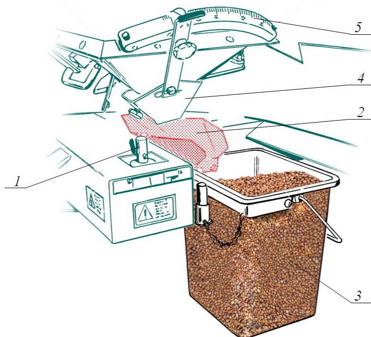
Рис. 9. Проверка нормы расхода при пробном проходе: 1 – вал диска; 2 – воронка; 3 – ведро; 4 – ссыпной лоток; 5 – шкала регулятора ширины захвата
