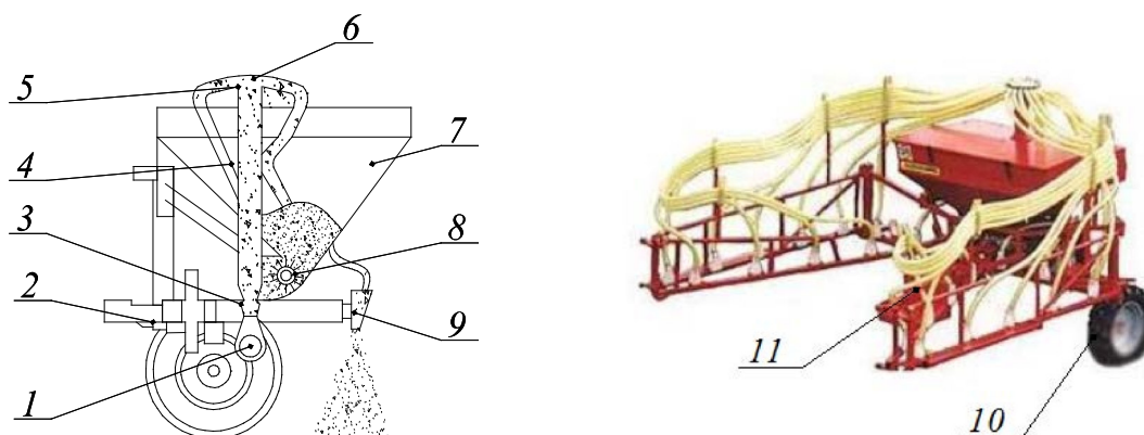
Рис. 13. Технологическая схема пневматической штанговой сеялки СУ-12: 1 – вентилятор; 2 – рама; 3 – эжектор; 4, 6 – пневмотукопроводы; 5 – распределительная головка; 7 – бункер; 8 – дозатор; 9 – распределители; 10 – колеса; 11 – штанга
