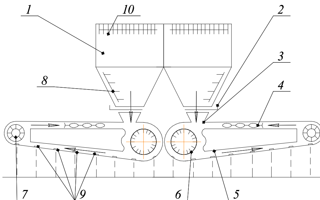
Рис. 14. Схема подкормщика РШУ-12: 1 – бункер; 2 – заслонка; 3 – приемный лоток; 4 – цепь с шайбами; 5 – распределительная штанга; 6 – ведущий шкив; 7 – ведомый шкив; 8 – воршитель; 9 – высевные отверстия; 10 – сетка
