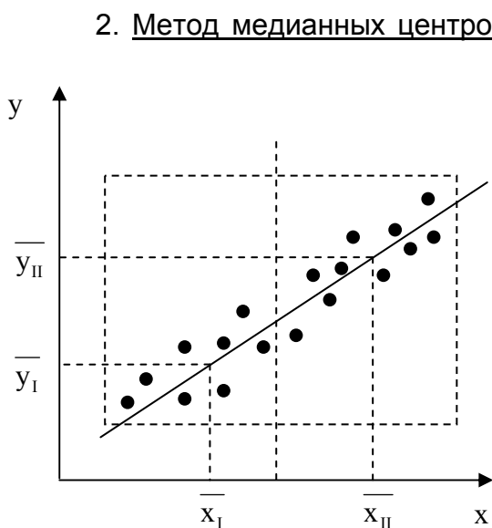
Рис.4.5. Метод медианных точек
