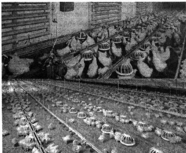
Рис. 9.13. Напольное содержание родительского стада бройлеров фирмы Big Dutchman с чашечной системой кормления
