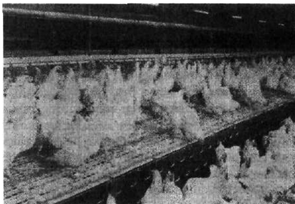
Рис. 9.20. Система напольного содержания кур с использованием решетчатого пола фирмы Big Dutchman
