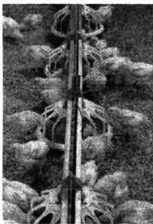
Рис. 9.11. Чашечная система кормления с высокорасположенным кормораздаточным каналом
