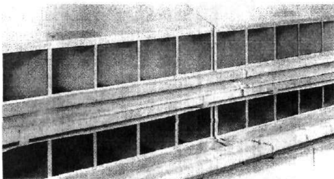
Рис. 9.15. Групповое гнездо «Колони» - двухэтажное полуавтоматическое Х-12
