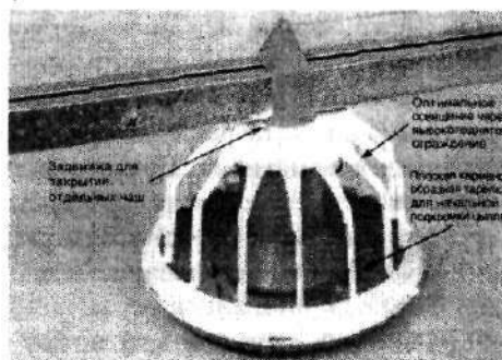
Рис. 9.10. Кормовая чаша для выращивания ремонтного молодняка (фирма Big Dutchman)
