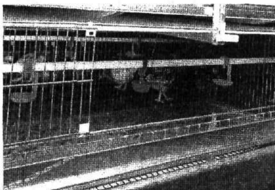
Рис. 9.3. Ярус для цыплят UV-S 630 с открытой круглой поилкой для упрощения поиска воды в первые дни
