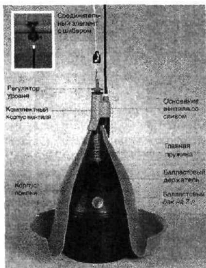
Рис. 9.26. Основные элементы устройства круговой поилки ЮМБО-Т фирмы Big Dutchman
