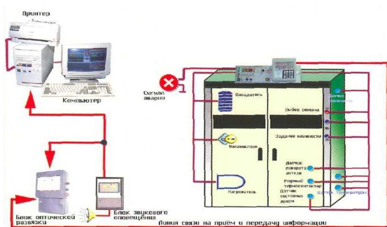
Рис. 48. Система управления инкубатором
