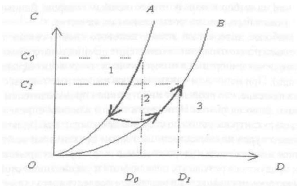
Рисунок 6.1 – Механизм импортозамещения
