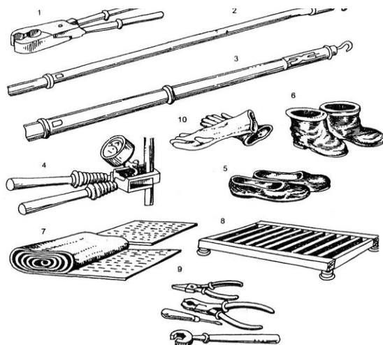
Рис. 3. Защитные средства, применяемые для работы в электроустановках:
