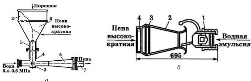
Рис. 6. Пеногенераторы:
