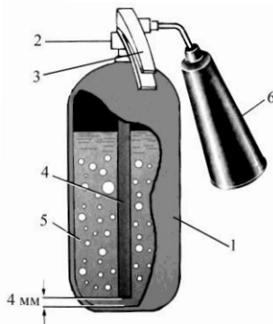
Рис. 5. Углекислотный огнетушитель:
