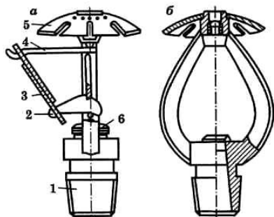
Рис. 7. Оросители водяные: а – спринклер; б – дренажер: 1 – насадок; 2, 4 – рычаги; 3 – легкоплавкий замок; 5 – розетка; 6 – клапан
